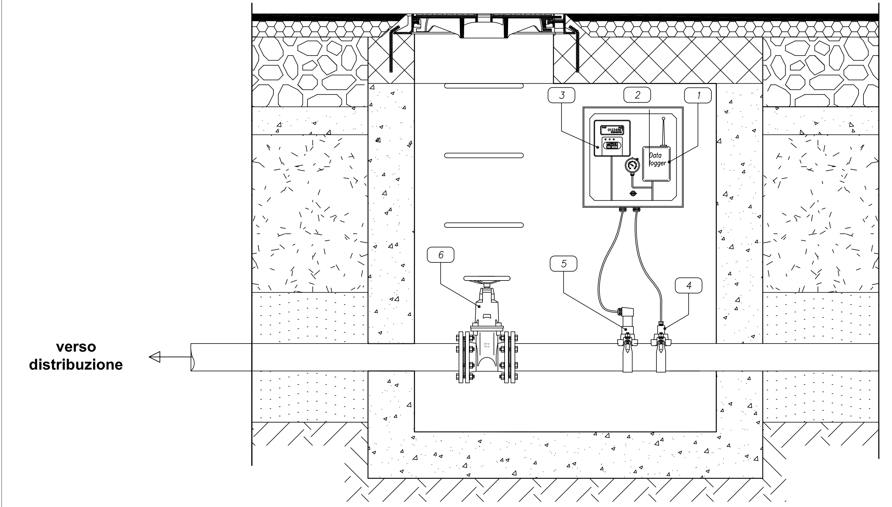
Pozzetto di distrettualizzazione
