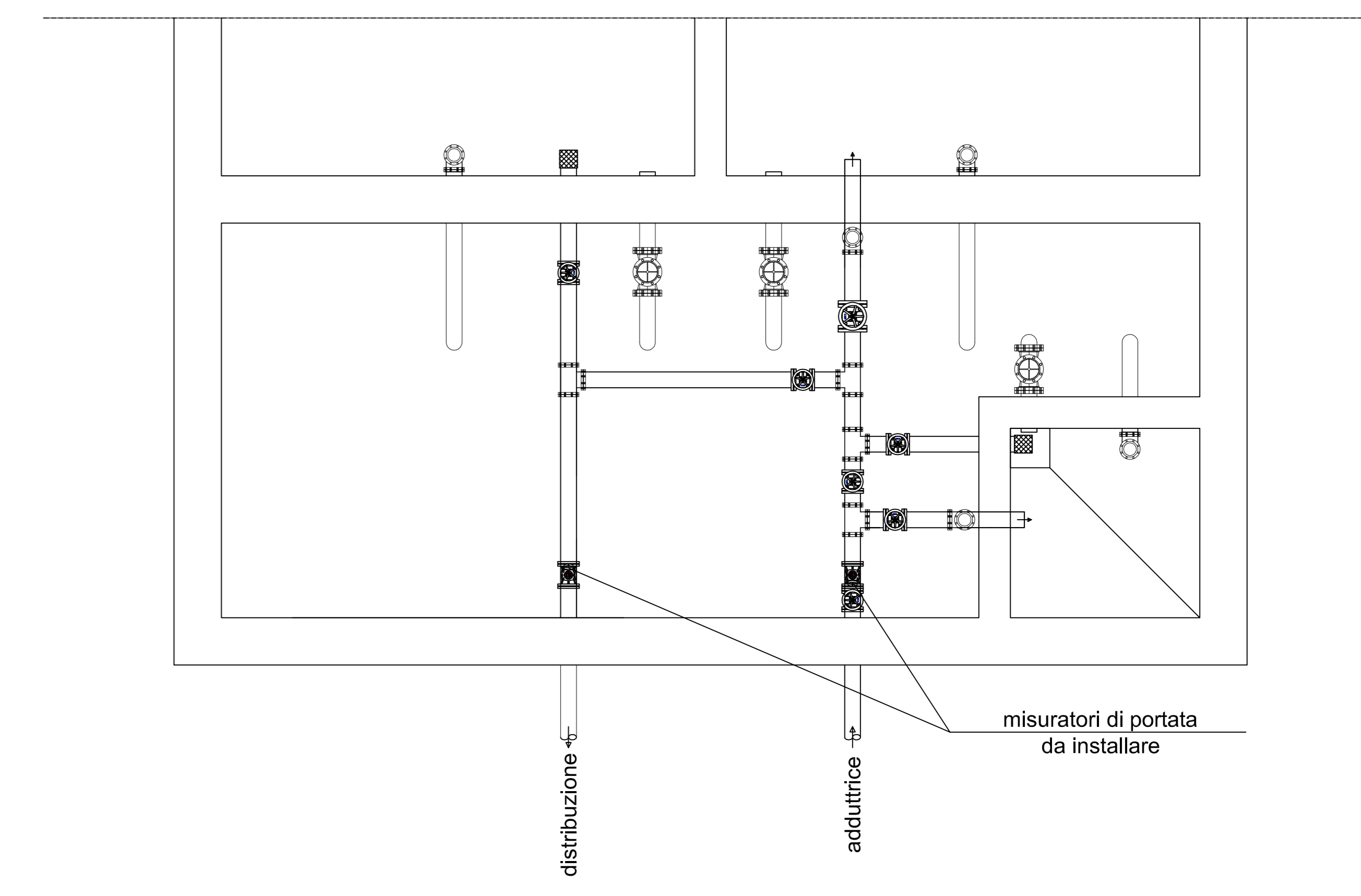
Serbatoio a due vasche rettangolari
