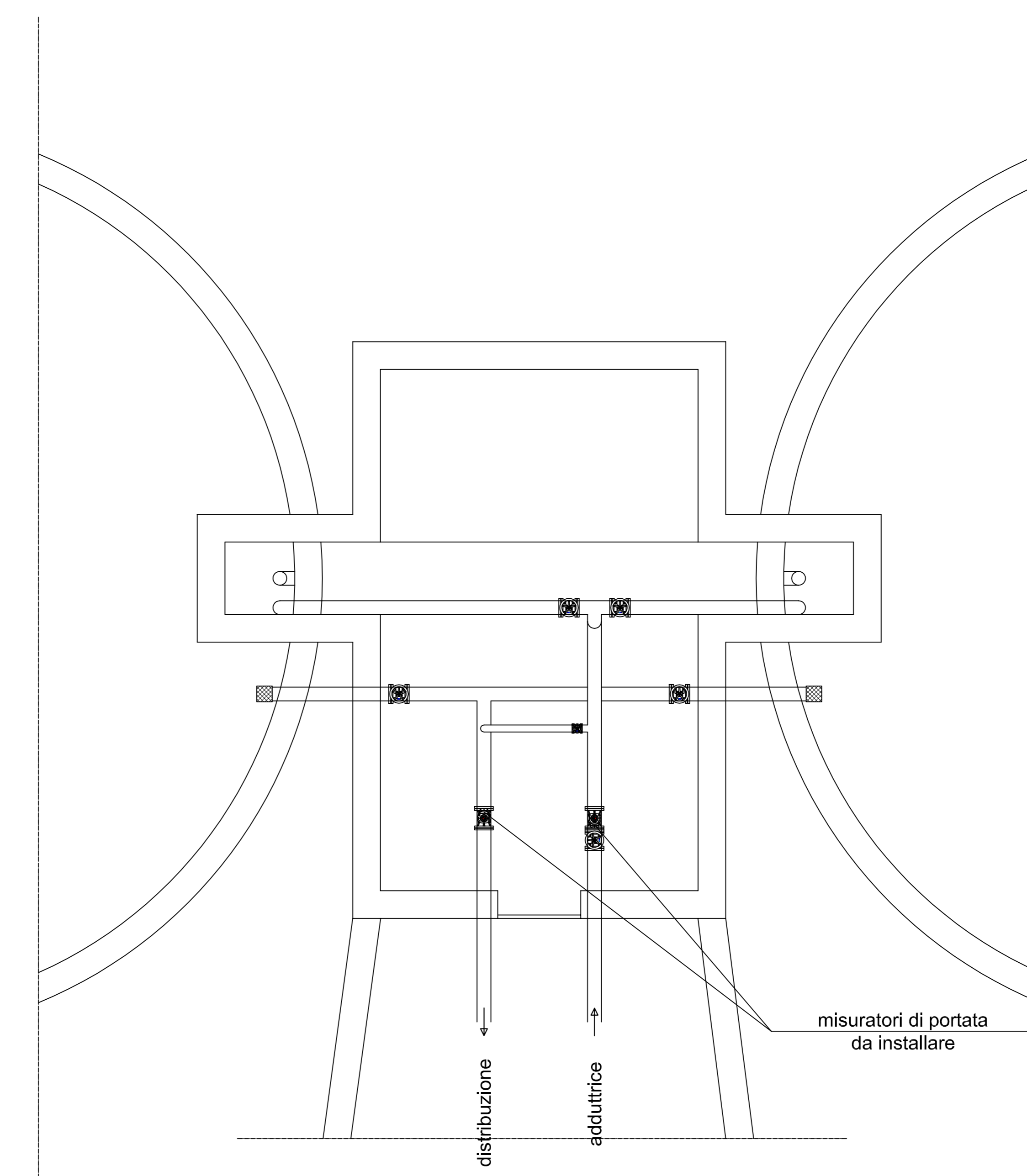
Serbatoio a due vasche circolari
