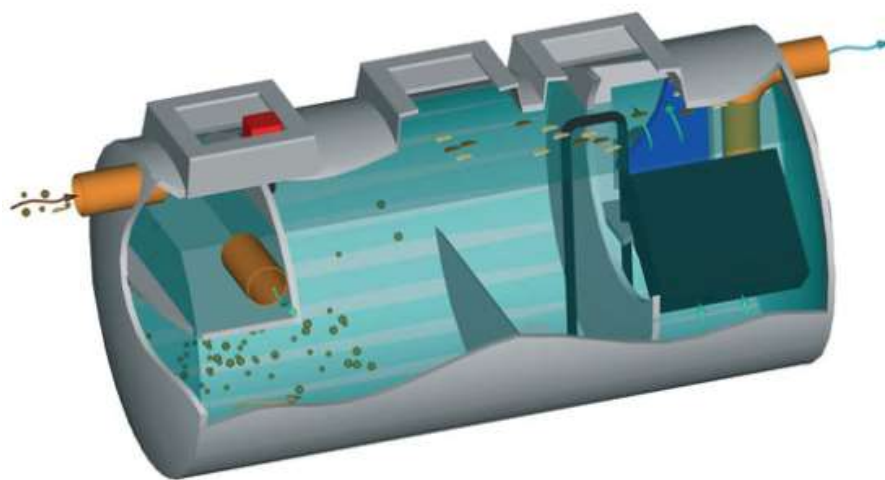
Figura 20: Spaccato tipico dell'impianto monoblocco di trattamento delle acque di prima pioggia
