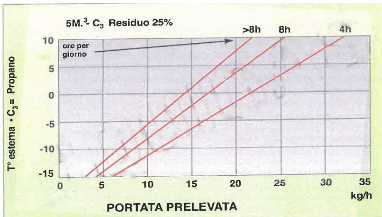
Figura 17: Grafico portata estratta dal serbatoio in funzione della temperatura
