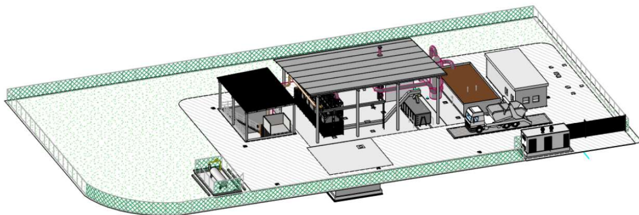
Figura 12: Vista 3D dell'ingresso impianto con indicazione della zona pesatura e dell'ufficio accettazione
