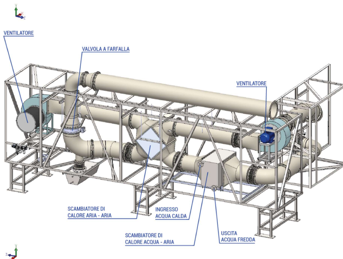
Figura 9: Rappresentazione 3D di un modulo BioDryer™, relativamente alla parte scambiatore di calore
