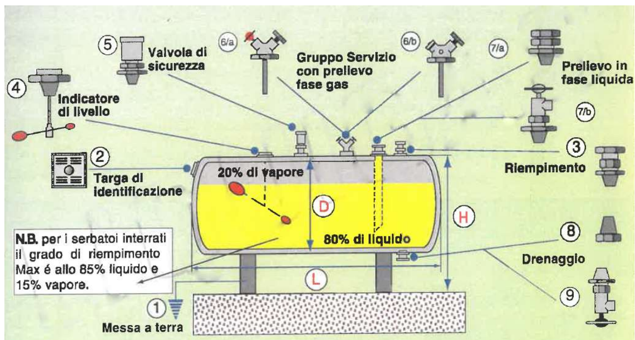
Figura 18: Schema tipico di un serbatoio GPL orizzontale con accessori
