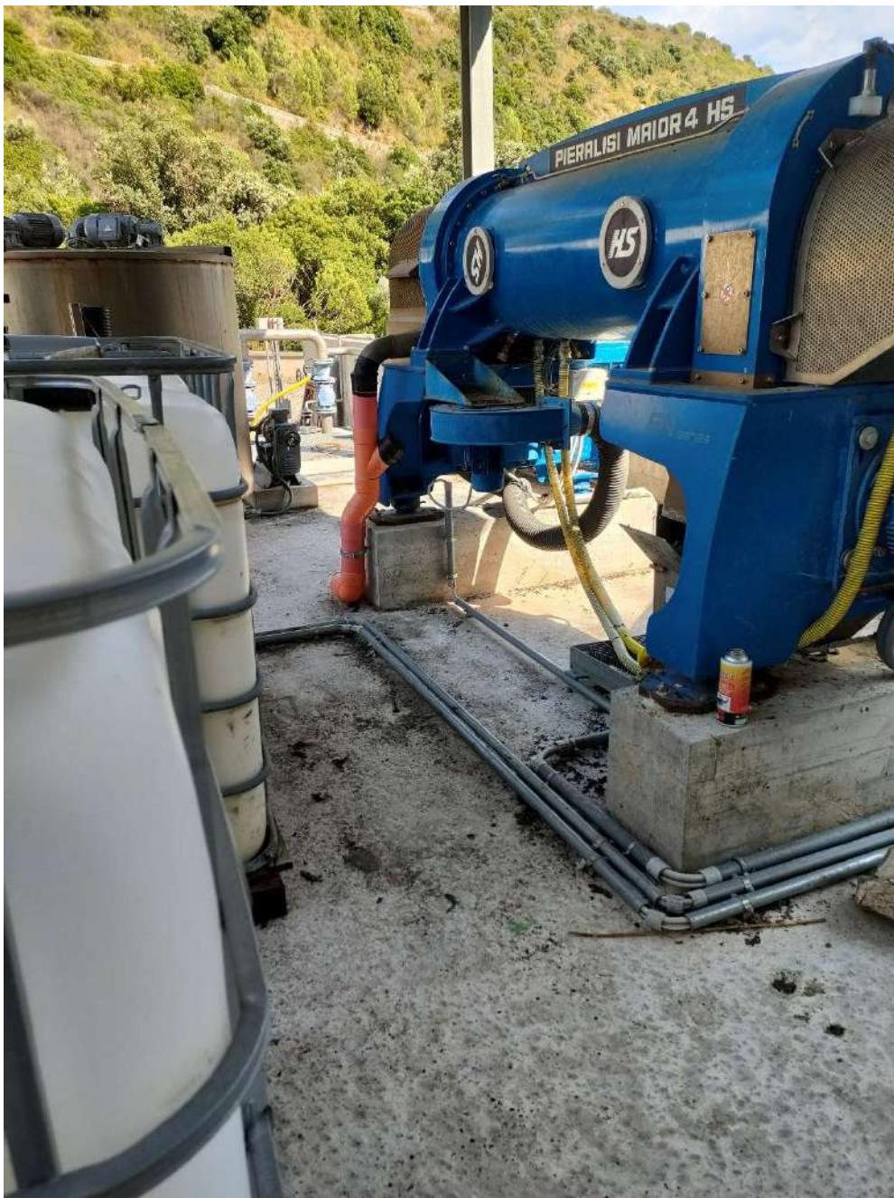
Figura 29: 2 – Centrifuga per disidratazione fanghi
