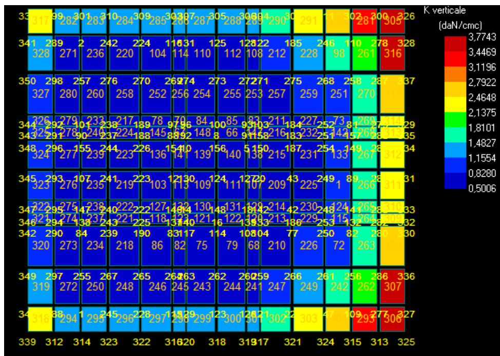
Figura 7: Costante di Winkler – stratigrafia 1.
