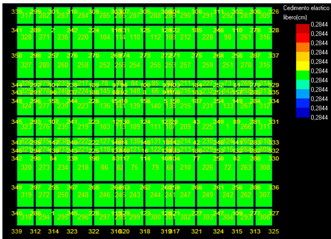
Figura 16: Cedimento - Stratigrafia 2.
