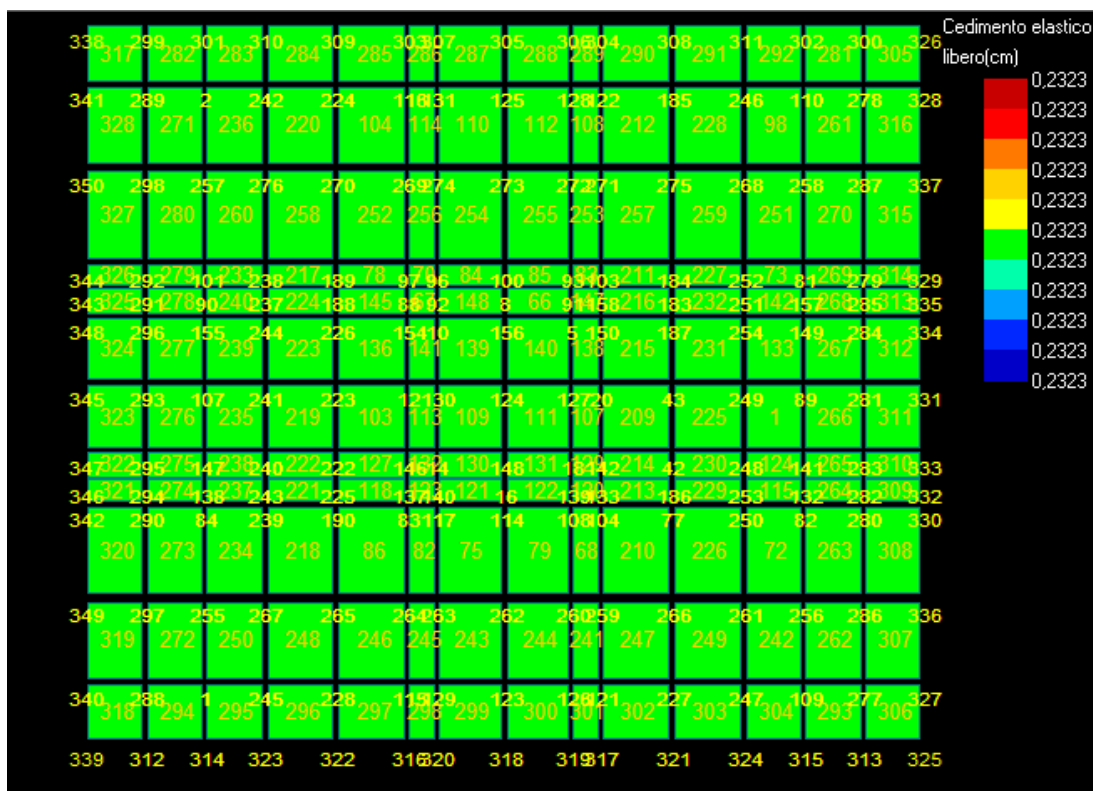
Figura 15: Cedimento - Stratigrafia 1.
