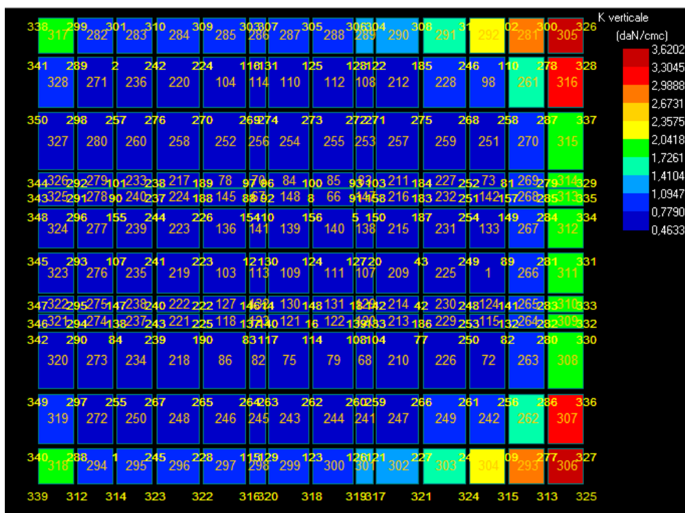
Figura 8: Costante di Winkler – stratigrafia 2.
