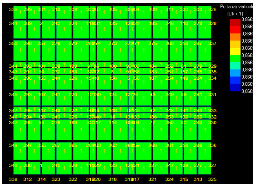
Figura 12: Portata – carico limite - Stratigrafia 2.
