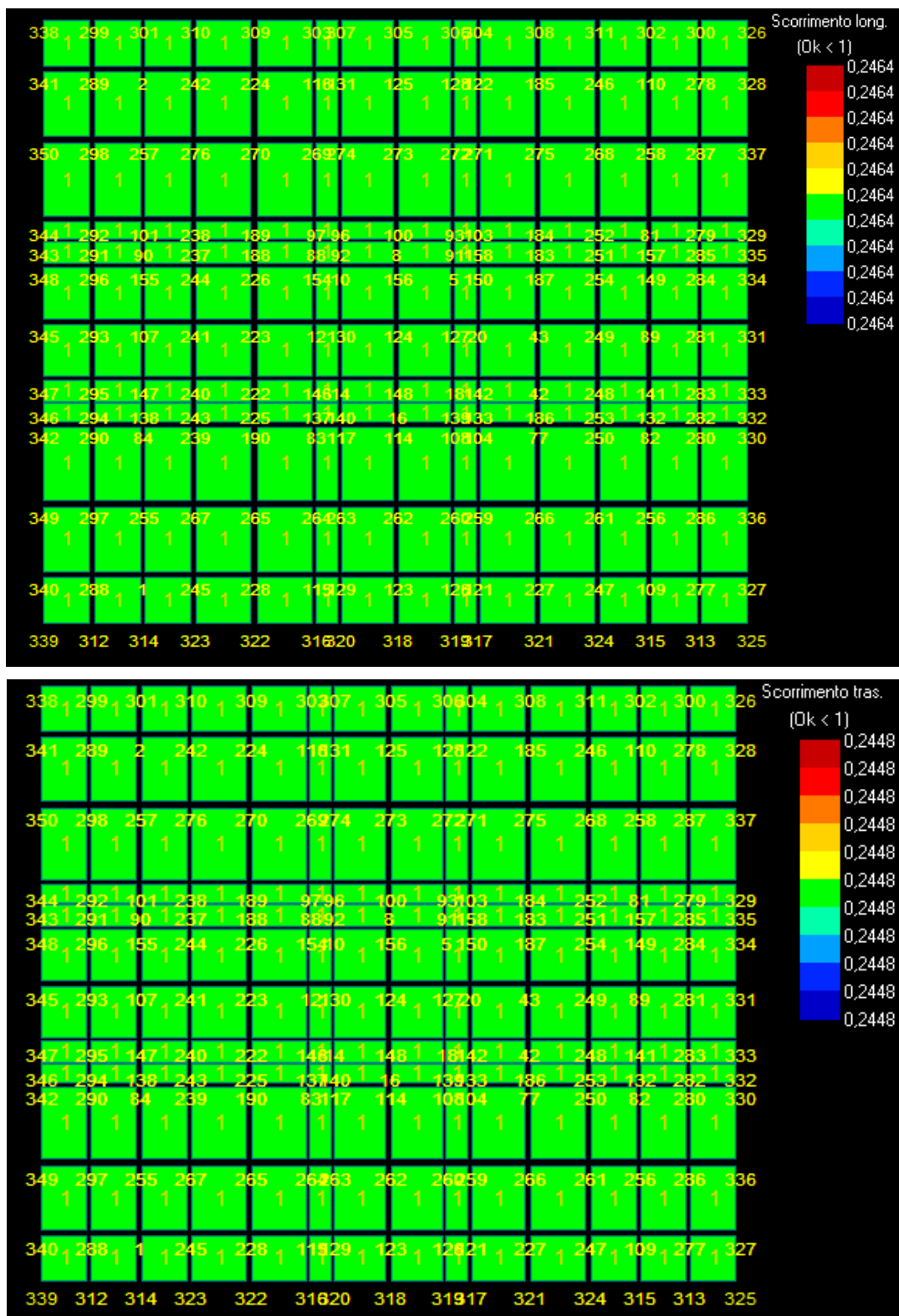
Figura 14: Scorrimento - Stratigrafia 2.
