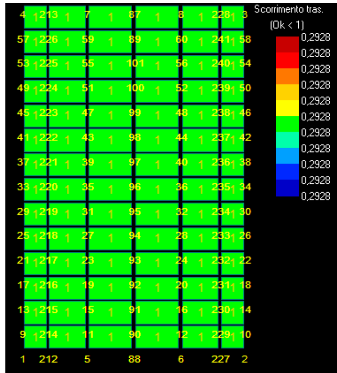
Figura 13: Scorrimento - Stratigrafia 1.
