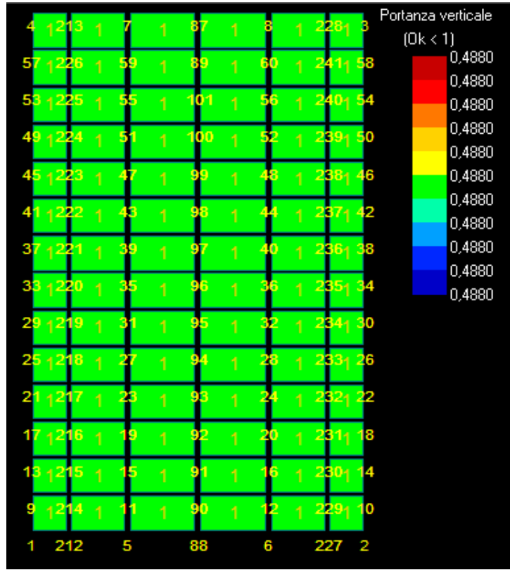
Figura 12: Portata – carico limite - Stratigrafia 2.
