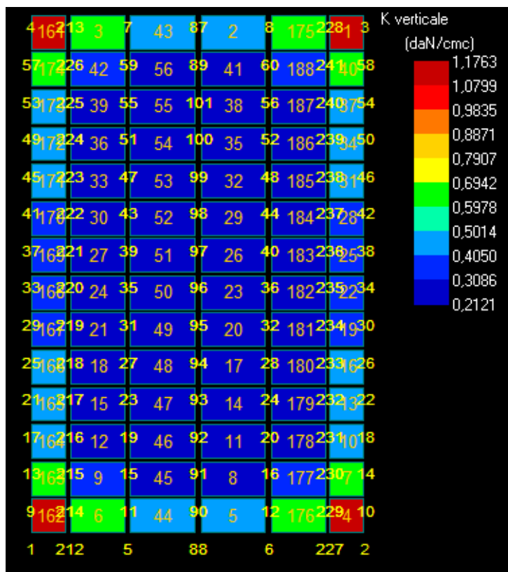
Figura 7: Costante di Winkler – stratigrafia 1.
