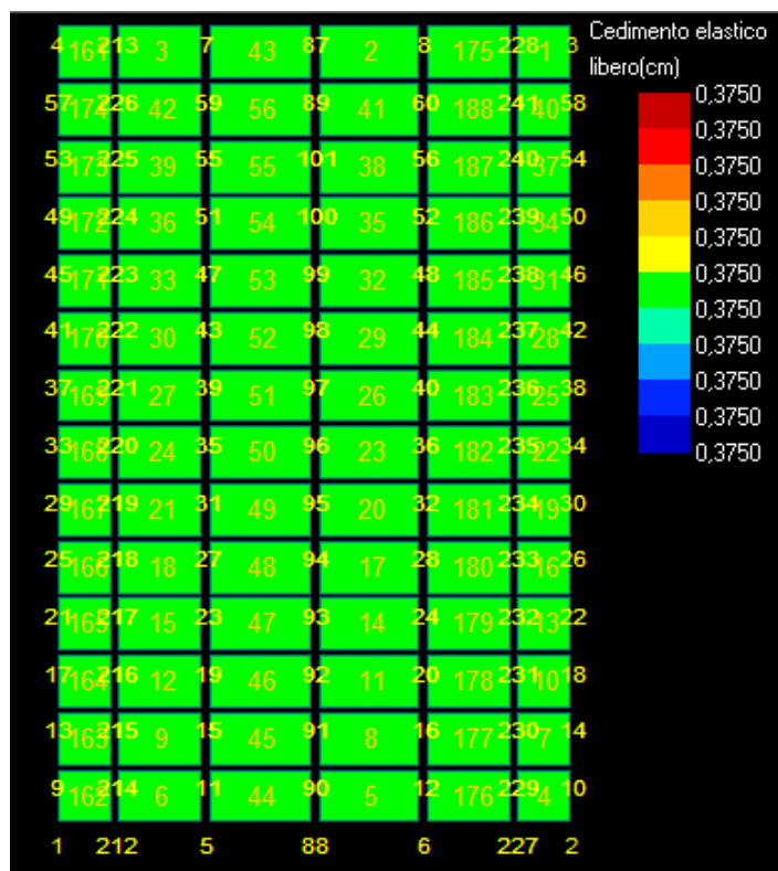
Figura 15: Cedimento - Stratigrafia 1.
