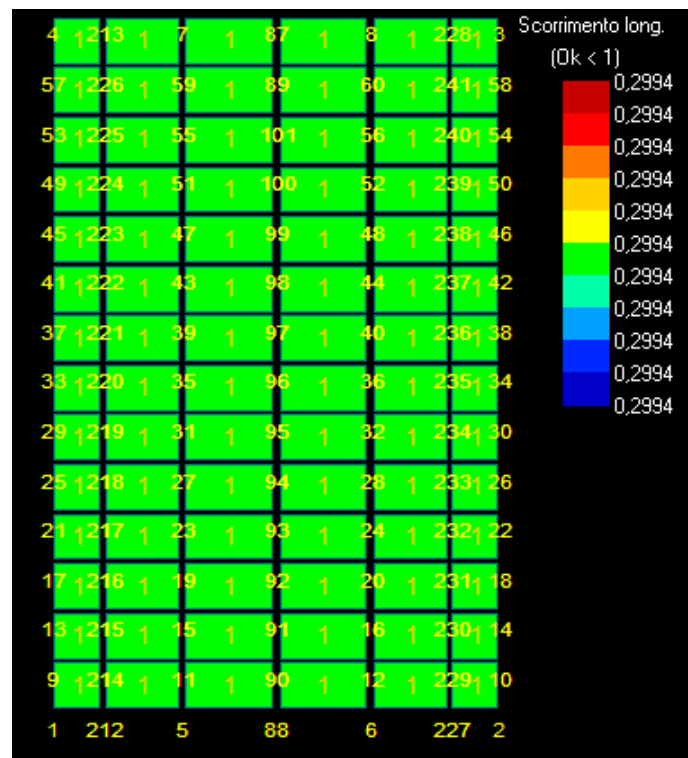
Figura 13: Scorrimento - Stratigrafia 1.
