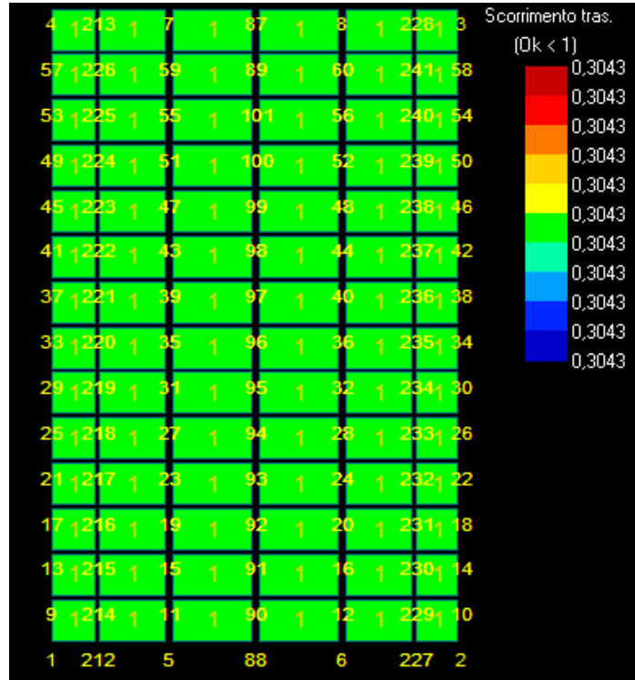
Figura 14: Scorrimento - Stratigrafia 2.
