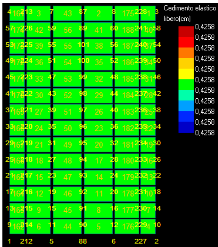
Figura 16: Cedimento - Stratigrafia 2.
