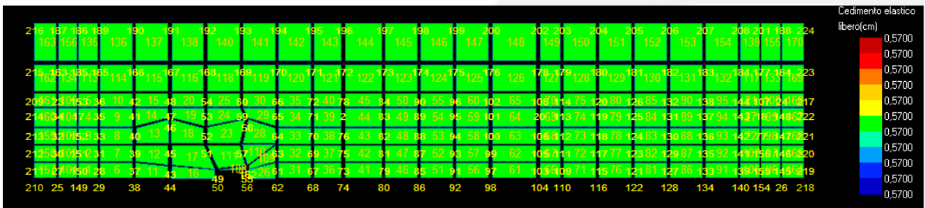
Figura 16: Cedimento - Stratigrafia 2.
