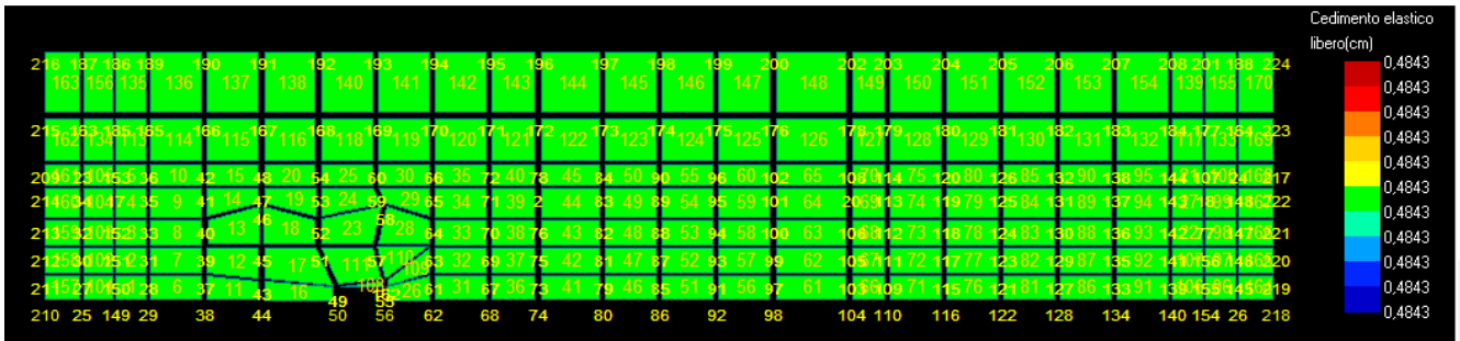
Figura 15: Cedimento - Stratigrafia 1.
