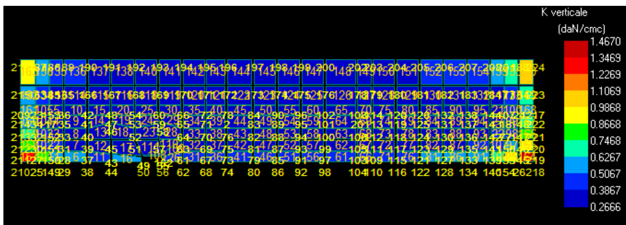
Figura 7: Costante di Winkler – stratigrafia 1.
