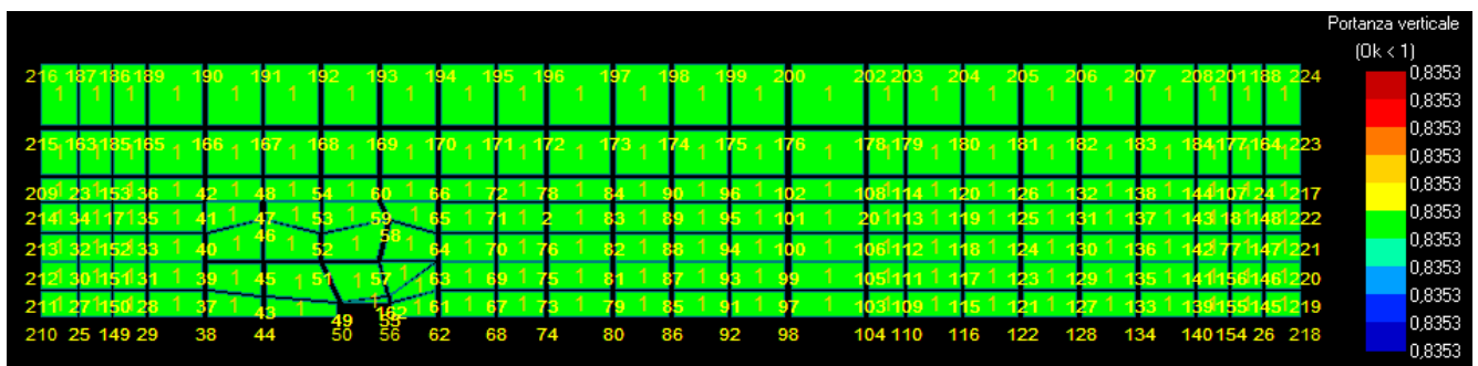
Figura 11: Portata – carico limite - Stratigrafia 1.
