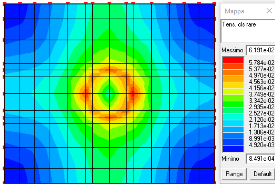
Figura 24: Verifica tensioni rare nel cls.
