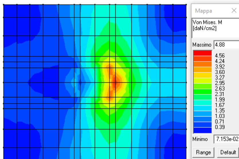
Figura 18: Tensioni di flessione (M) tramite formulazione di Von Mises.
