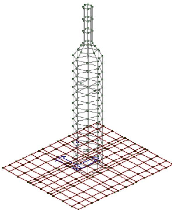
Figura 16: Vista complessiva del modello di calcolo
