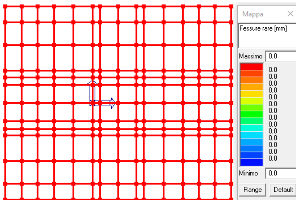
Figura 23: Fessure nel cls.
