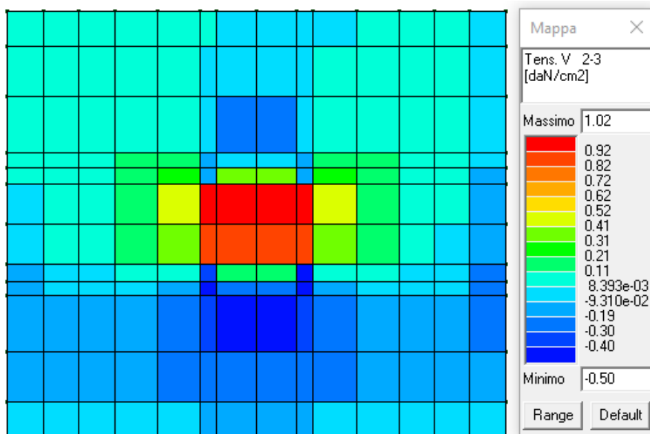
Figura 20: Tensioni di taglio 2-3 in daN/cm 2 .
