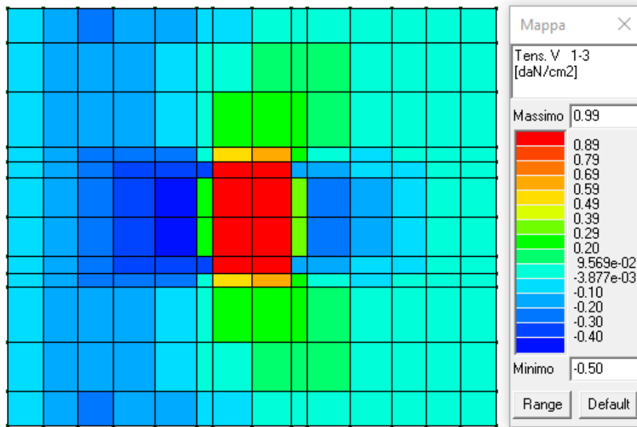
Figura 19: Tensioni di taglio 1-3 in daN/cm 2 .
