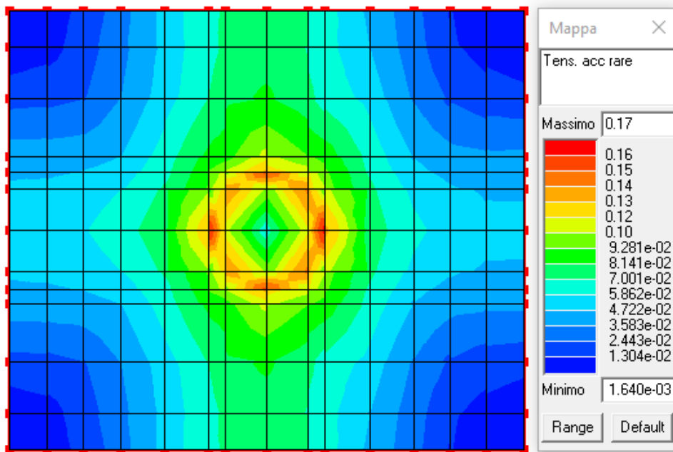
Figura 25: Verifica tensioni rare nell'acciaio.
