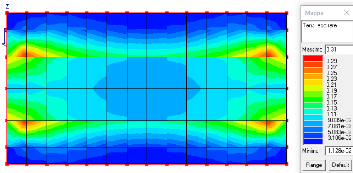
Figura 24: Verifica tensioni rare nell'acciaio.
