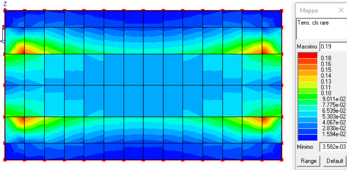
Figura 23: Verifica tensioni rare nel cls.
