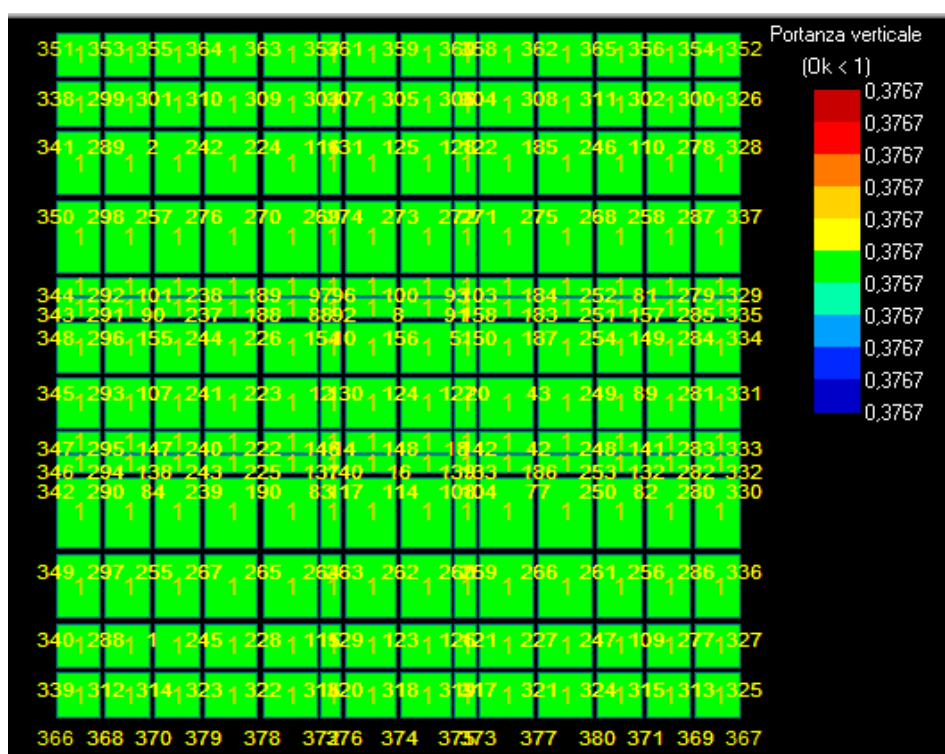
Figura 11: Portata – carico limite - Stratigrafia 1.
