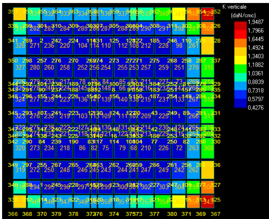
Figura 7: Costante di Winkler – stratigrafia 1.
