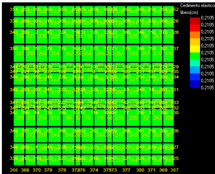
Figura 15: Cedimento - Stratigrafia 1.
