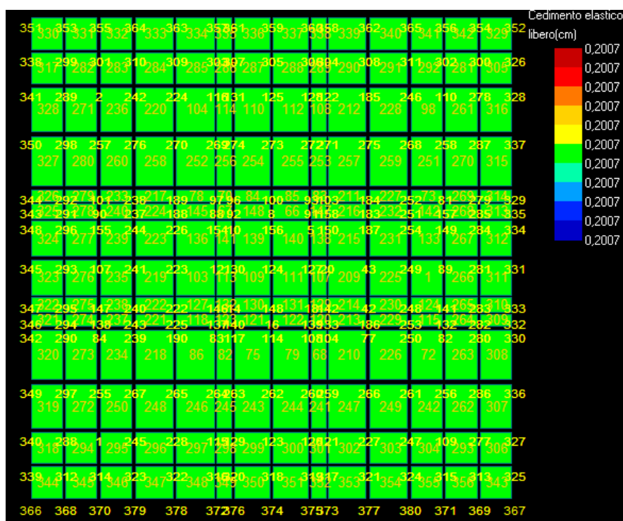
Figura 16: Cedimento - Stratigrafia 2.
