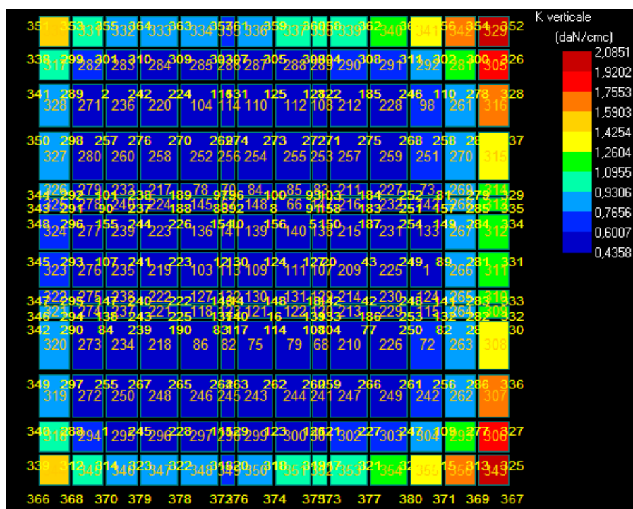
Figura 8: Costante di Winkler – stratigrafia 2.
