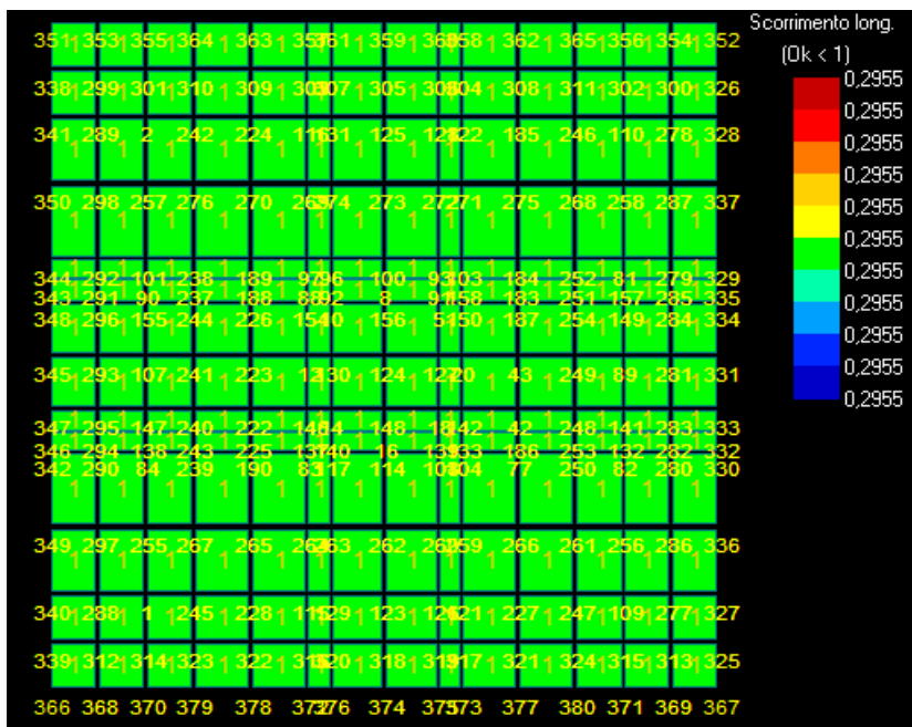
Figura 13: Scorrimento - Stratigrafia 1.
