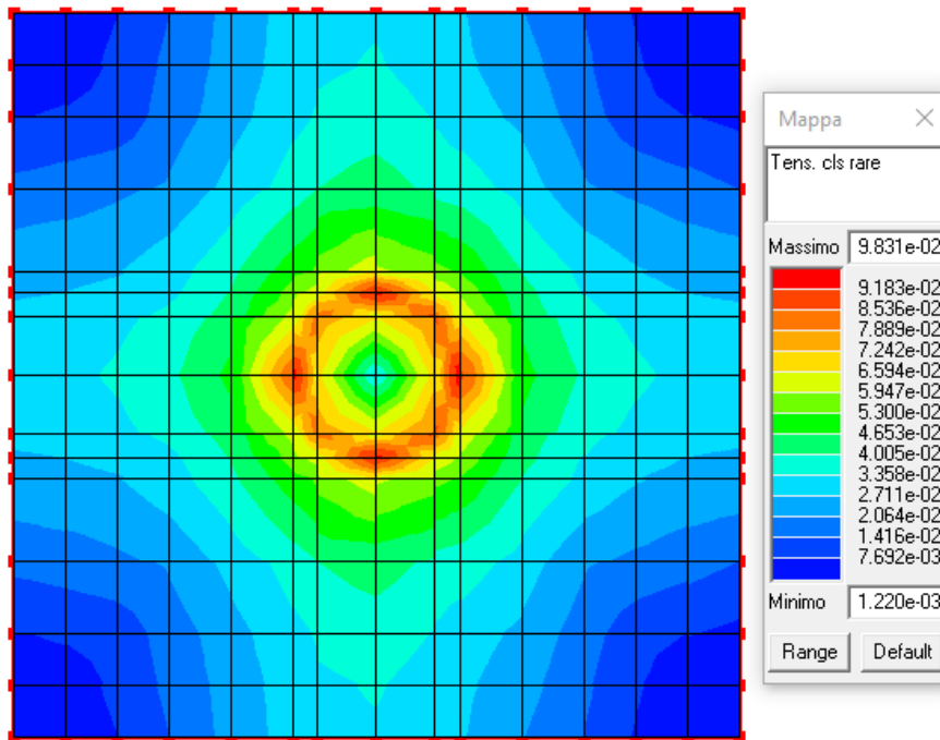
Figura 24: Verifica tensioni rare nel cls.
