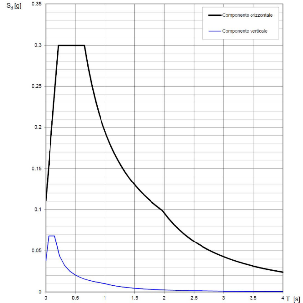
Figura 14: Parametri spettro di risposta SLV.
