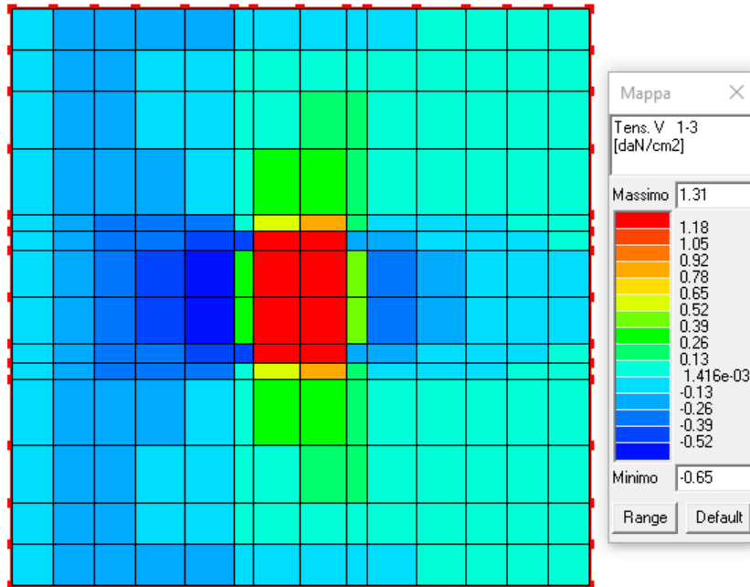
Figura 19: Tensioni di taglio 1-3 in daN/cm 2 .
