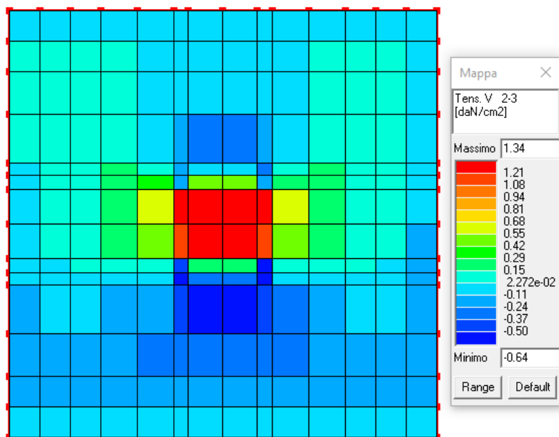
Figura 20: Tensioni di taglio 2-3 in daN/cm 2 .
