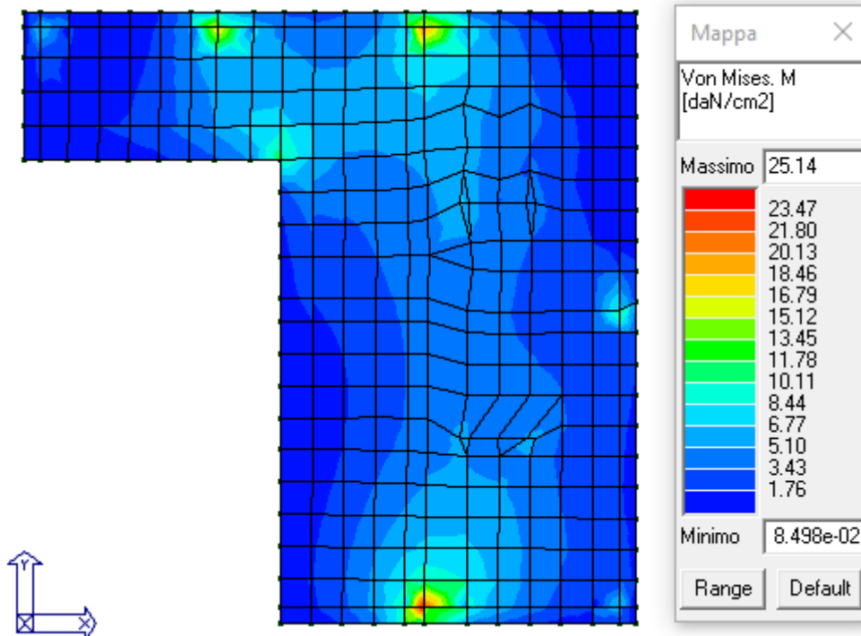
Figura 19: Tensioni di flessione (M) tramite formulazione di Von Mises.
