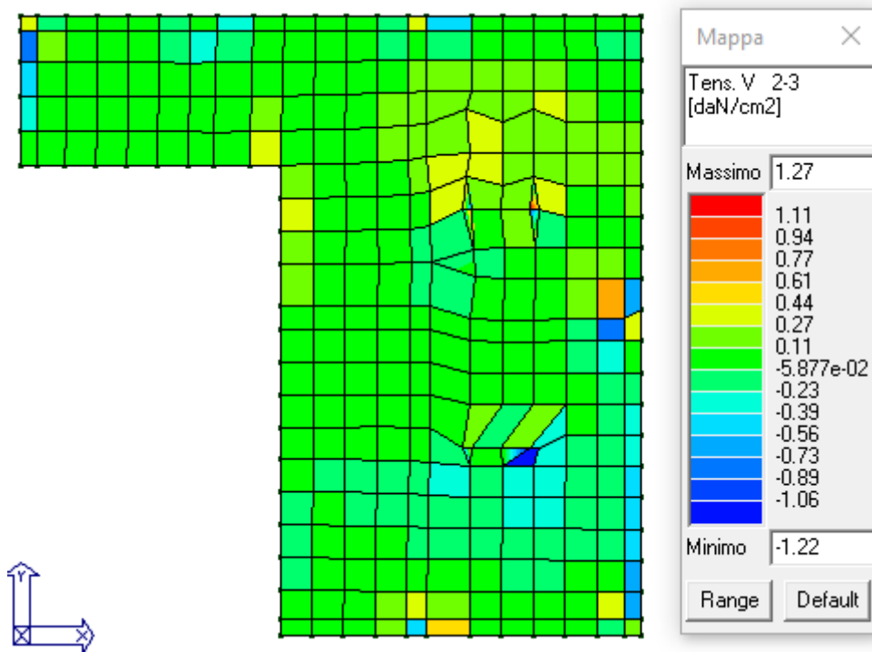
Figura 21: Tensioni di taglio 2-3 in daN/cm 2 .
