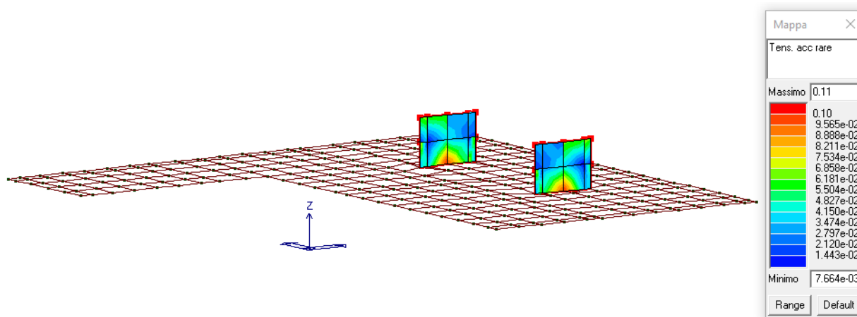
Figura 35: Verifica tensioni rare nell'acciaio.
