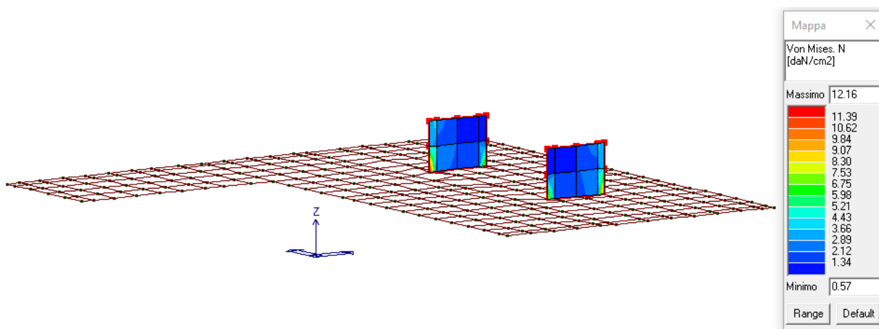
Figura 27: Tensioni di membrana (N) tramite formulazione di Von Mises.
