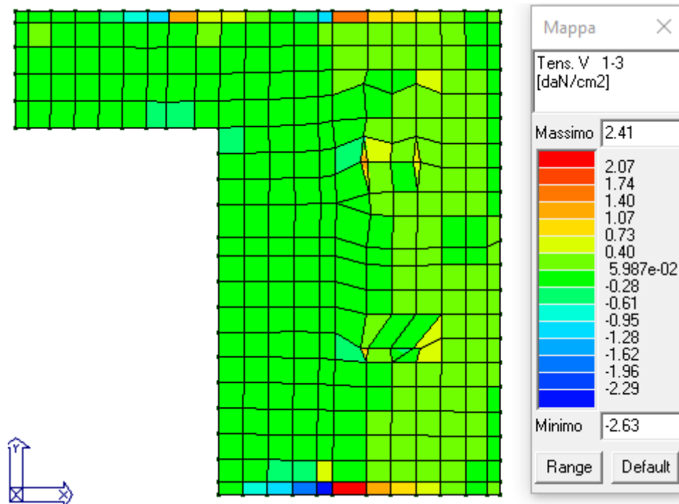
Figura 20: Tensioni di taglio 1-3 in daN/cm 2 .
