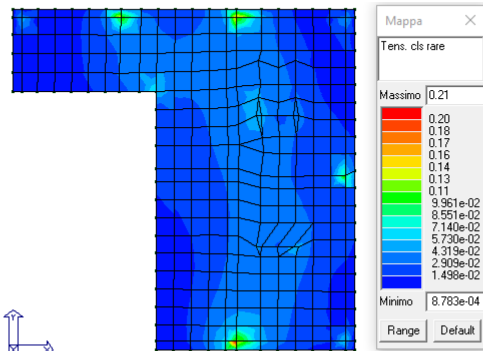
Figura 25: Verifica tensioni rare nel cls.
