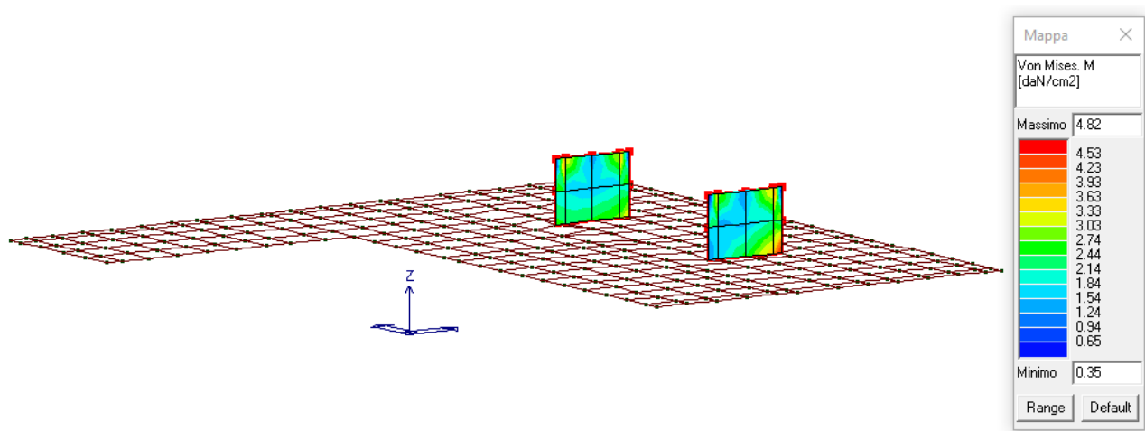
Figura 28: Tensioni di flessione (M) tramite formulazione di Von Mises.
