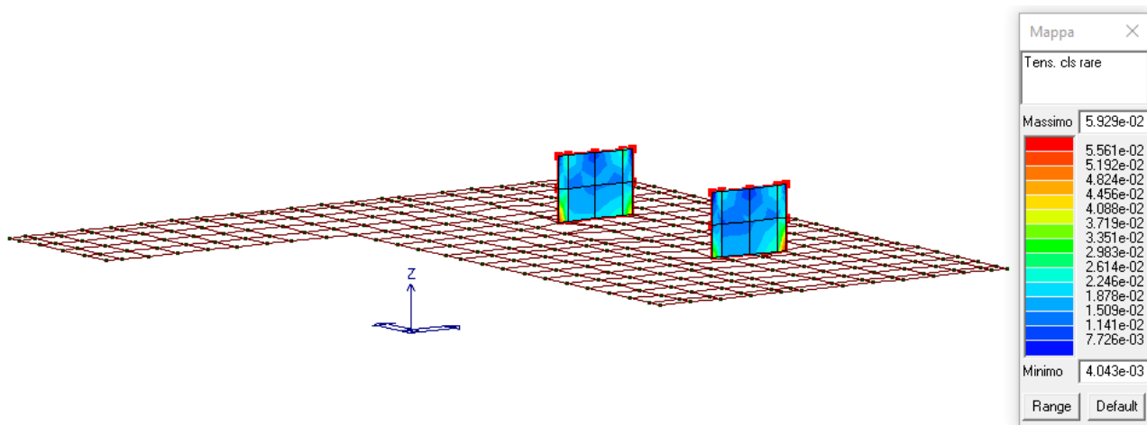
Figura 34: Verifica tensioni rare nel cls.
