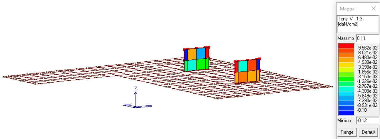
Figura 29: Tensioni di taglio 1-3 in daN/cm 2 .
