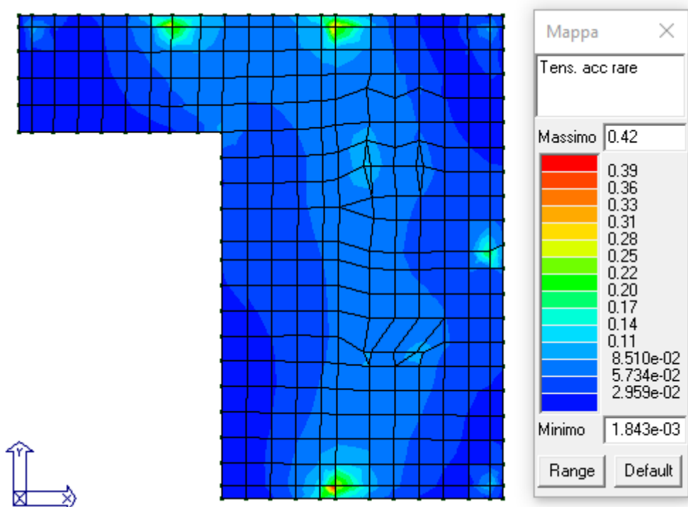
Figura 26: Verifica tensioni rare nell'acciaio.
