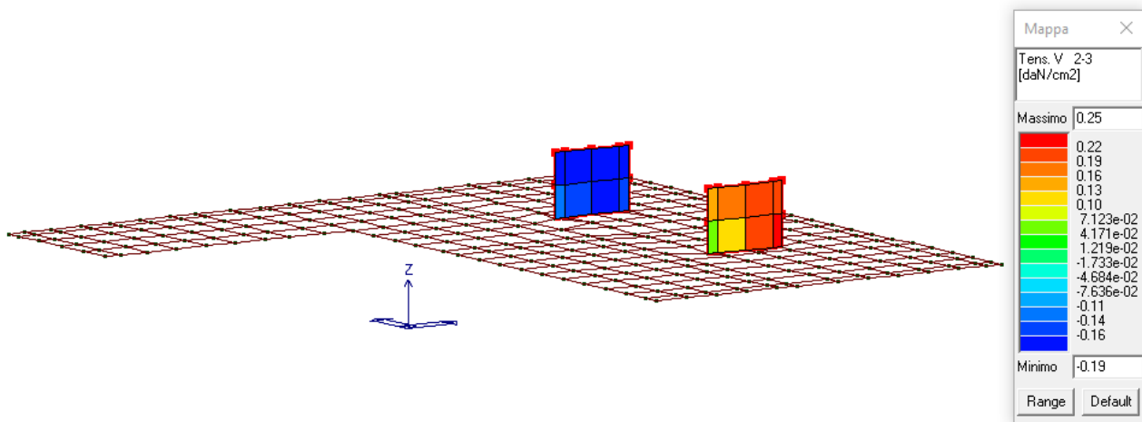
Figura 30: Tensioni di taglio 2-3 in daN/cm 2 .
