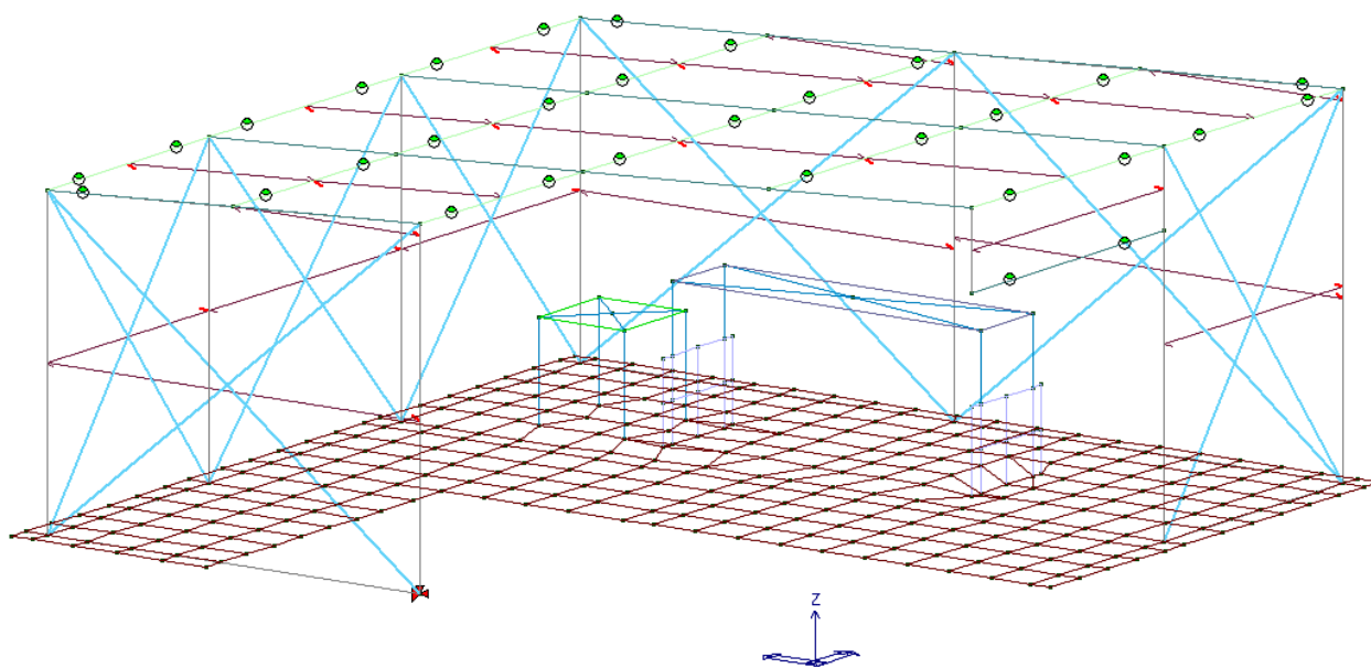
Figura 17: Vista complessiva del modello di calcolo
