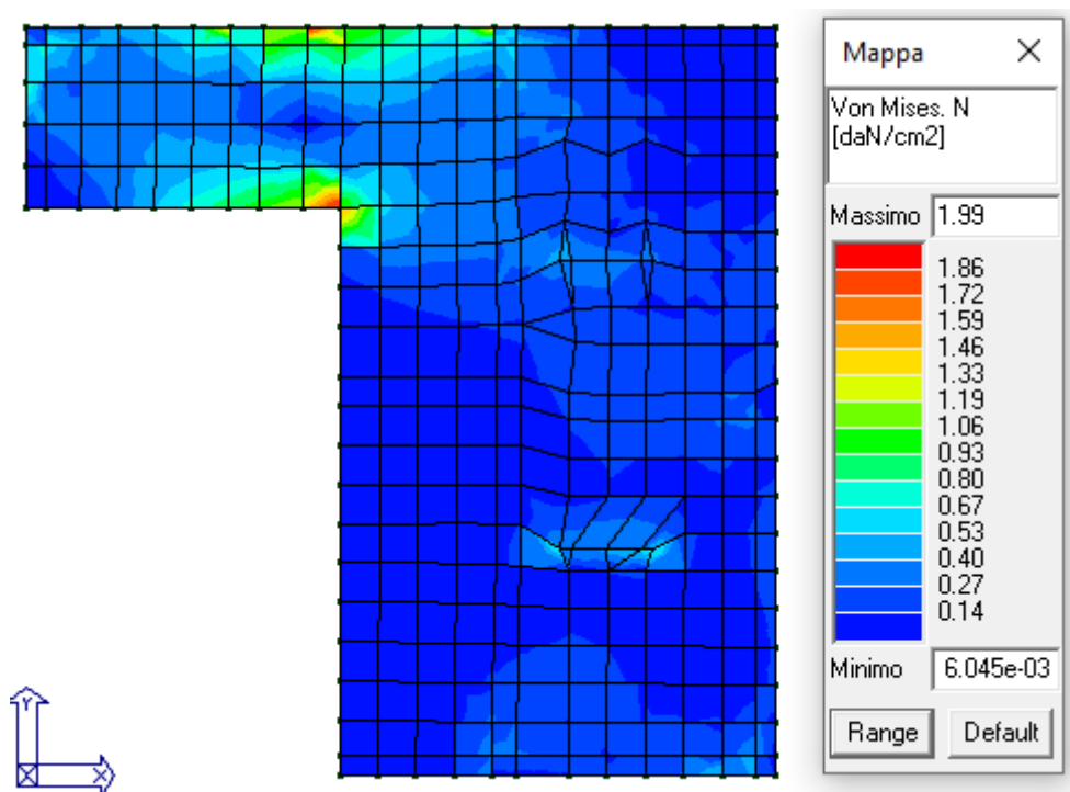
Figura 18: Tensioni di membrana (N) tramite formulazione di Von Mises.
