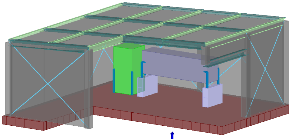
Figura 2: Vista modello - ProSap .
