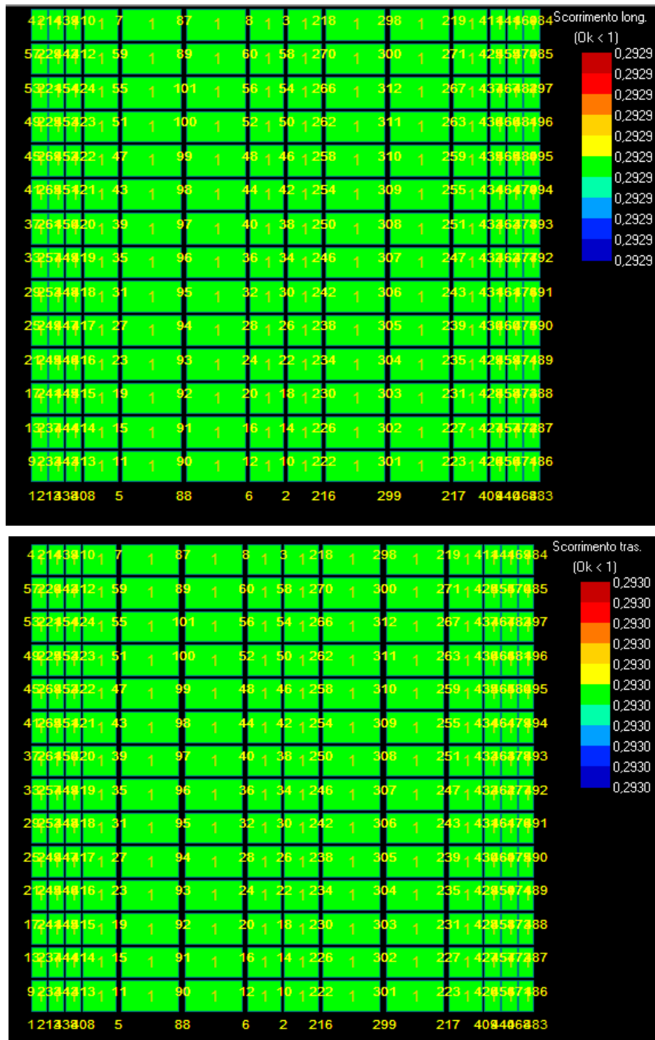
Figura 13: Scorrimento - Stratigrafia 1.
