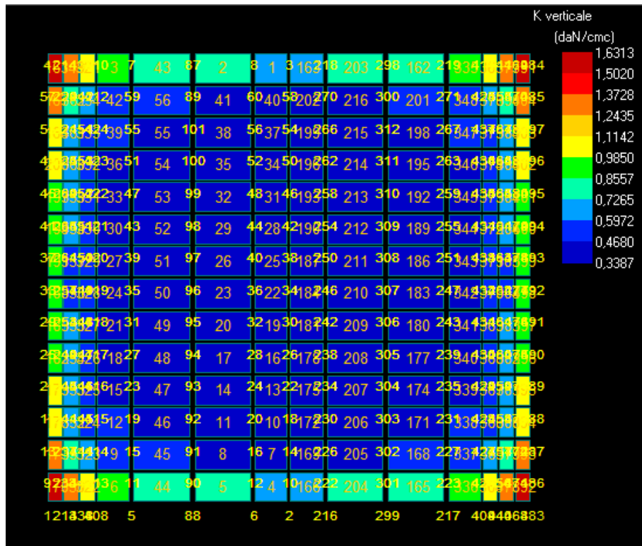
Figura 7: Costante di Winkler – stratigrafia 1.
