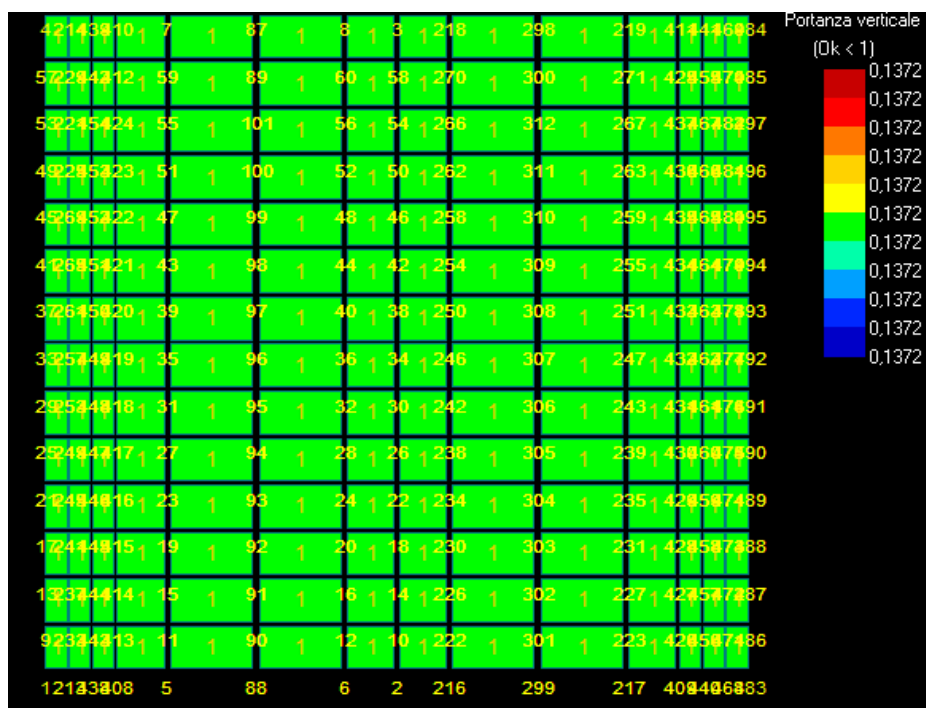
Figura 12: Portata – carico limite - Stratigrafia 2.
