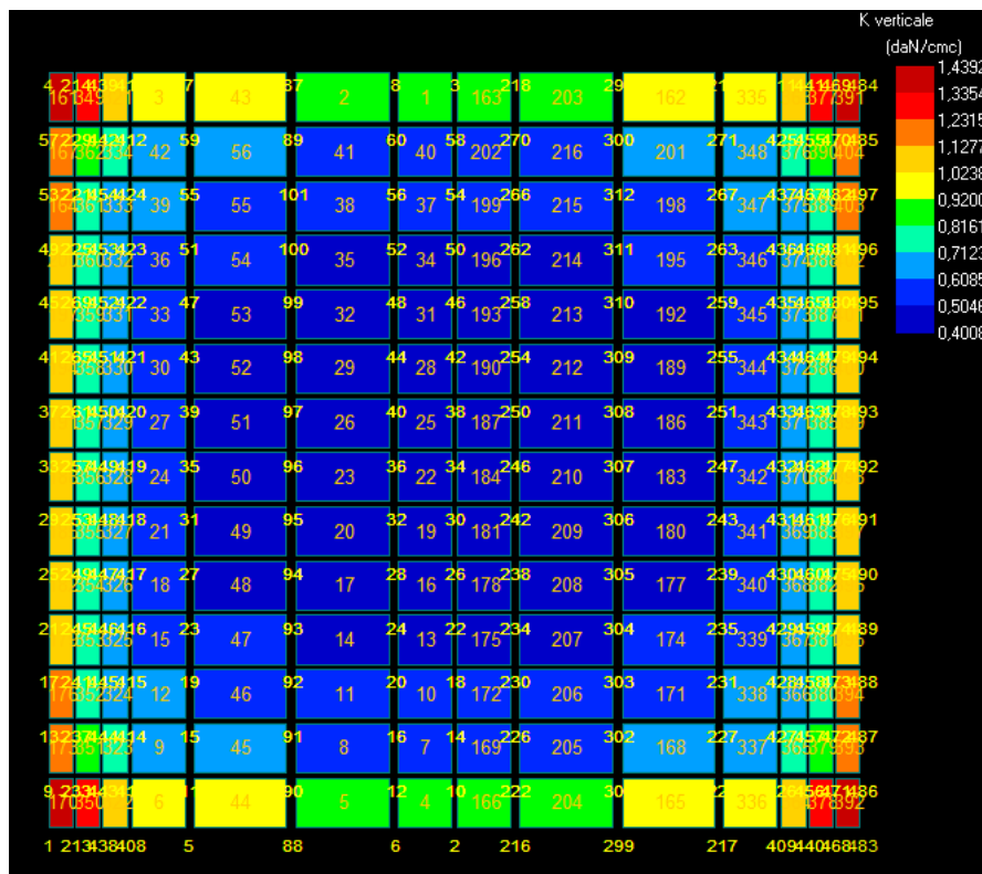
Figura 8: Costante di Winkler – stratigrafia 2.
