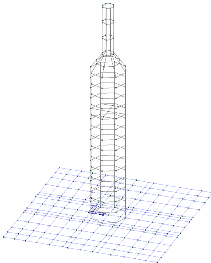
Figura 16: Vista complessiva del modello di calcolo
