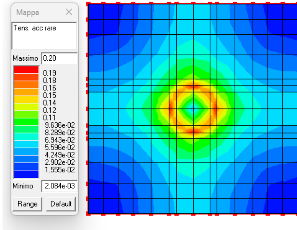
Figura 25: Verifica tensioni rare nell'acciaio.
