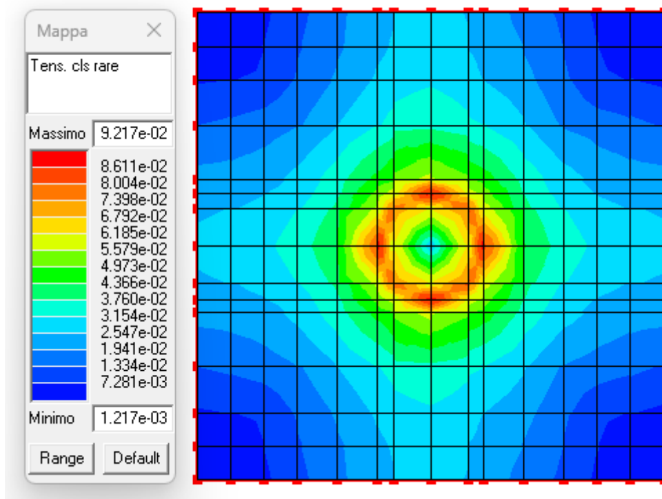
Figura 24: Verifica tensioni rare nel cls.
