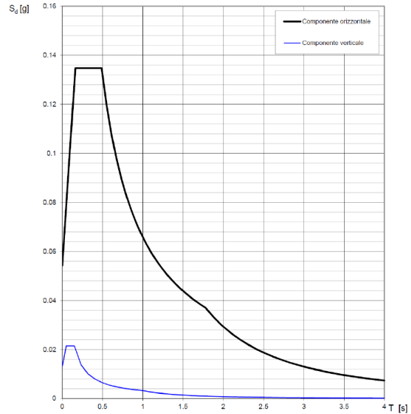
Figura 15: Parametri spettro di risposta SLD.
