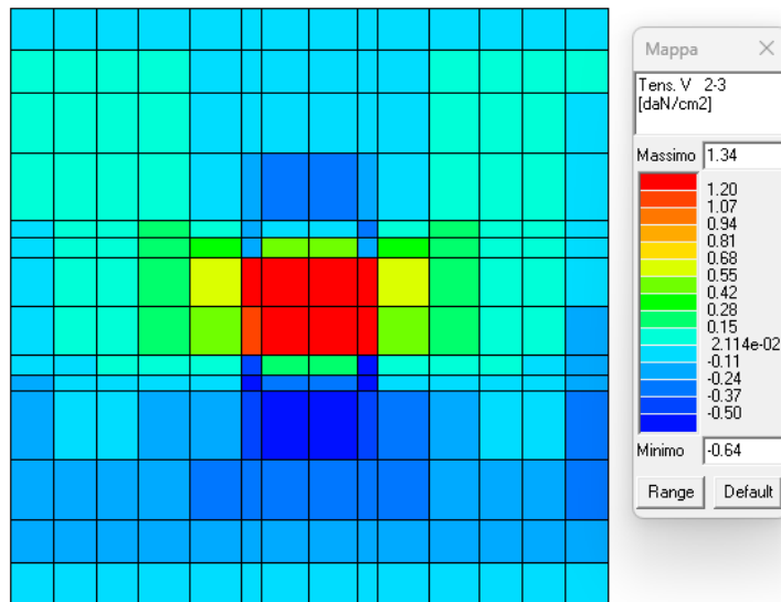
Figura 20: Tensioni di taglio 2-3 in daN/cm 2 .
