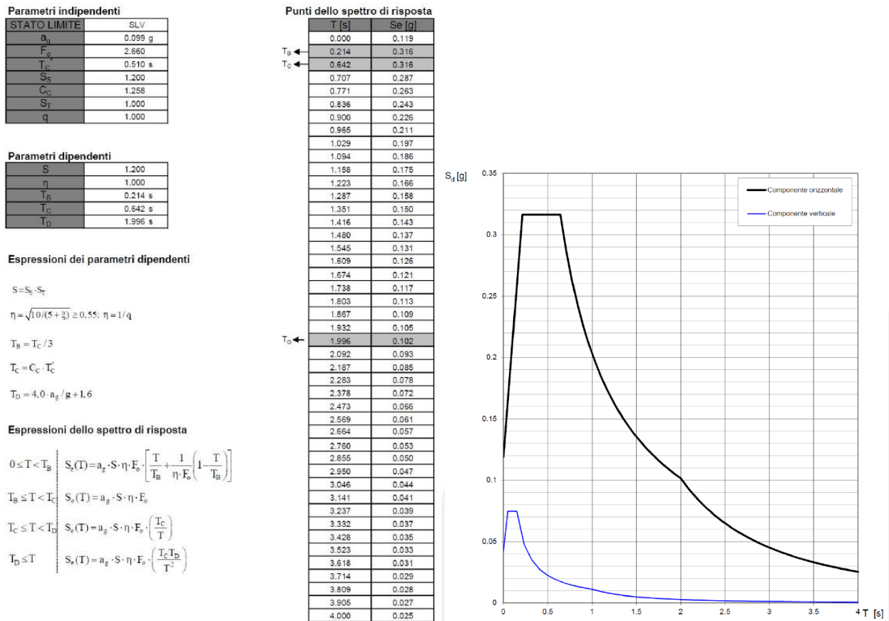
Figura 14: Parametri spettro di risposta SLV.
