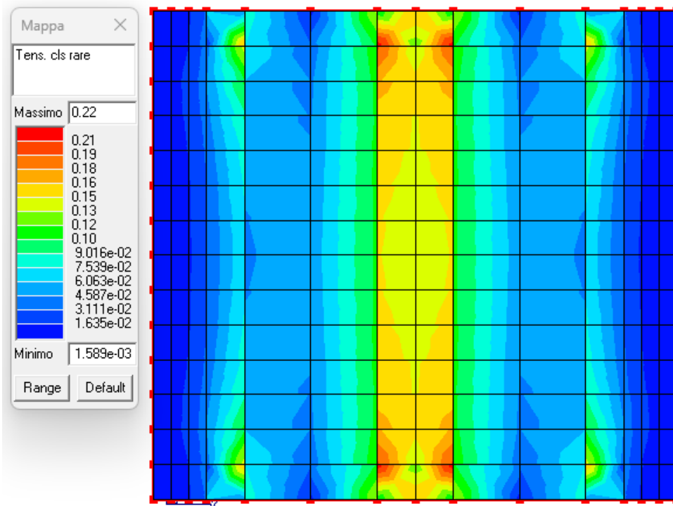
Figura 23: Verifica tensioni rare nel cls.
