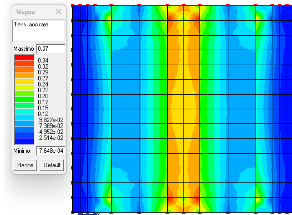
Figura 24: Verifica tensioni rare nell'acciaio.
