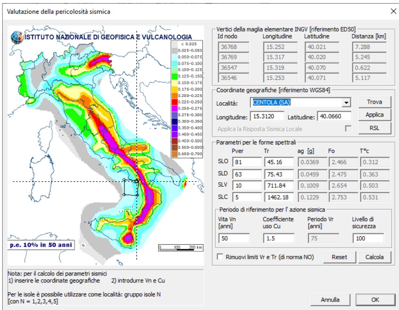
Figura 4: Valutazione della pericolosità sismica.
