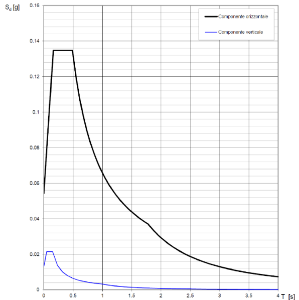
Figura 14: Parametri spettro di risposta SLD.
