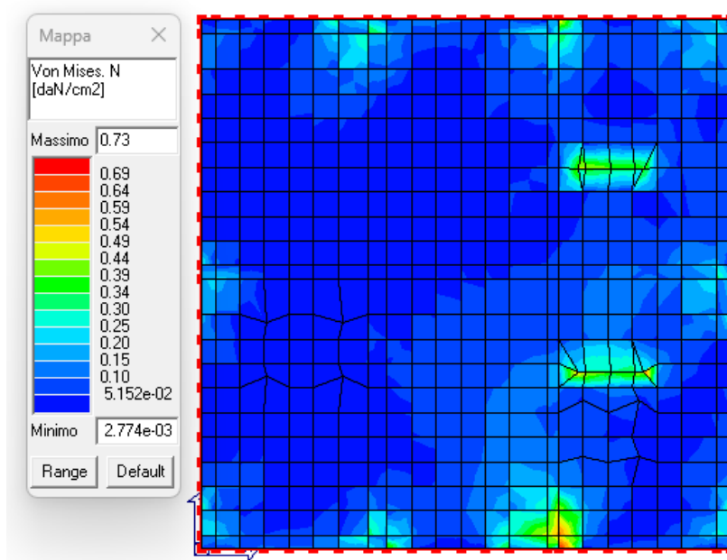
Figura 18: Tensioni di membrana (N) tramite formulazione di Von Mises.
