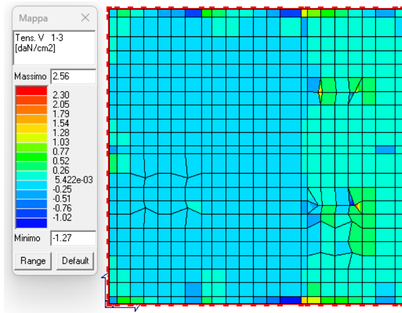
Figura 20: Tensioni di taglio 1-3 in daN/cm 2 .
