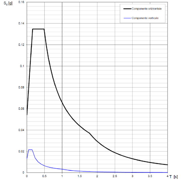
Figura 16: Parametri spettro di risposta SLD.
