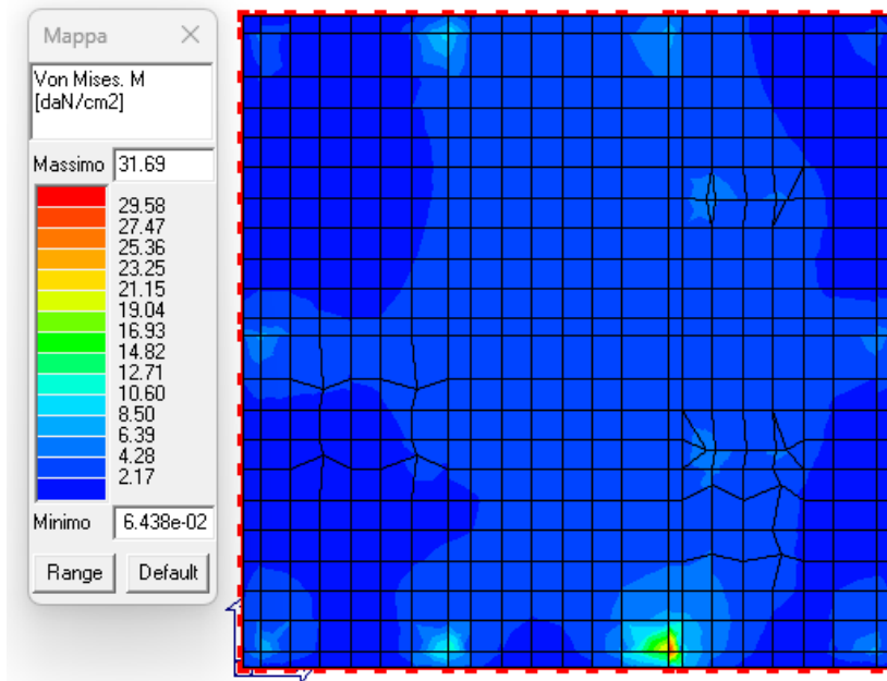
Figura 19: Tensioni di flessione (M) tramite formulazione di Von Mises.
