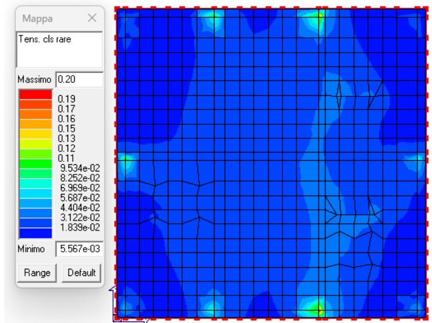
Figura 25: Verifica tensioni rare nel cls.
