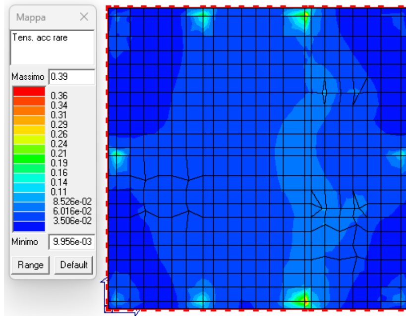
Figura 26: Verifica tensioni rare nell'acciaio.
