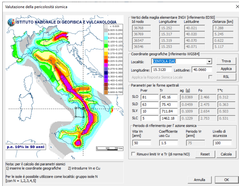
Figura 6: Valutazione della pericolosità sismica.
