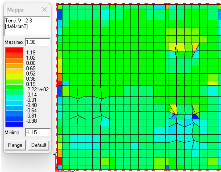
Figura 21: Tensioni di taglio 2-3 in daN/cm 2 .
