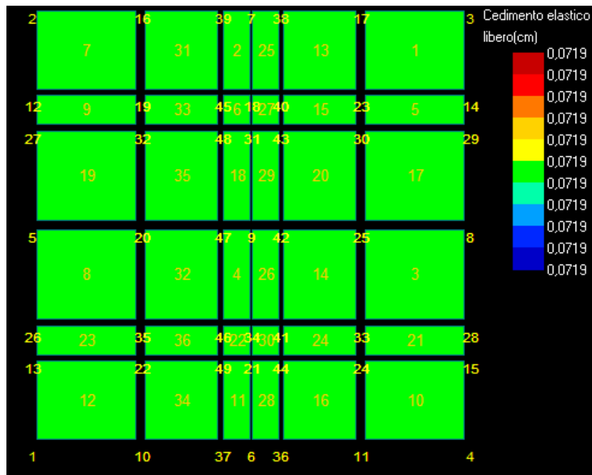
Figura 25: Cedimento - Stratigrafia 3.
