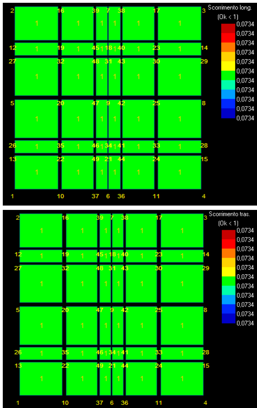
Figura 19: Scorrimento - Stratigrafia 1.
