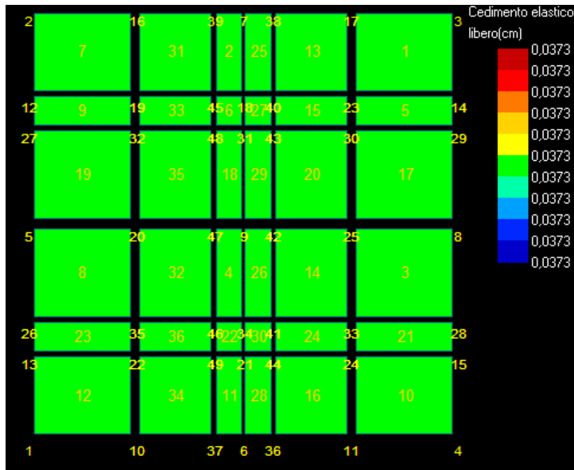
Figura 23: Cedimento - Stratigrafia 1.
