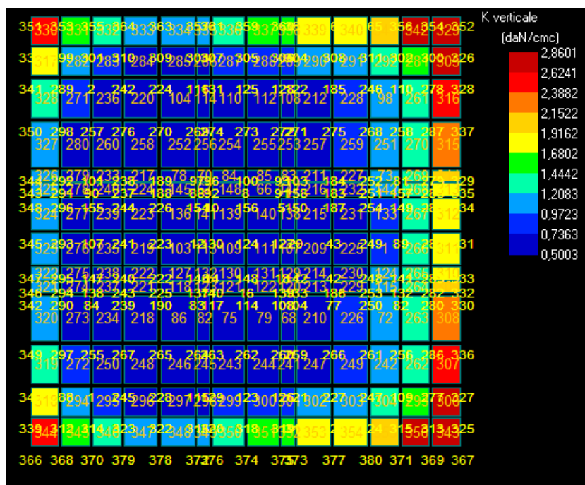
Figura 9: Costante di Winkler – stratigrafia 1.
