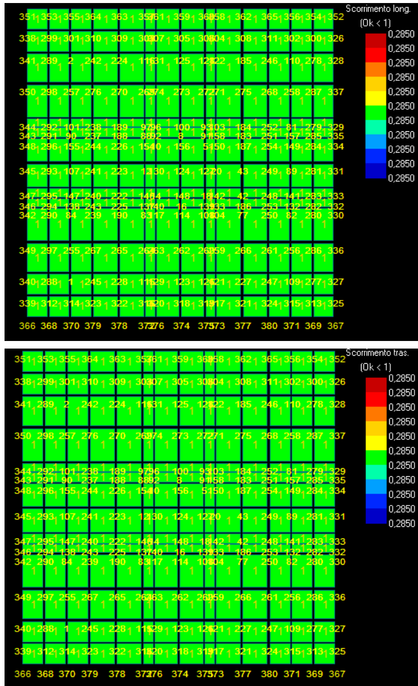
Figura 22: Scorrimento - Stratigrafia 4.
