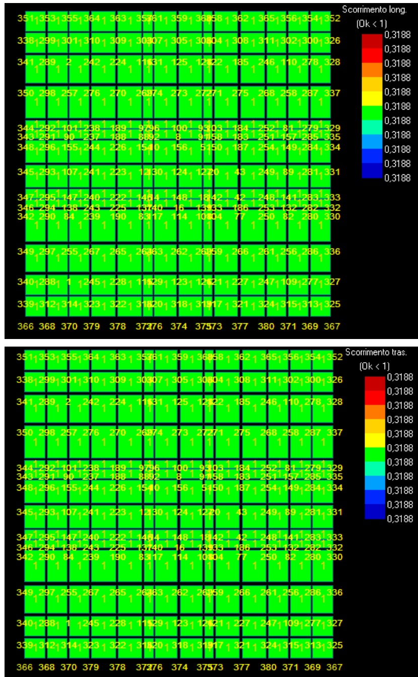
Figura 21: Scorrimento - Stratigrafia 3.
