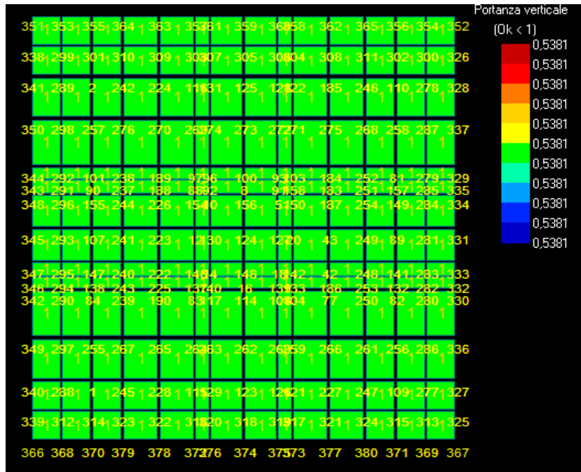
Figura 18: Portata – carico limite - Stratigrafia 4.
