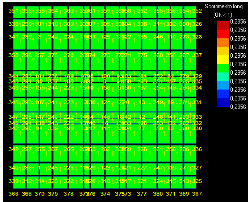
Figura 19: Scorrimento - Stratigrafia 1.
