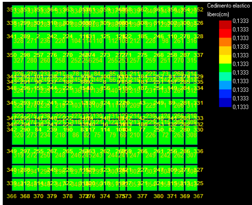
Figura 26: Cedimento - Stratigrafia 4.
