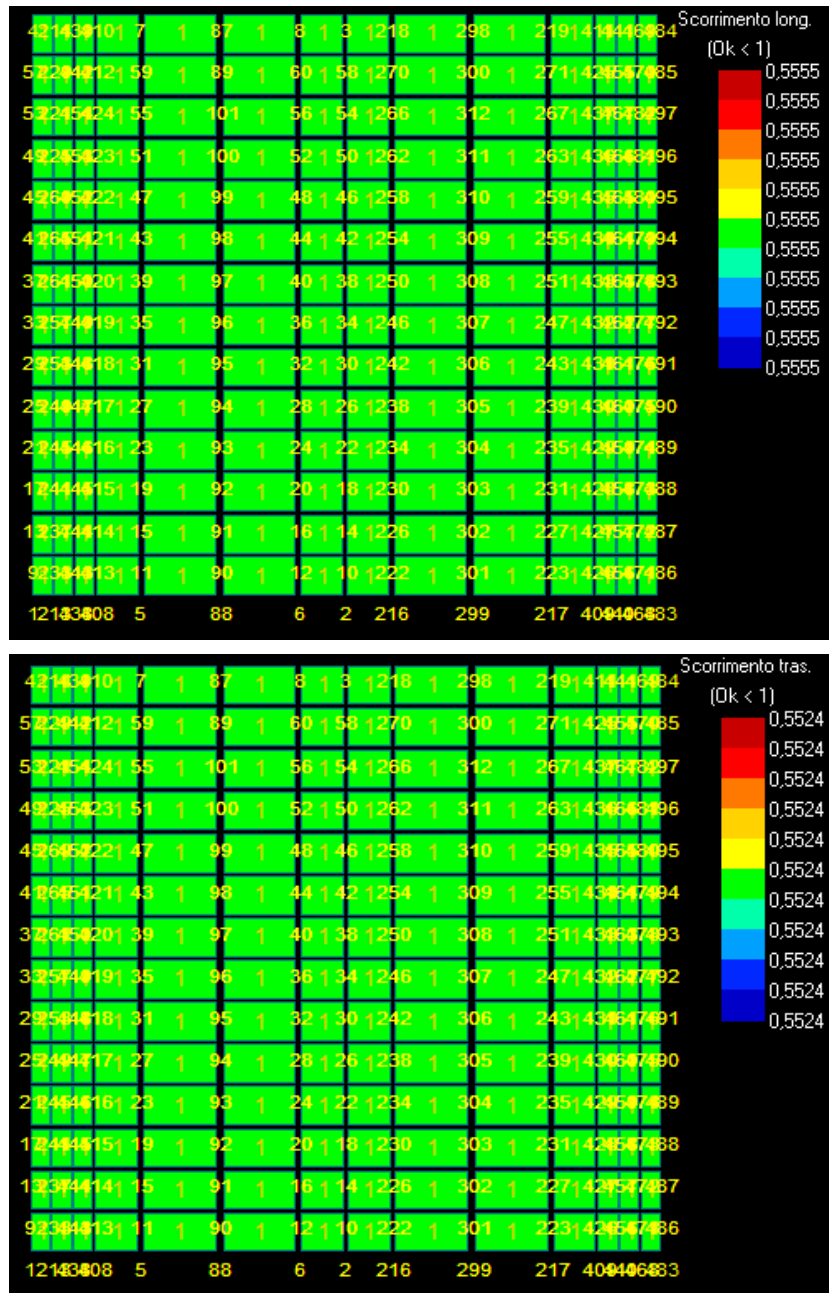
Figura 22: Scorrimento - Stratigrafia 4.
