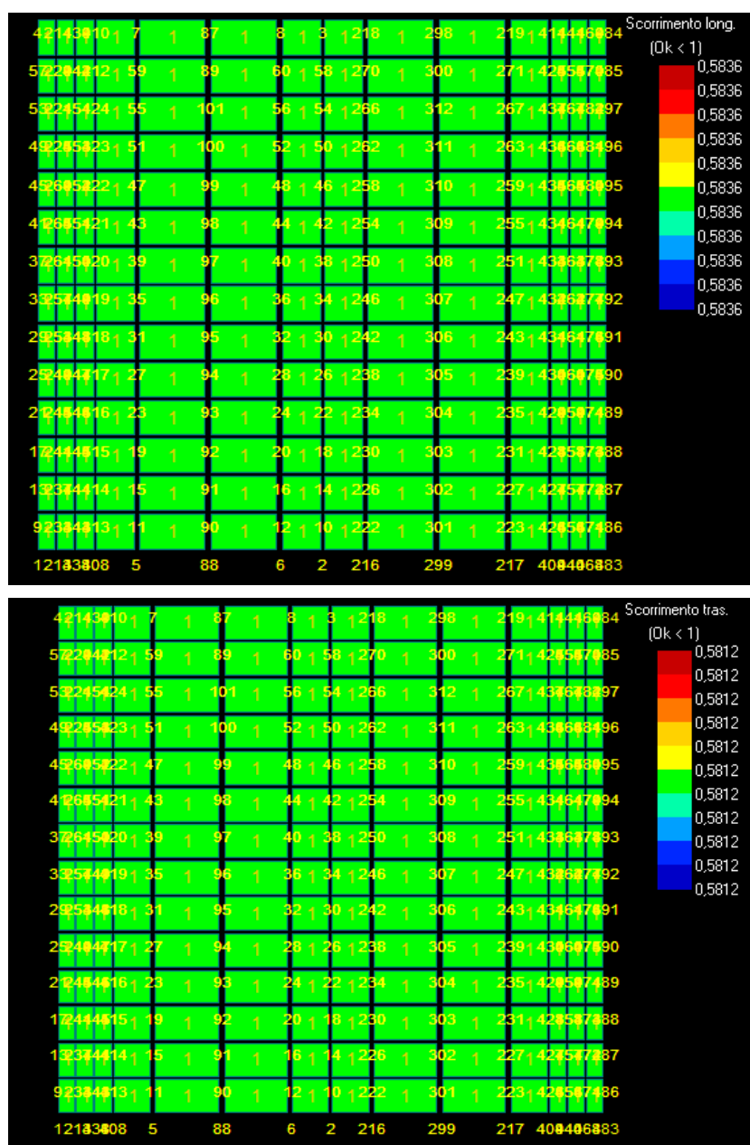
Figura 19: Scorrimento - Stratigrafia 1.
