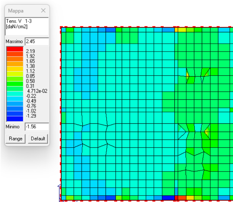
Figura 20: Tensioni di taglio 1-3 in daN/cm 2 .
