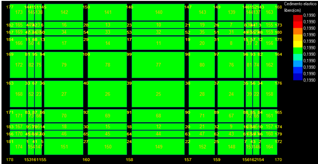
Figura 16: Cedimento - Stratigrafia 2.
