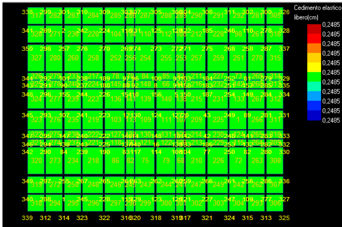
Figura 15: Cedimento - Stratigrafia 1.
