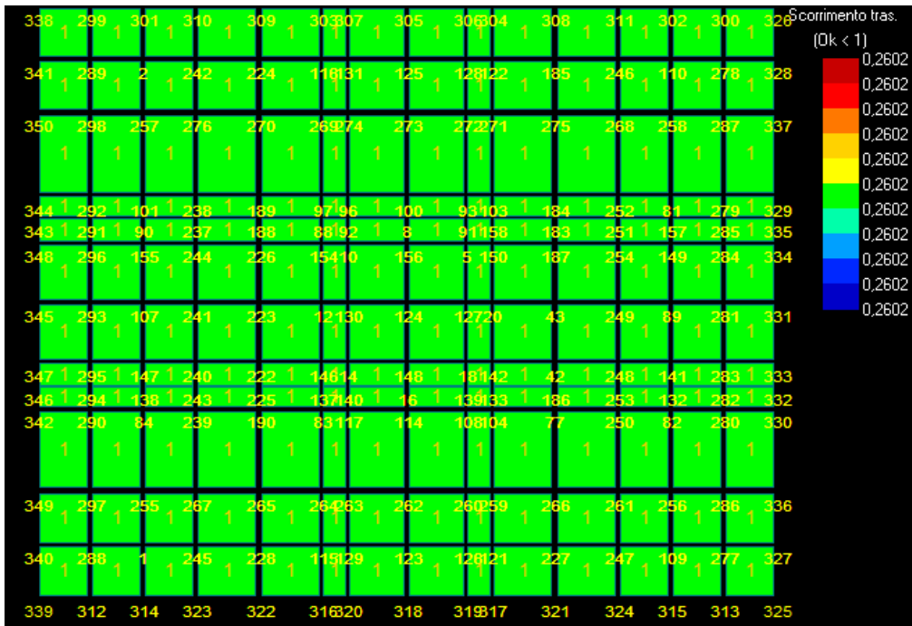
Figura 13: Scorrimento - Stratigrafia 1.
