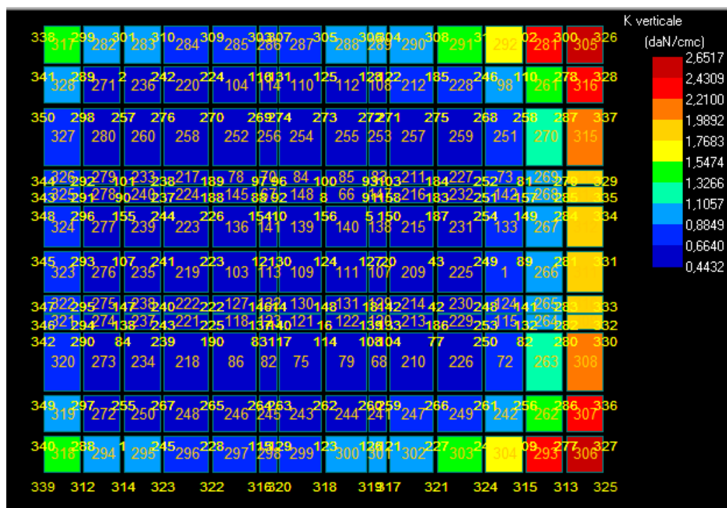
Figura 8: Costante di Winkler – stratigrafia 2.
