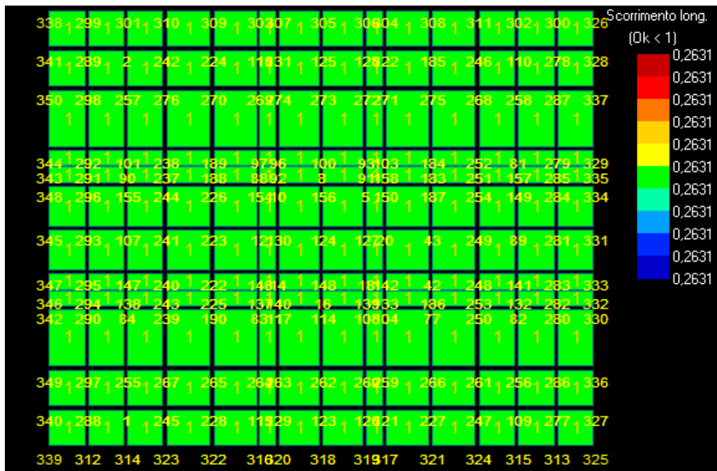
Figura 13: Scorrimento - Stratigrafia 1.
