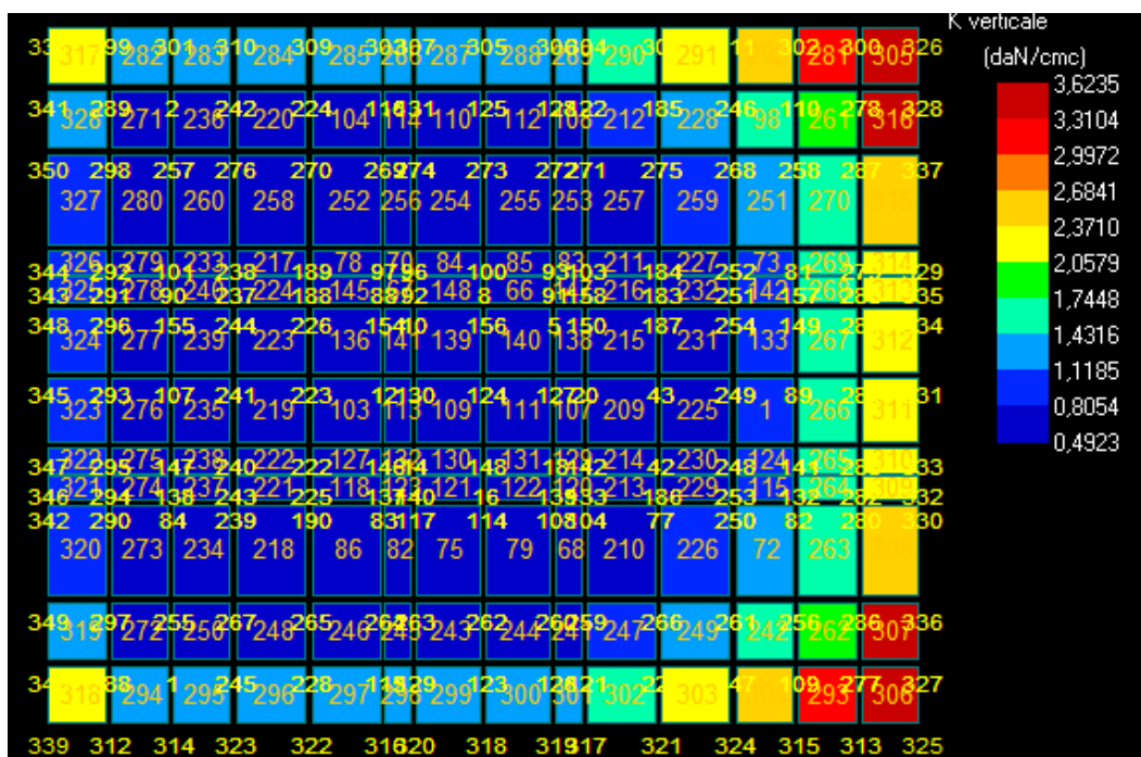
Figura 7: Costante di Winkler – stratigrafia 1.
