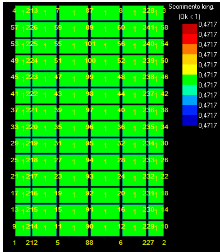
Figura 13: Scorrimento - Stratigrafia 1.
