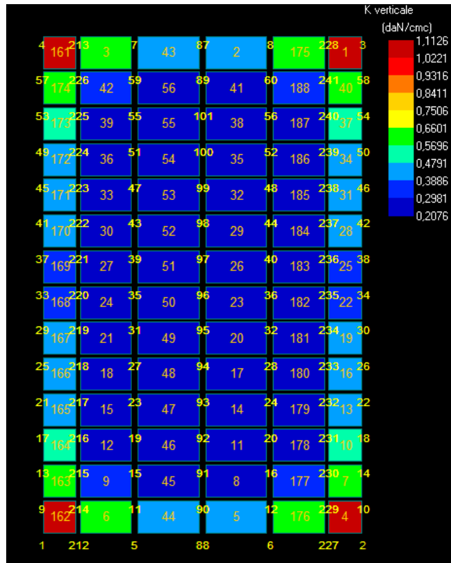
Figura 7: Costante di Winkler – stratigrafia 1.
