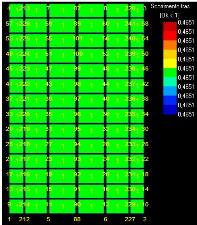
Figura 13: Scorrimento - Stratigrafia 1.
