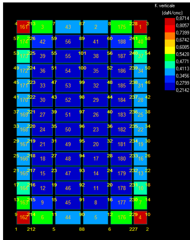
Figura 8: Costante di Winkler – stratigrafia 2.
