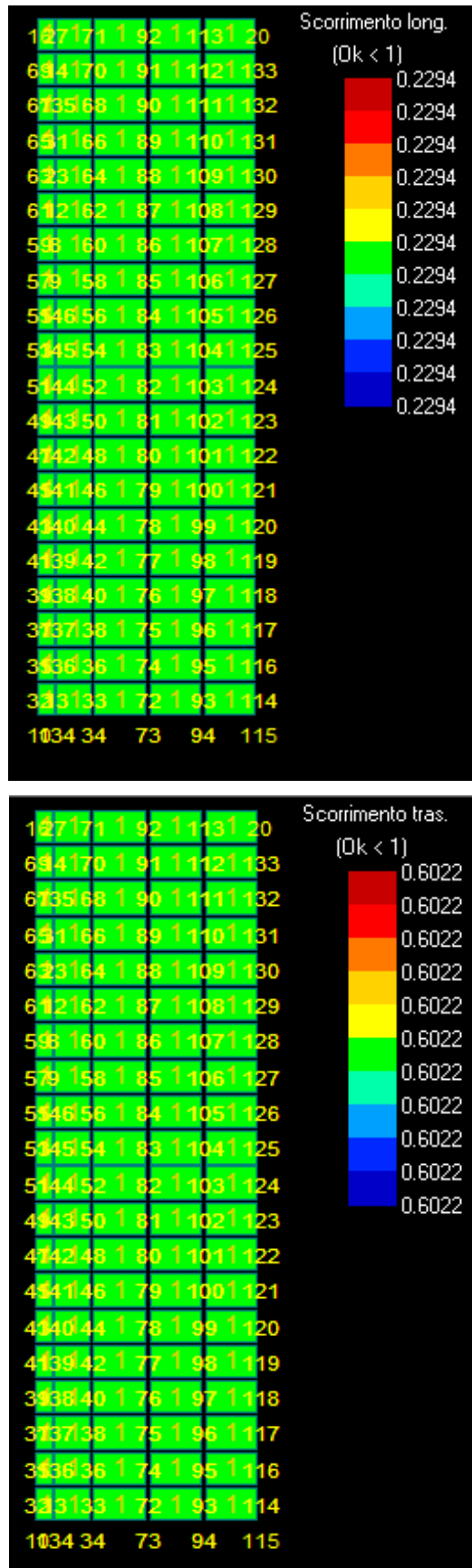
Figura 14: Scorrimento - Stratigrafia 2.
