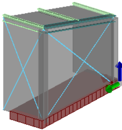
Figura 2: Vista modello - ProSap .
