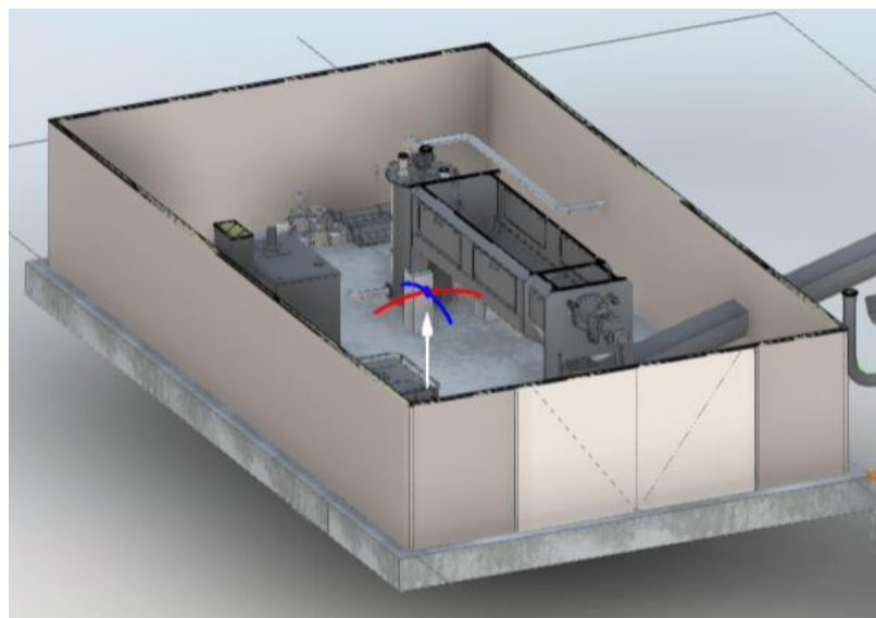
Figura 3: Estratto da modellazione BIM.
