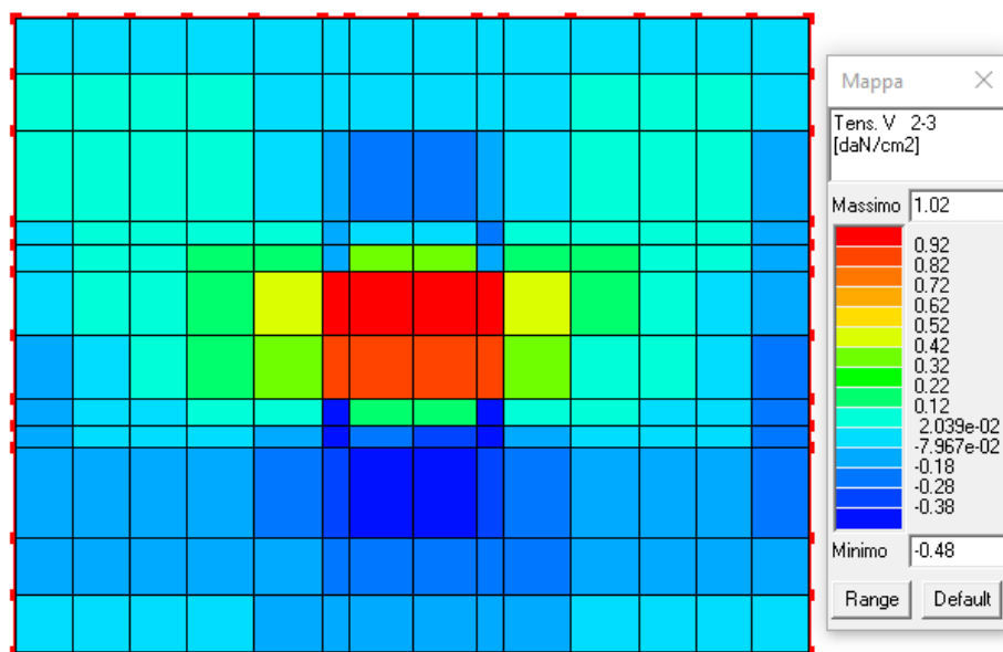
Figura 20: Tensioni di taglio 2-3 in daN/cm 2 .
