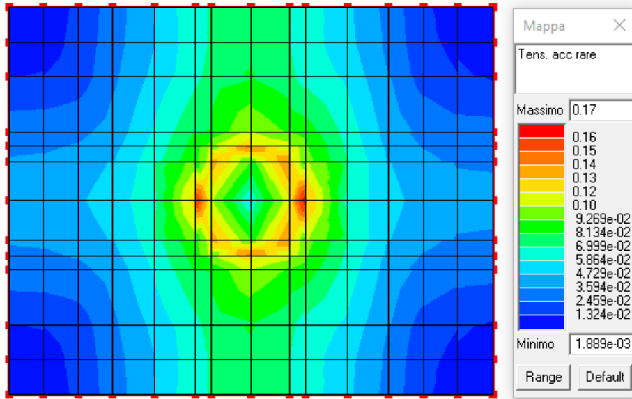
Figura 25: Verifica tensioni rare nell'acciaio.
