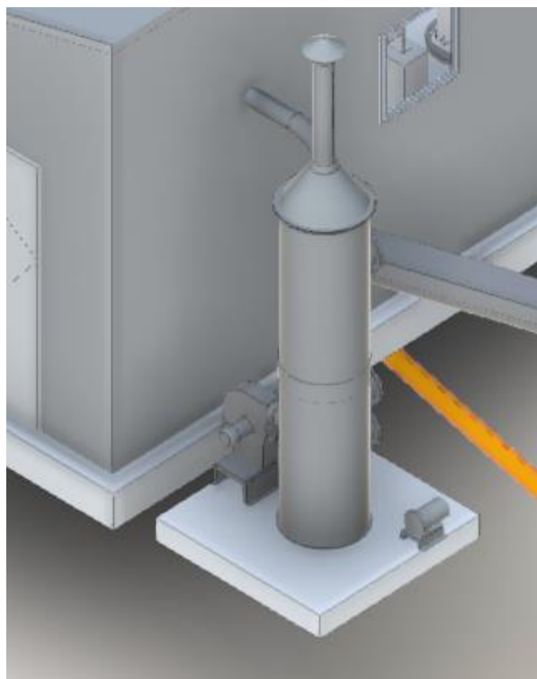
Figura 3: Estratto da modellazione BIM.
