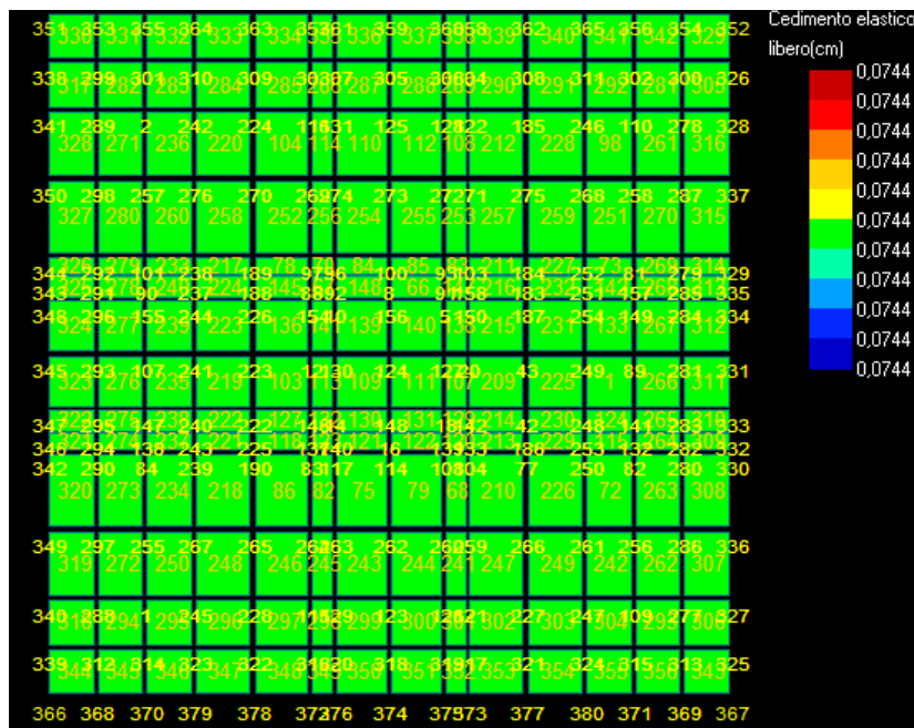
Figura 15: Cedimento - Stratigrafia 1.
