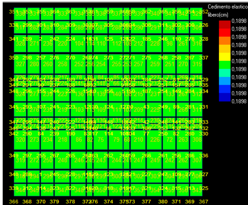
Figura 16: Cedimento - Stratigrafia 2.
