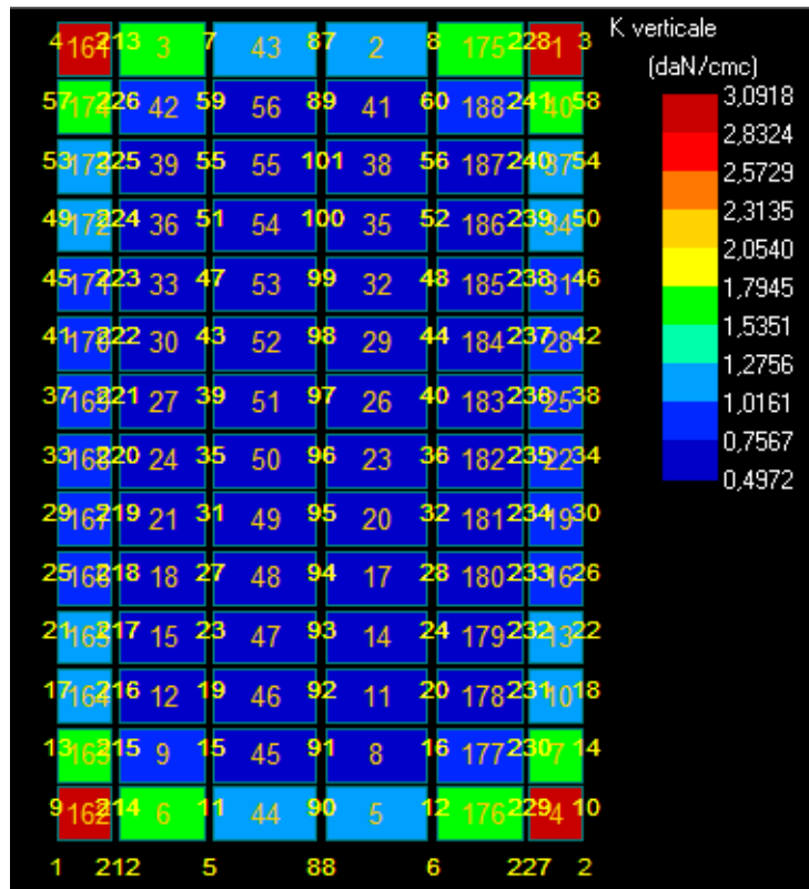
Figura 7: Costante di Winkler – stratigrafia 1.
