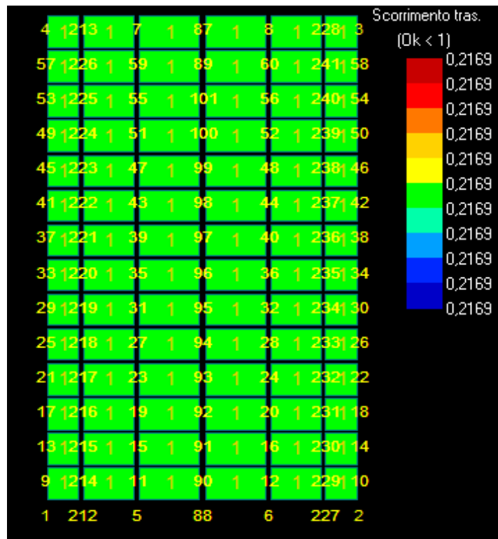
Figura 13: Scorrimento - Stratigrafia 1.
