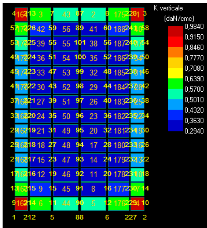
Figura 8: Costante di Winkler – stratigrafia 2.
