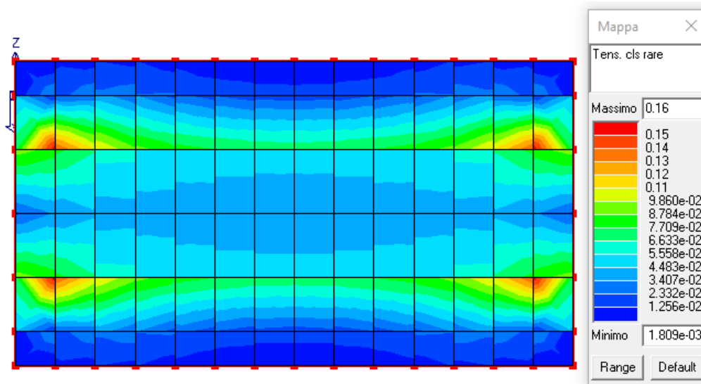
Figura 23: Verifica tensioni rare nel cls.
