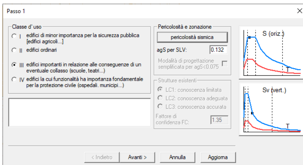
Figura 5: Classe d'uso.
