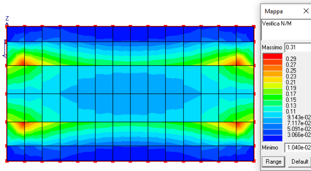
Figura 20: Verifica N/M
