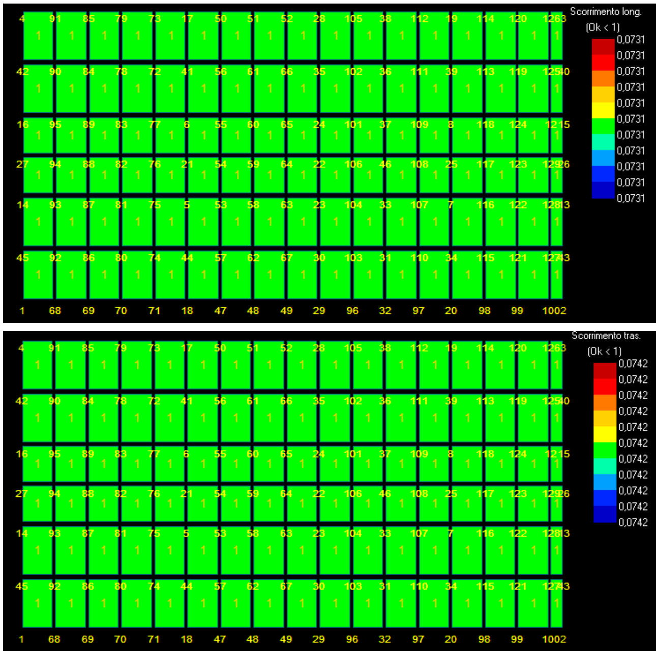
Figura 19: Scorrimento - Stratigrafia 1.
