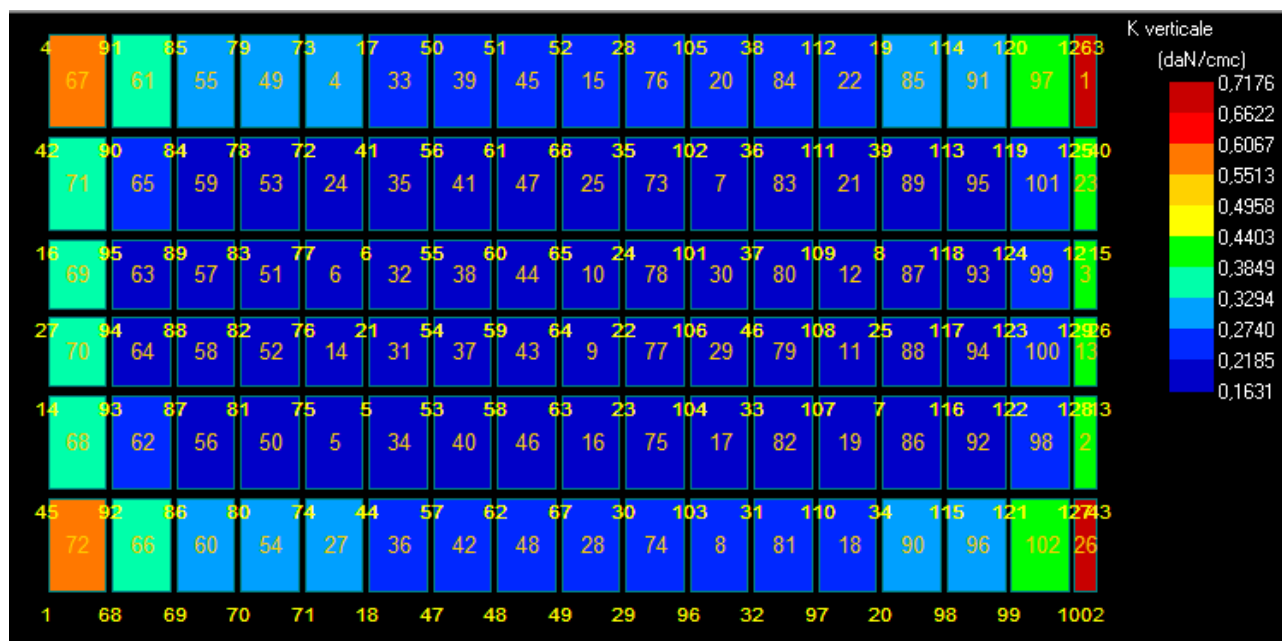
Figura 12: Costante di Winkler – stratigrafia 4.
