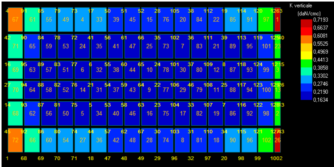
Figura 10: Costante di Winkler – stratigrafia 2.
