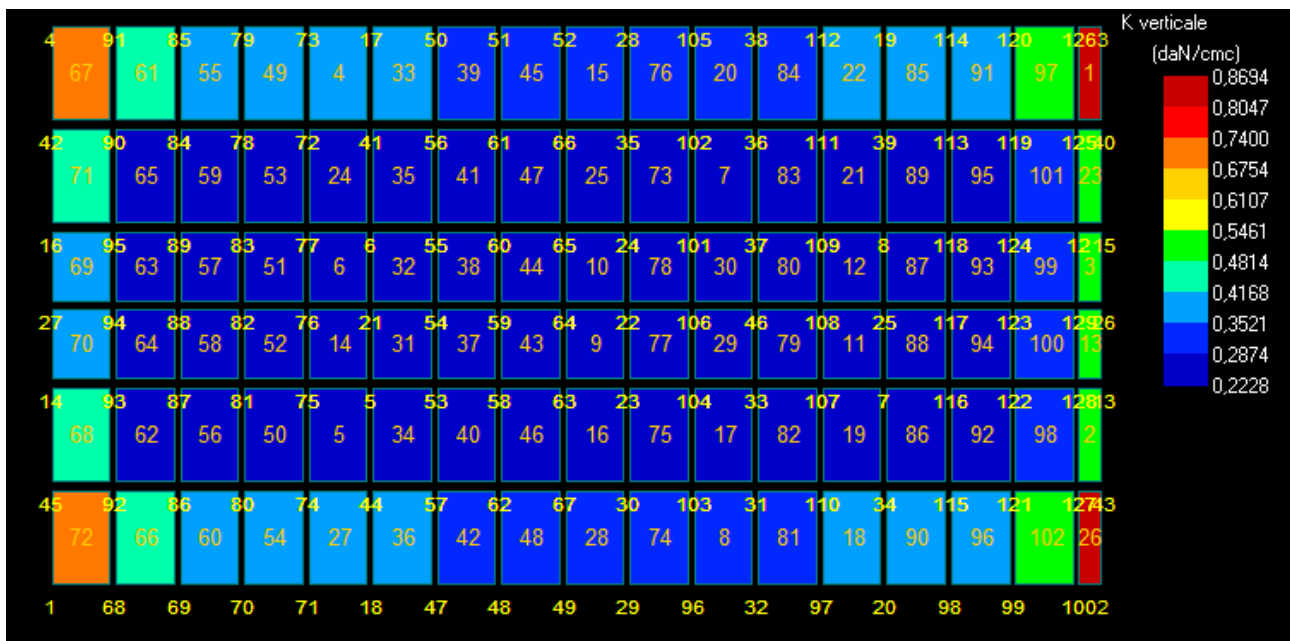
Figura 11: Costante di Winkler – stratigrafia 3.
