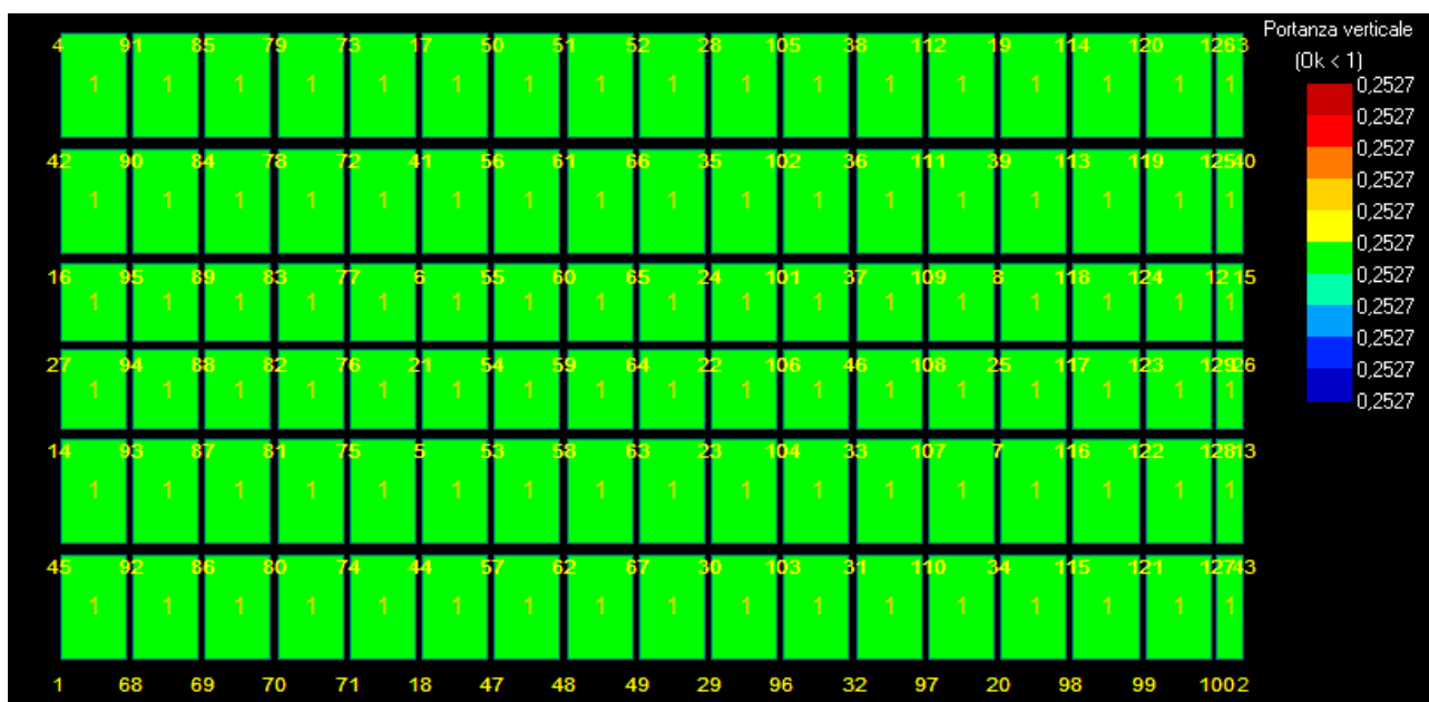
Figura 17: Portata – carico limite - Stratigrafia 3.
