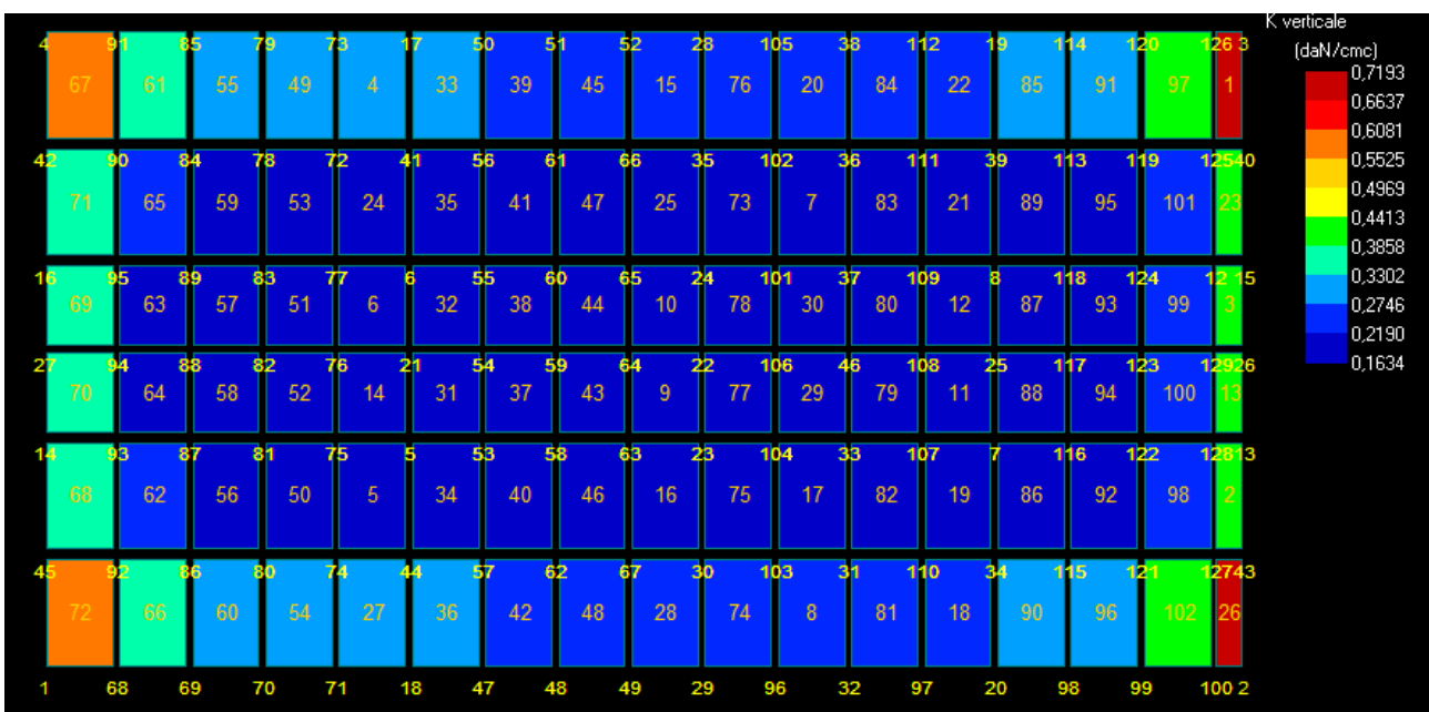
Figura 9: Costante di Winkler – stratigrafia 1.
