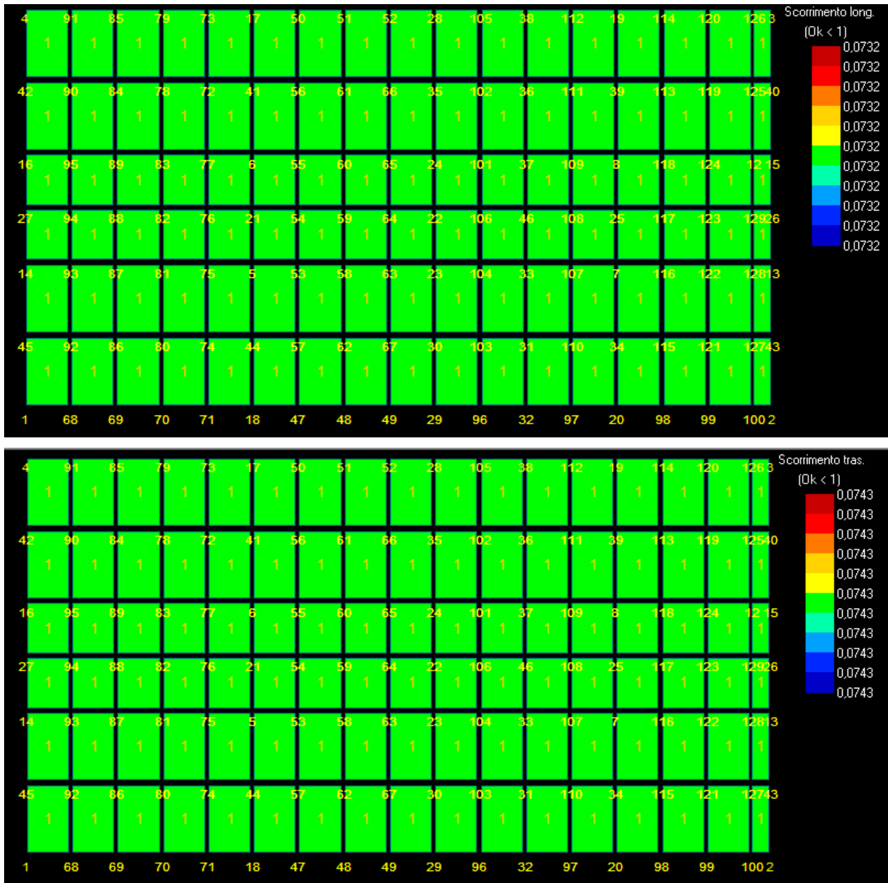
Figura 22: Scorrimento - Stratigrafia 4.
