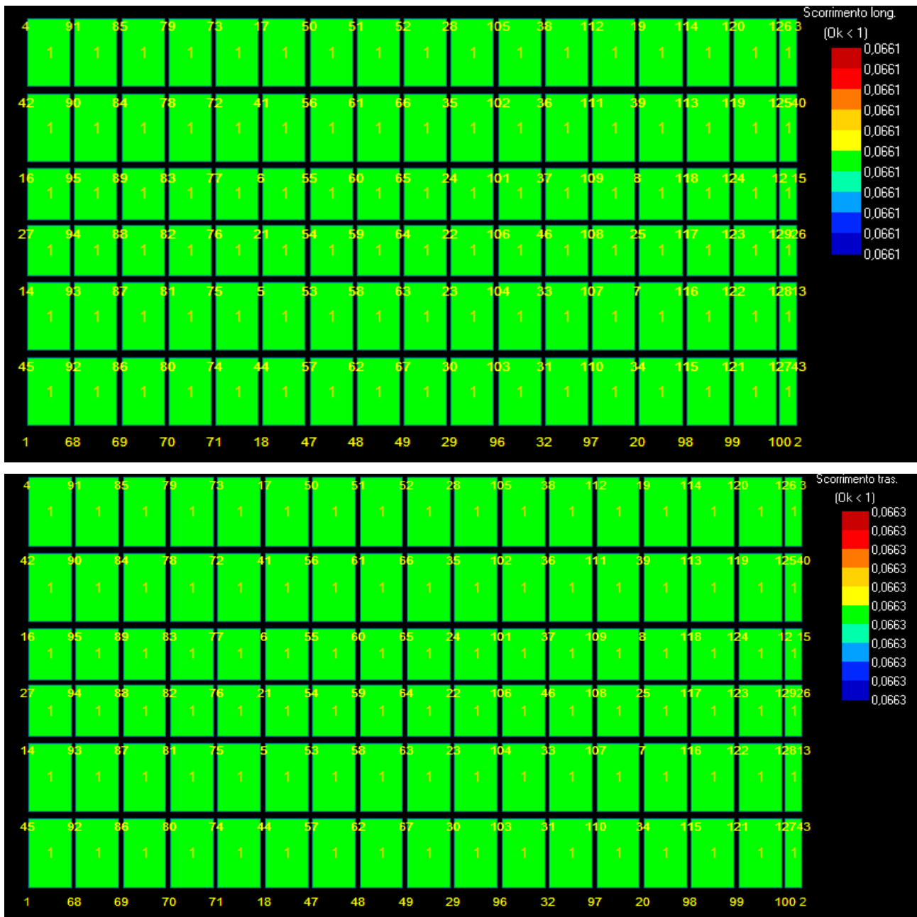
Figura 21: Scorrimento - Stratigrafia 3.
