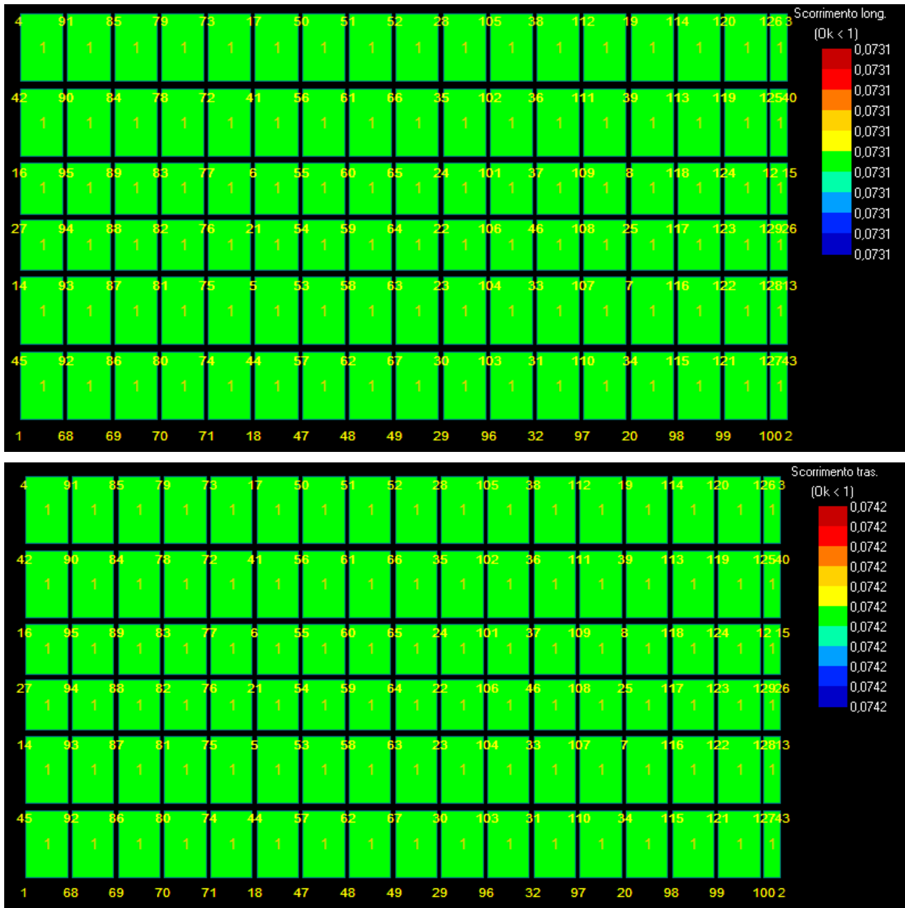
Figura 20: Scorrimento - Stratigrafia 2.
