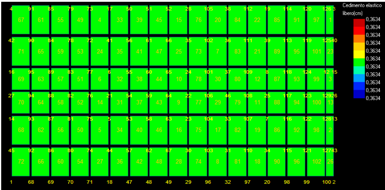
Figura 26: Cedimento - Stratigrafia 4.
