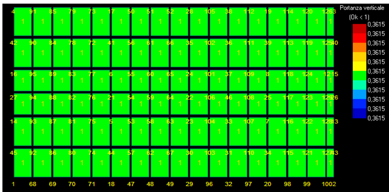
Figura 18: Portata – carico limite - Stratigrafia 4.
