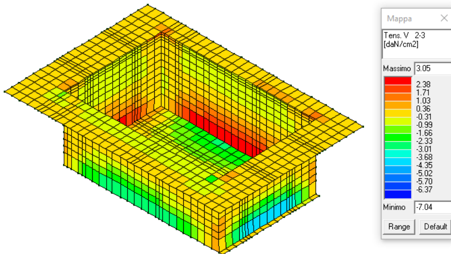
Figura 22: Tensioni di taglio 2-3 in daN/cm 2 .
