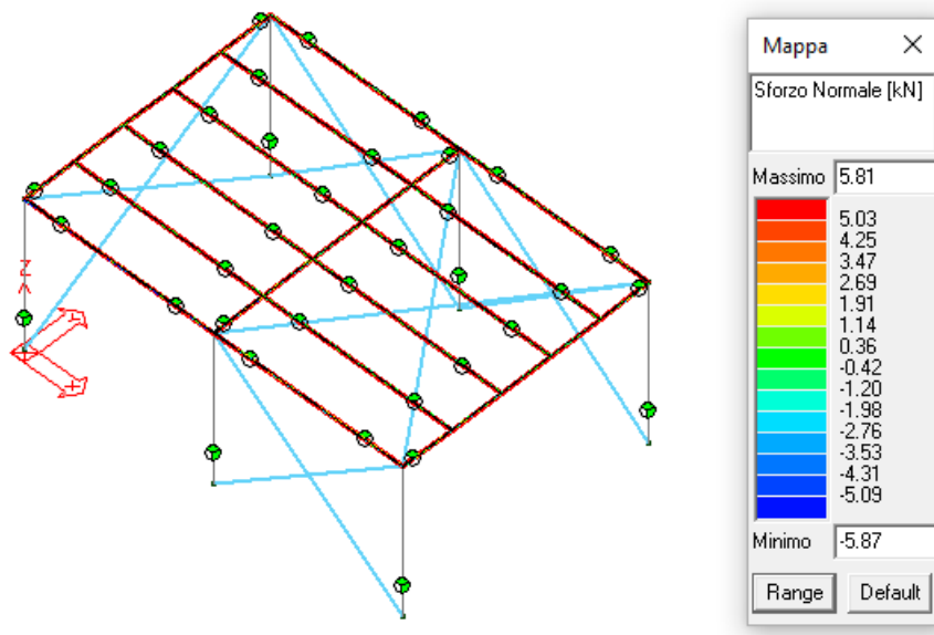
Figura 41: Azioni assiali (N) sulle travi.
