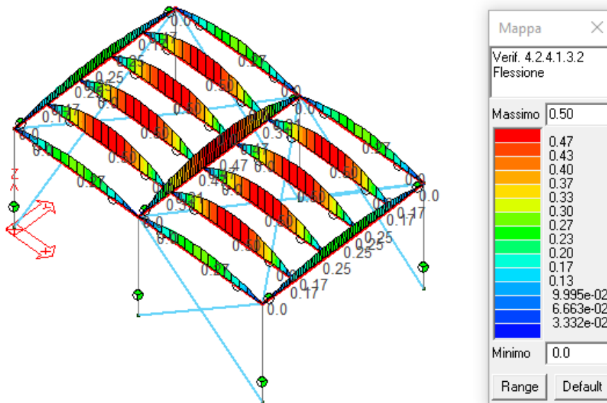
Figura 47: Verifica ad instabilità flessionale travi.
