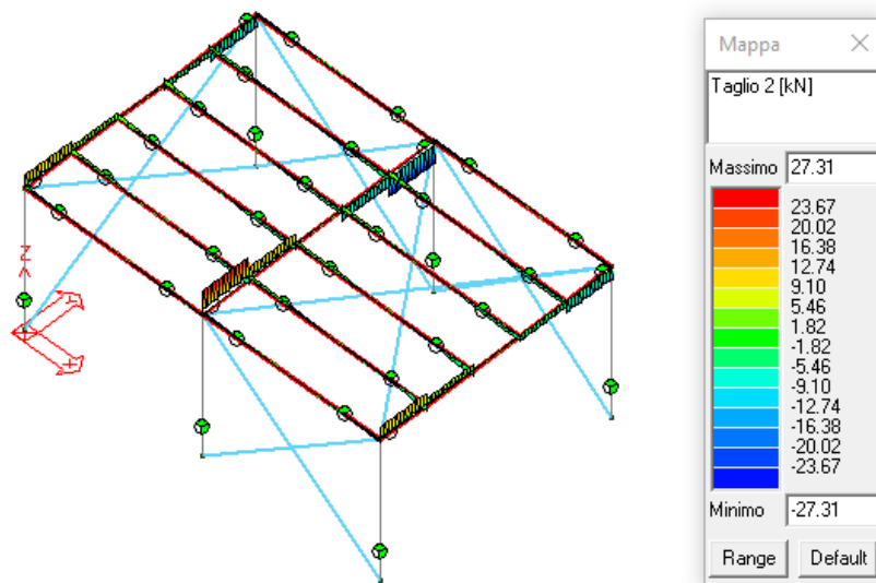
Figura 42: Azioni di taglio V2-2 (N) sulle travi.
