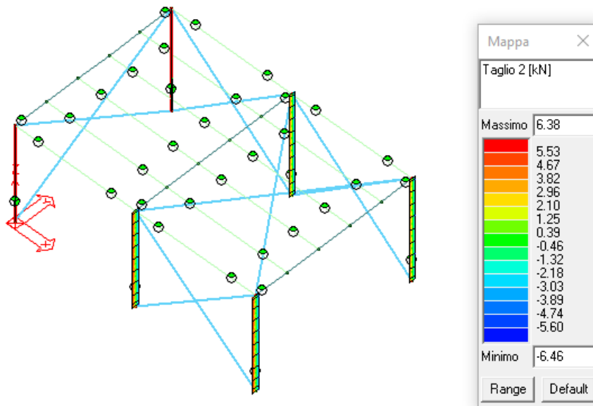
Figura 29: Azioni di taglio V2-2 (N) sulle colonne.
