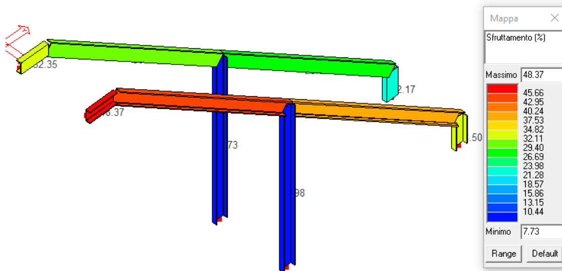
Figura 55: Sfruttamento (%) scala.
