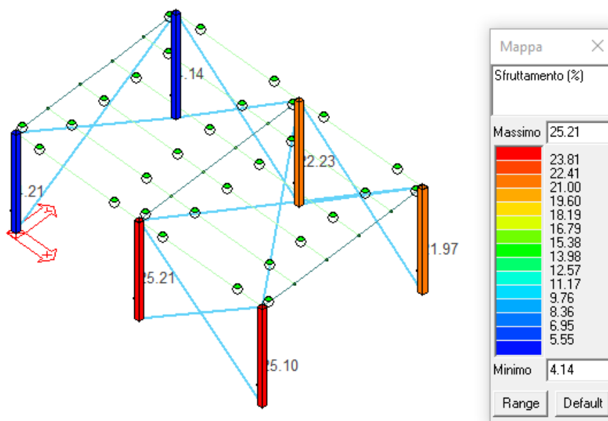
Figura 33: Sfruttamento (%) colonne.
