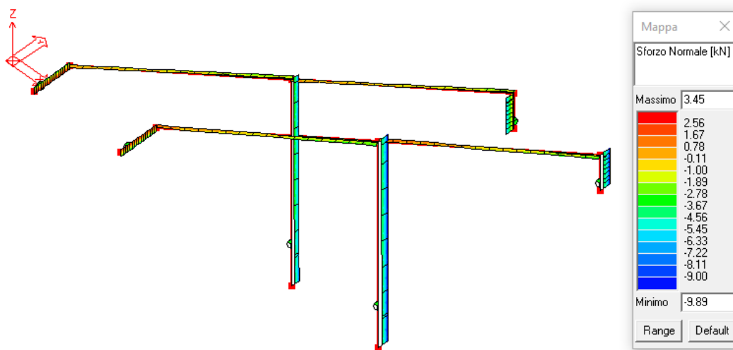
Figura 52: Azioni assiali (N) sulle travi.
