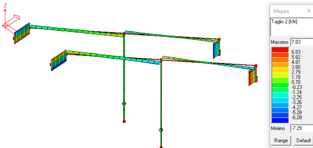
Figura 53: Azioni di taglio V2-2 (N) sulle travi.
