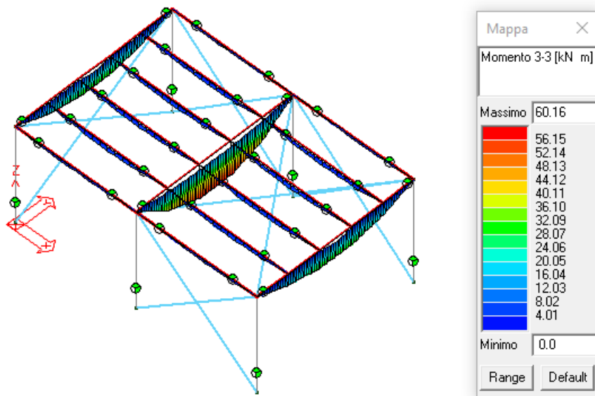
Figura 43: Azioni di taglio M3-3 (N) sulle colonne
