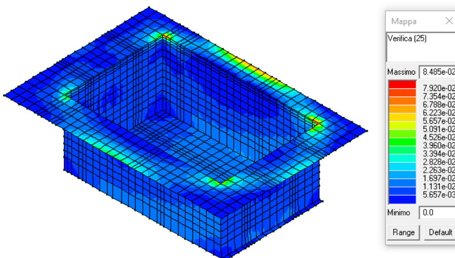
Figura 24: Verifica 25
