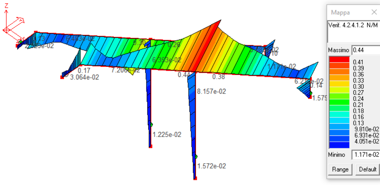
Figura 56: Verifica N/M scala.
