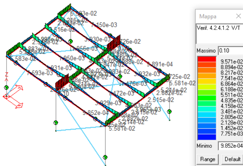
Figura 46: Verifica a taglio torsione travi.
