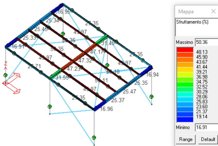
Figura 44: Sfruttamento (%) travi.
