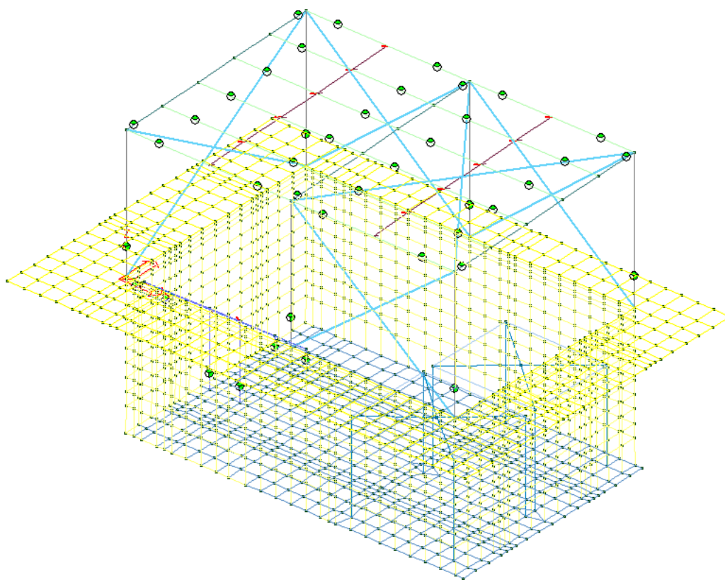
Figura 18: Vista complessiva del modello di calcolo
