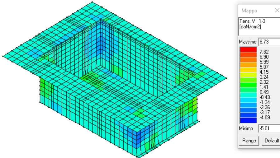
Figura 21: Tensioni di taglio 1-3 in daN/cm 2 .
