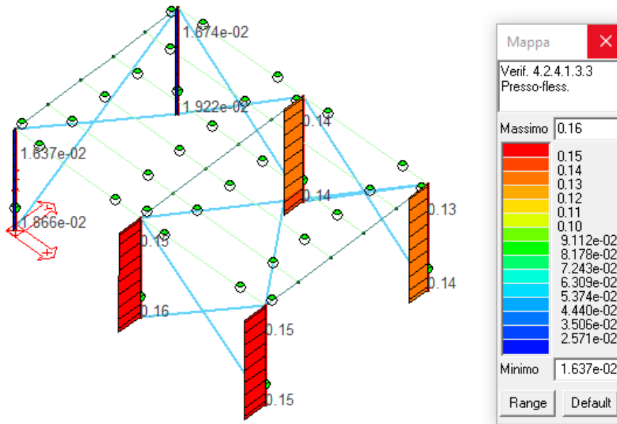
Figura 36: Verifica ad instabilità presso-flessionale colonne.
