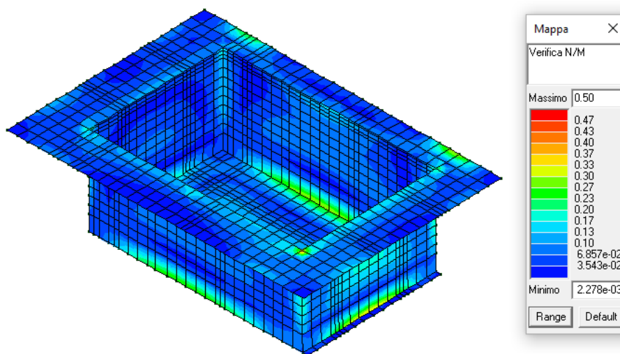
Figura 23: Verifica N/M
