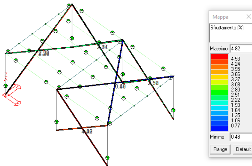
Figura 50: Sfruttamento (%) controventi.
