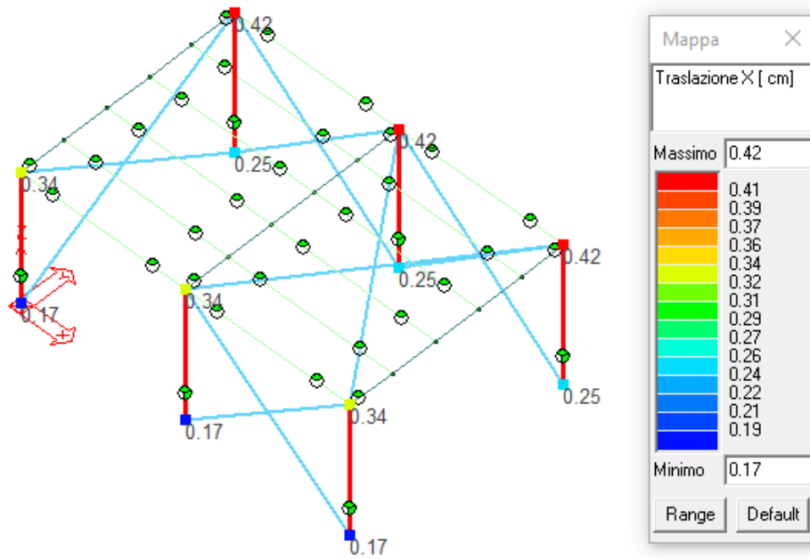
Figura 39: Massimi spostamenti in direzione X - SLE.
