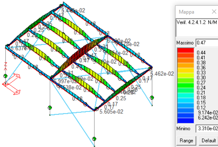
Figura 45: Verifica N/M travi.
