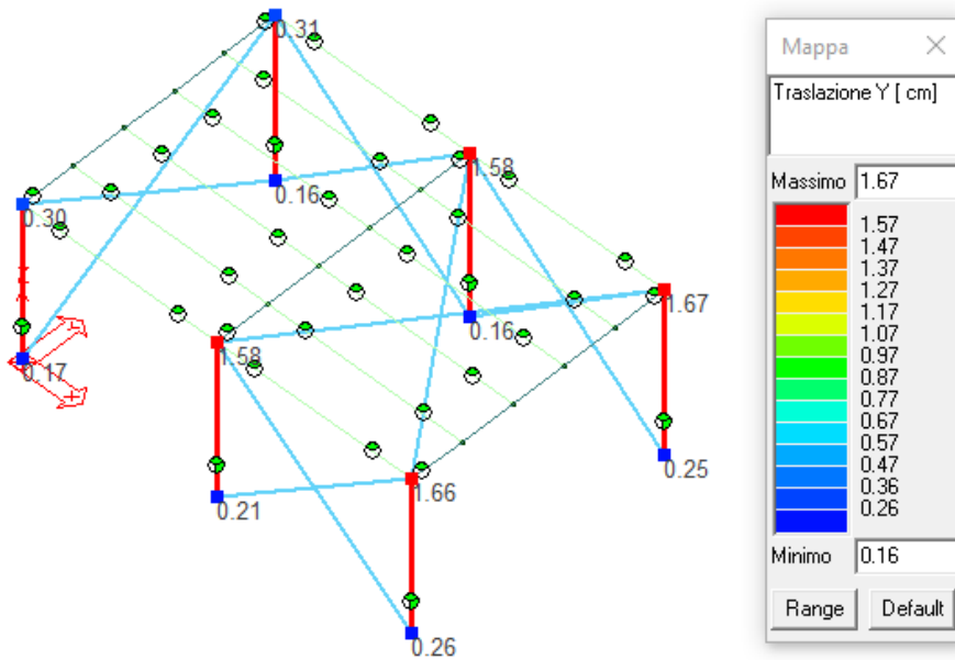
Figura 40: Massimi spostamenti in direzione Y - SLE.
