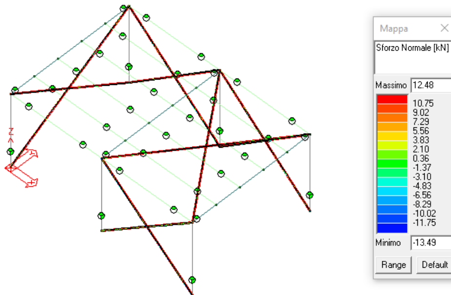
Figura 49: Azioni assiali (N) sui controventi.
