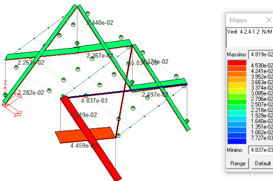
Figura 51: Verifica N/M controventi
