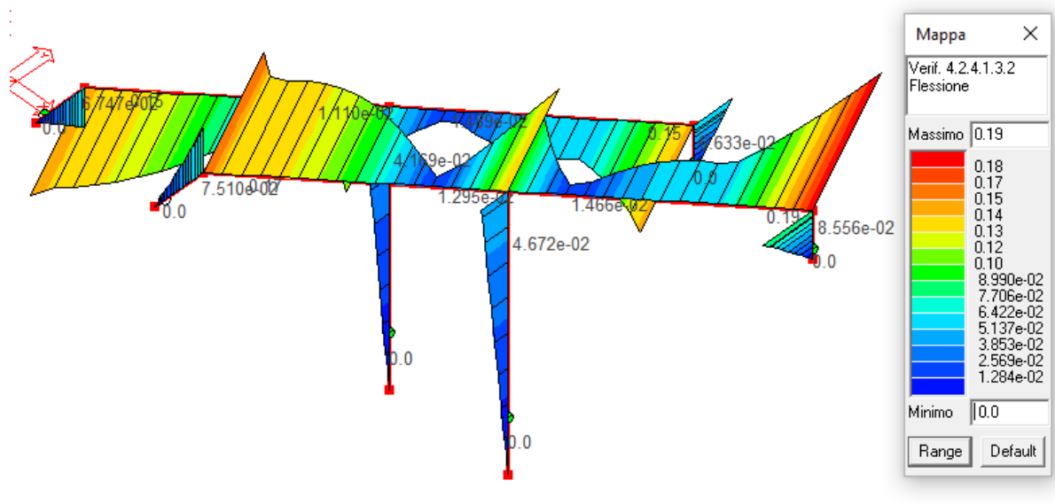
Figura 58: Verifica ad instabilità flessionale scala.
