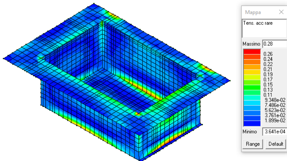
Figura 27: Verifica tensioni rare nell'acciaio.
