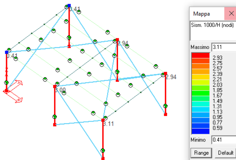
Figura 38: Verifica spostamenti interpiano orizzontale struttura di sostegno.
