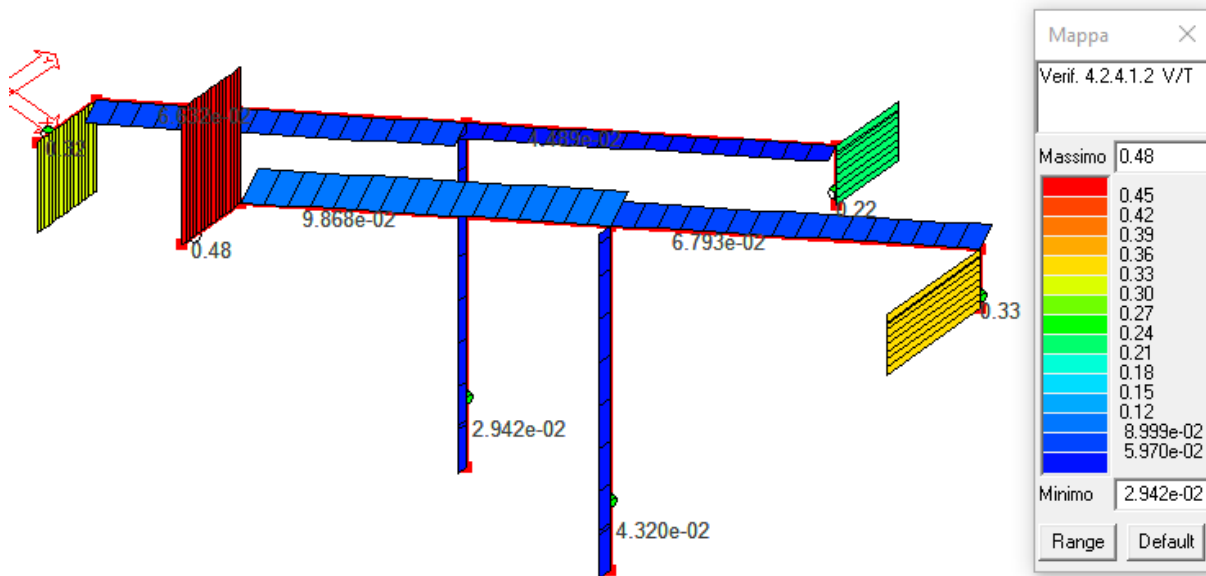
Figura 57: Verifica a taglio torsione scala.
