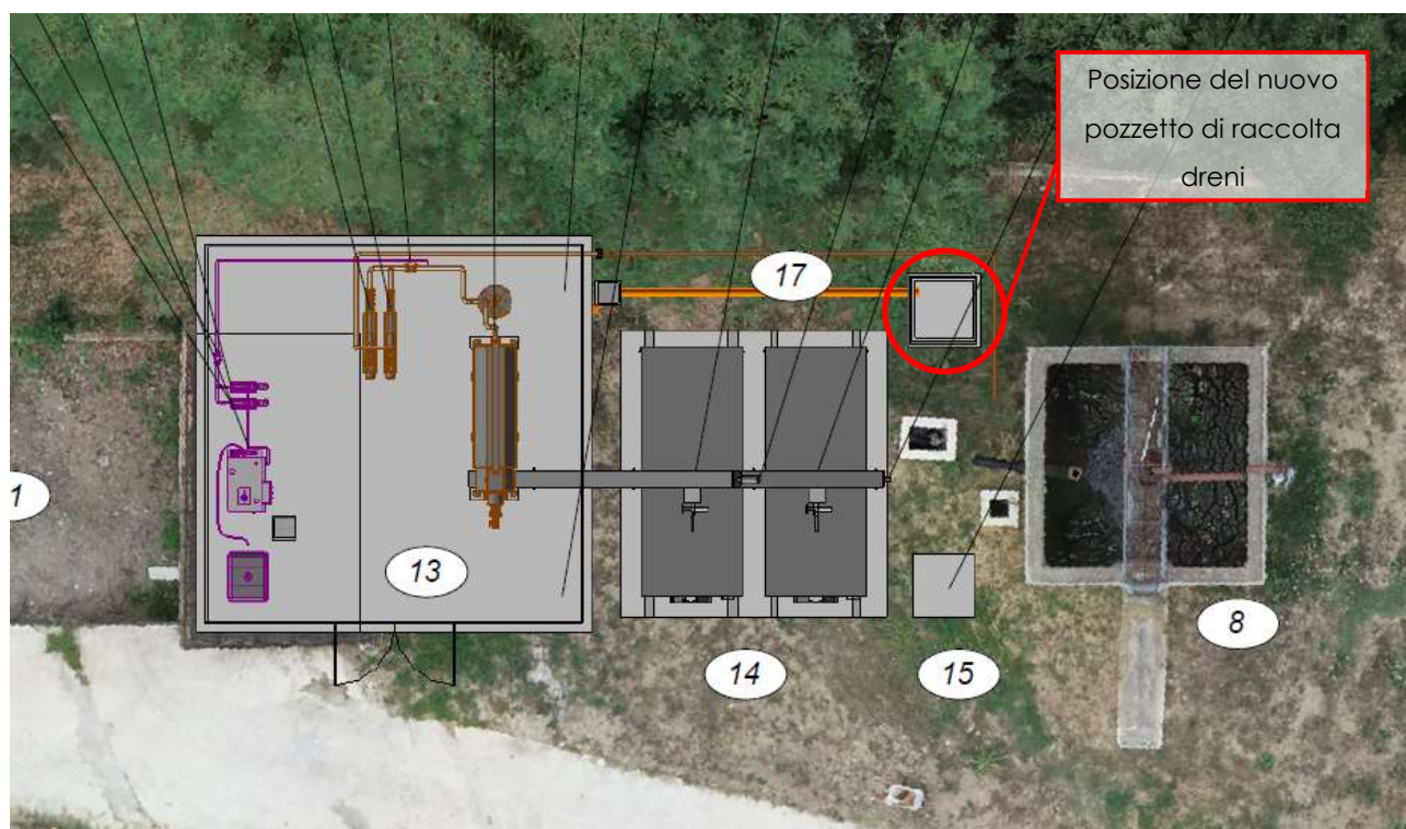
Figura 6: Risoluzione dell'interferenza superficiale nell'impianto di Ascea
