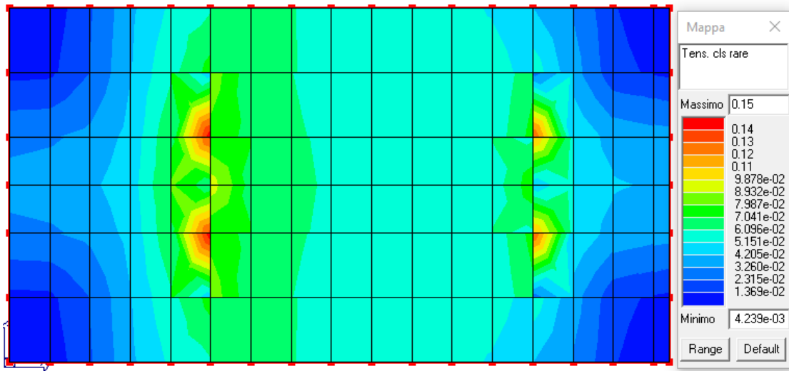
Figura 23: Verifica tensioni rare nel cls.
