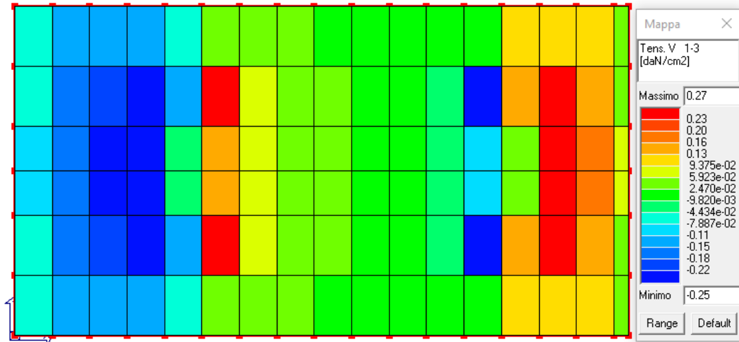
Figura 18: Tensioni di taglio 1-3 in daN/cm 2 .
