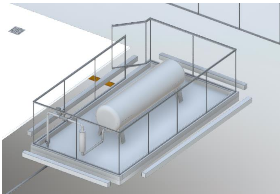
Figura 3: Estratto da modellazione BIM.
