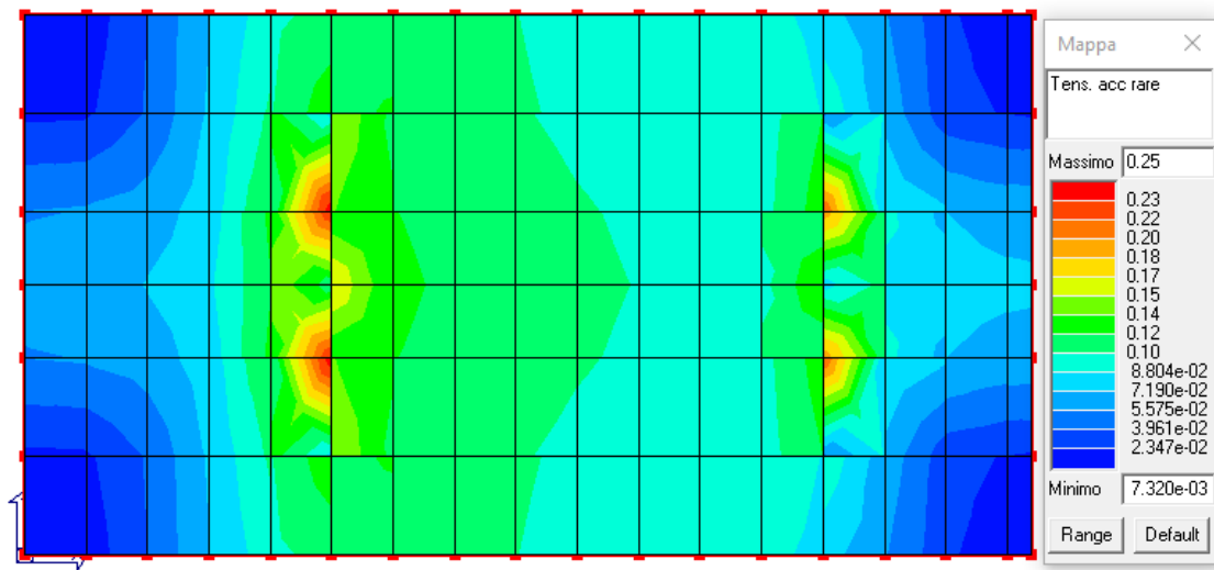
Figura 24: Verifica tensioni rare nell'acciaio.
