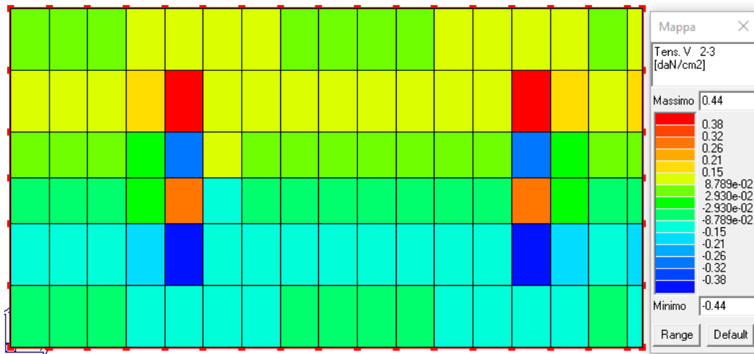
Figura 19: Tensioni di taglio 2-3 in daN/cm 2 .
