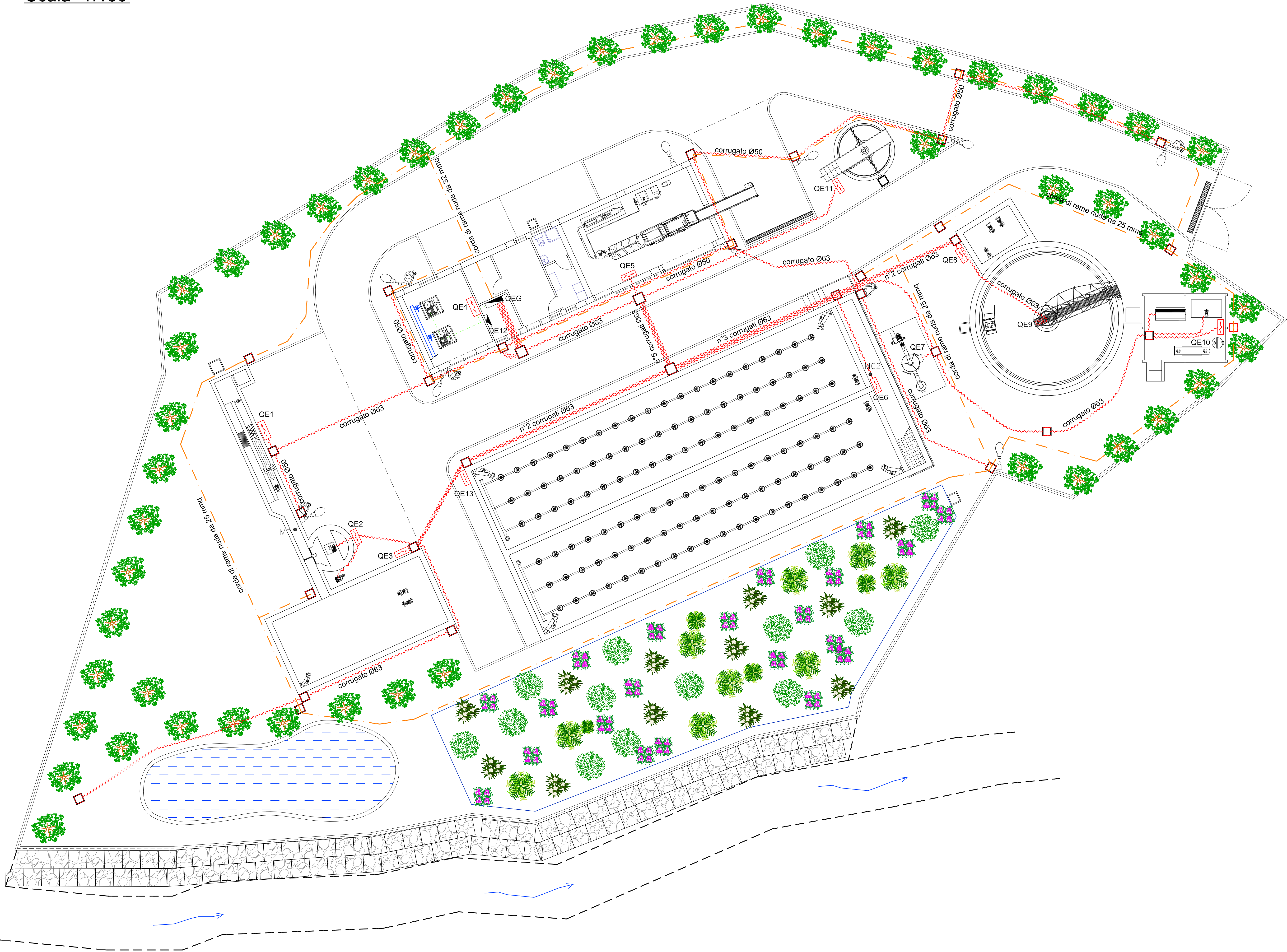
Planimetria generale Scala=1:100
