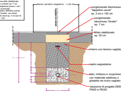
SEZIONE DI POSA TIPO SU CIGLIO BANCHINA STRADA COMUNALE
