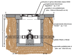
SEZIONE DI POSA TIPO SU STRADA COMUNALE ASFALTATA
