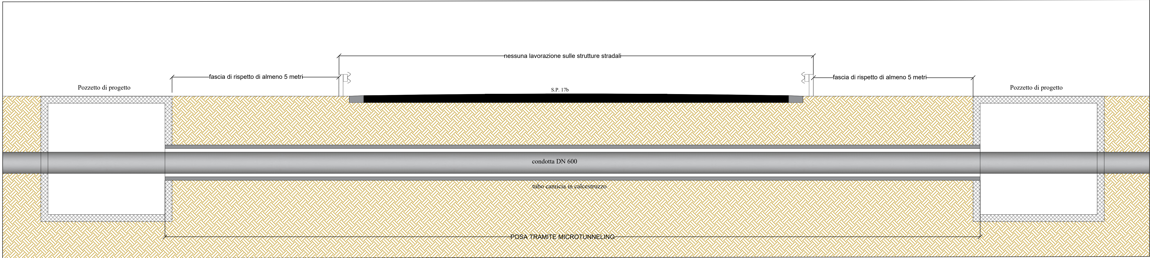
Sezione attraversamento trasversale - Stato di Progetto; scala 1:50
