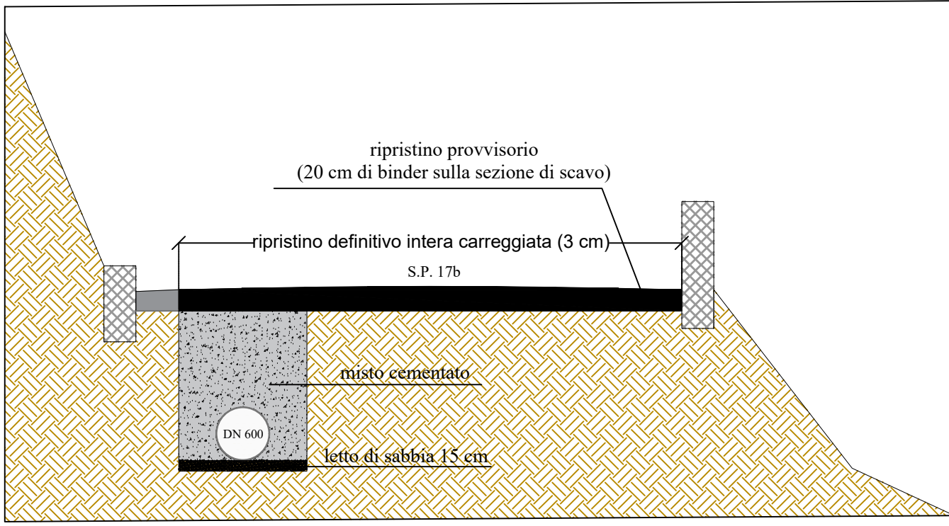
Sezione tipo 3 - Stato di Progetto; scala 1:50
