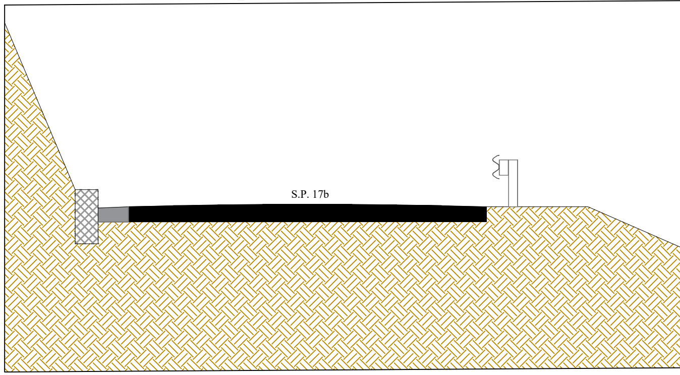
Sezione tipo 2 - Stato di Fatto; scala 1:50
