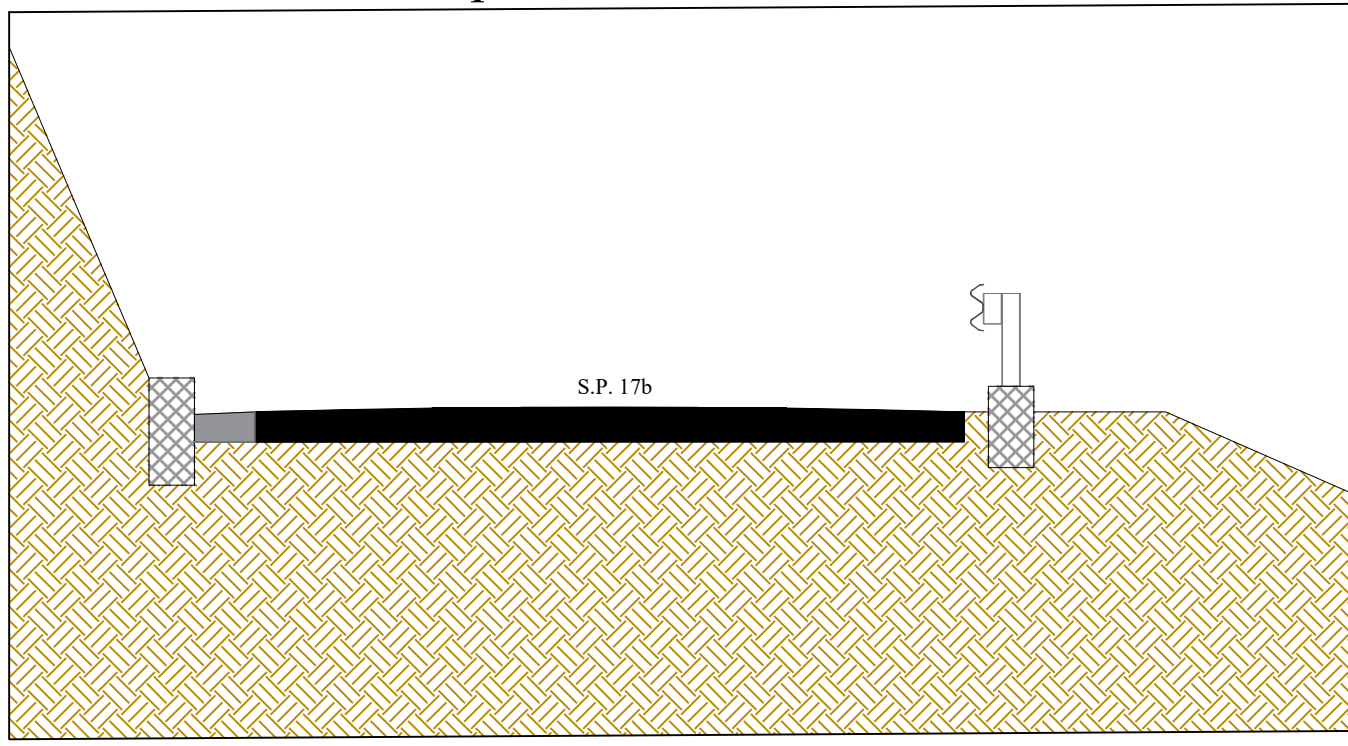
Sezione tipo 1 - Stato di Fatto; scala 1:50
