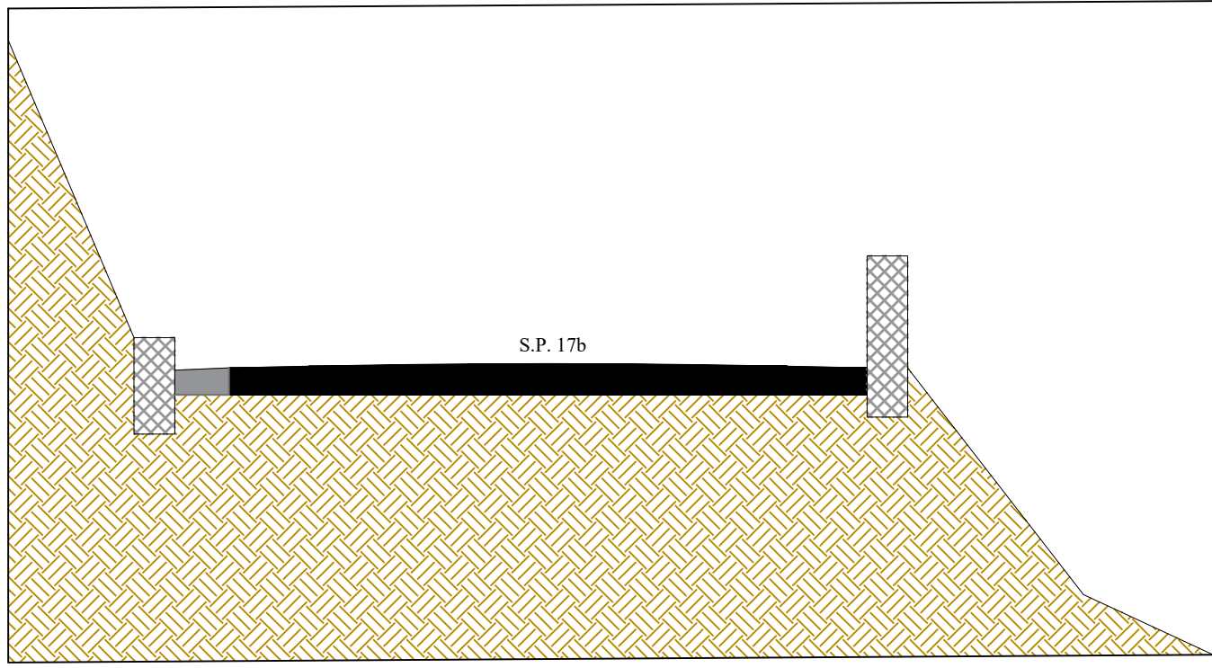
Sezione tipo 3 - Stato di Fatto; scala 1:50
