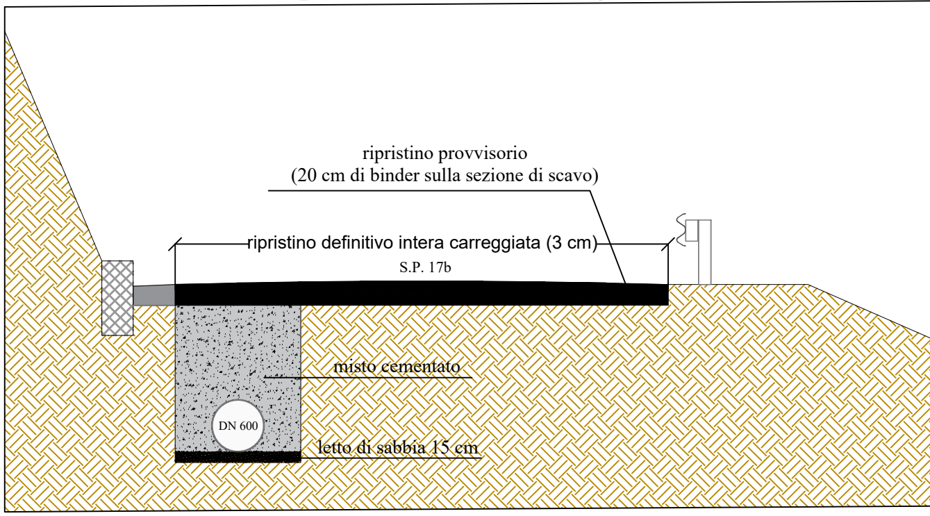
Sezione tipo 2 - Stato di Progetto; scala 1:50
