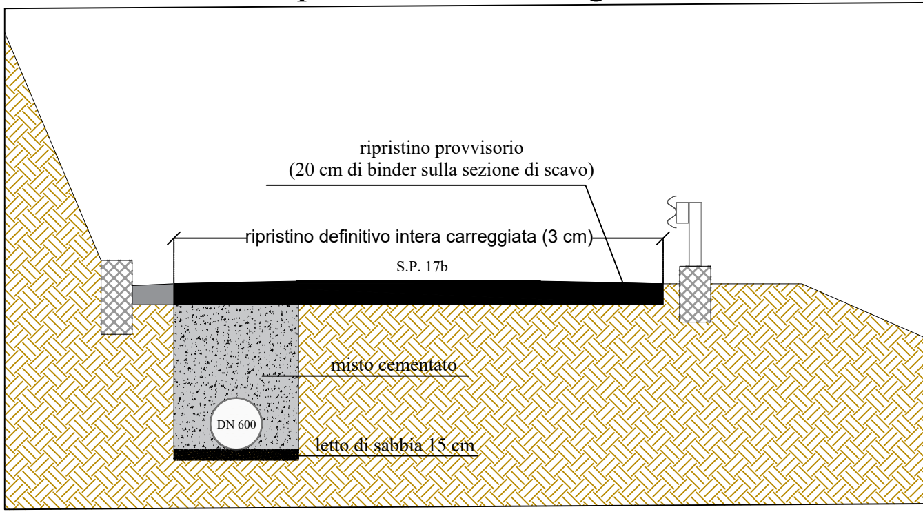
Sezione tipo 1 - Stato di Progetto; scala 1:50
