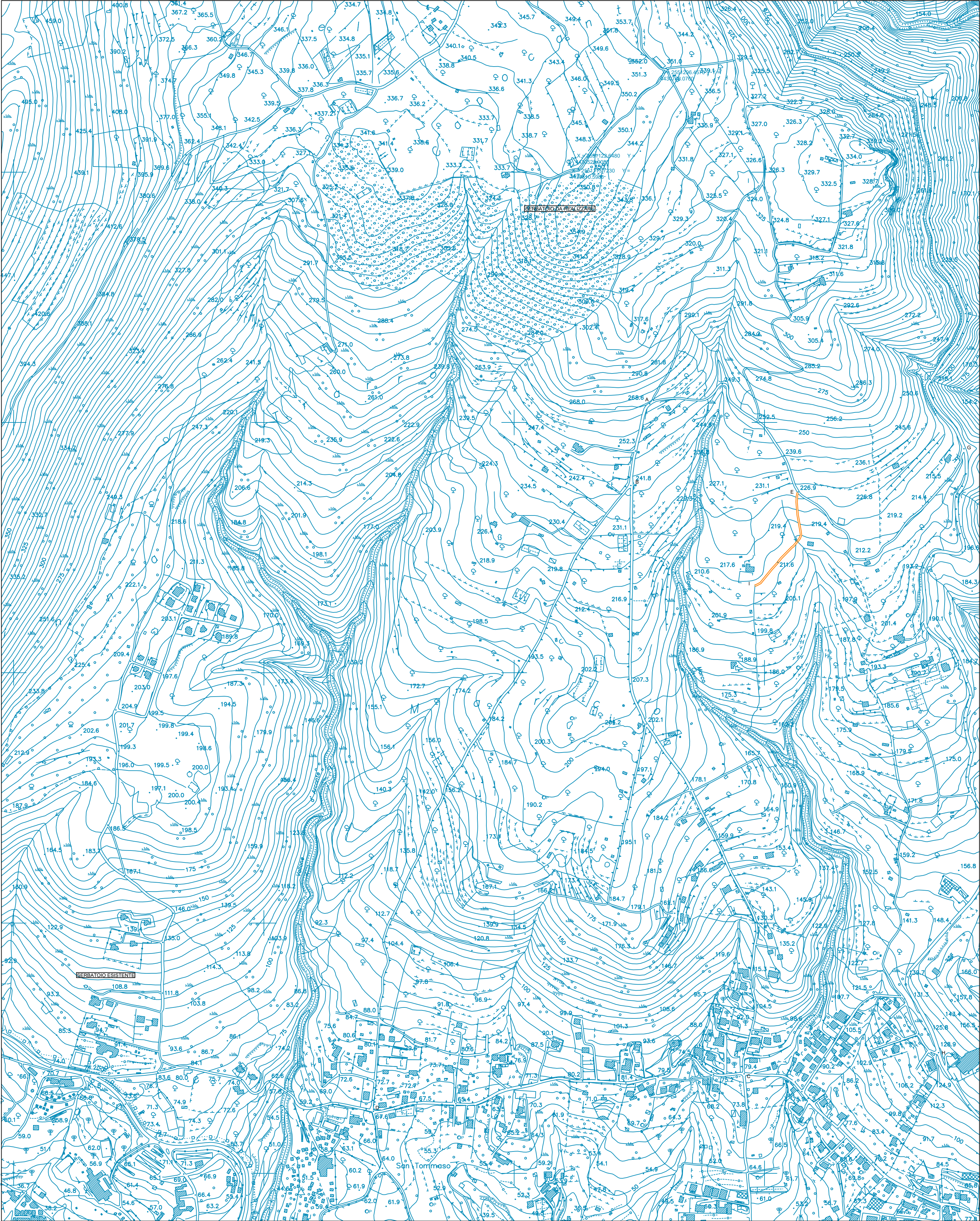
- Stralcio Aerofotogrammetrico - - Scala 1:5000 -
