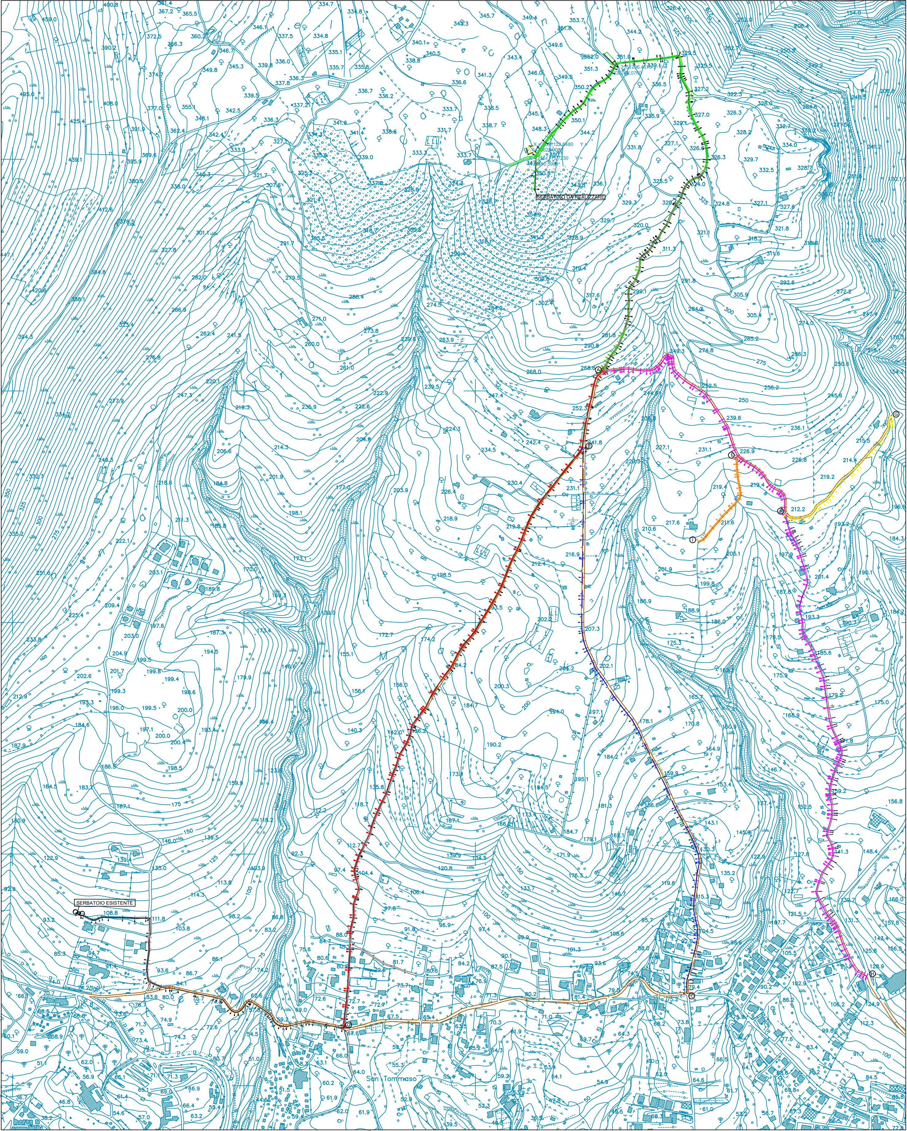
- Stralcio Aerofotogrammetrico - - Con Posizionamento - - Scala 1:5000 -
