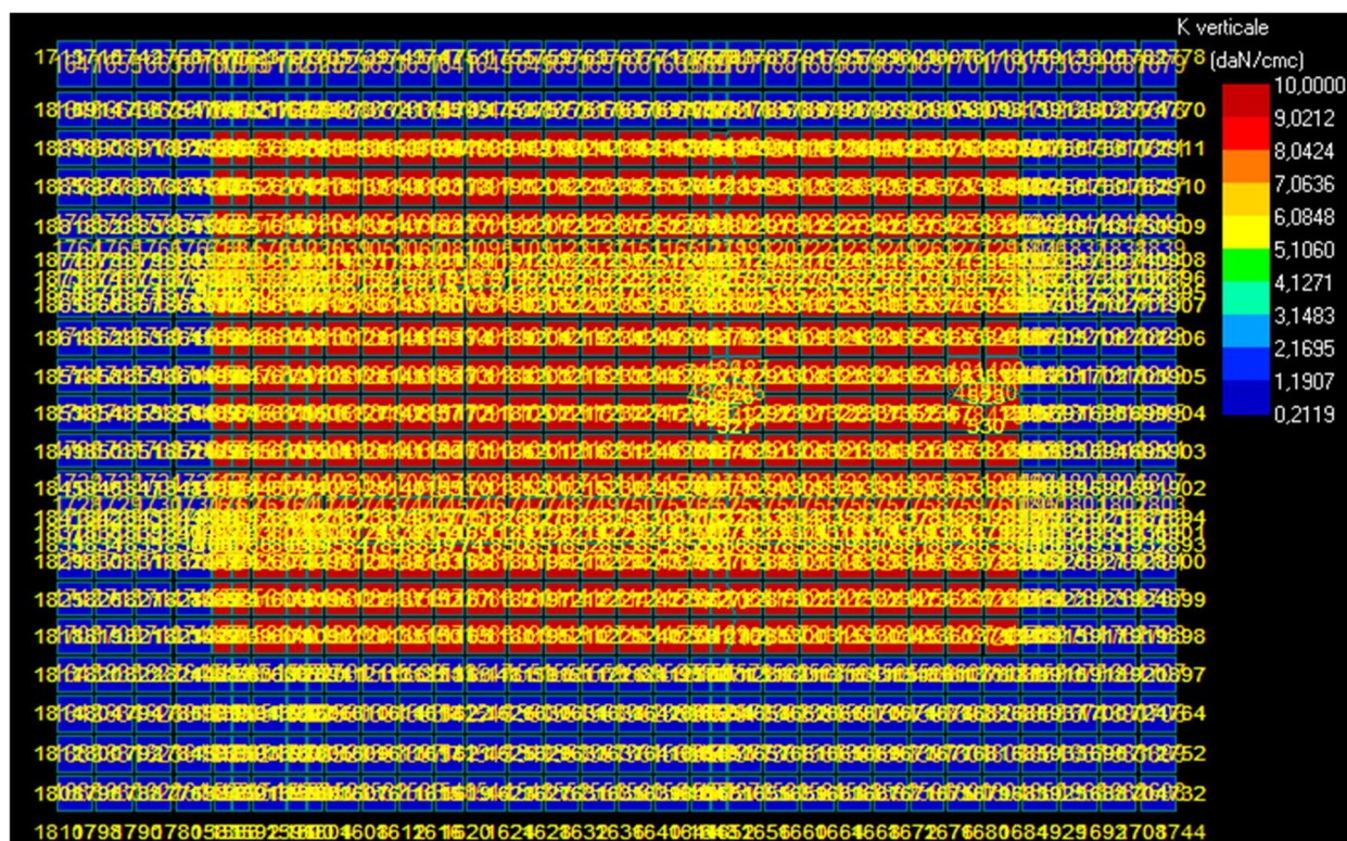
Figura 4: Costante di Winkler – stratigrafia 2.
