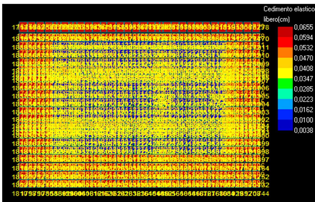
Figura 9: Cedimento - Stratigrafia 2.
