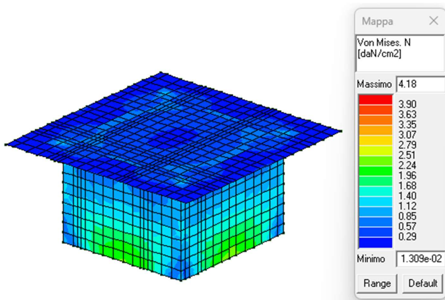
Figura 19: Tensioni di membrana (N) tramite formulazione di Von Mises.
