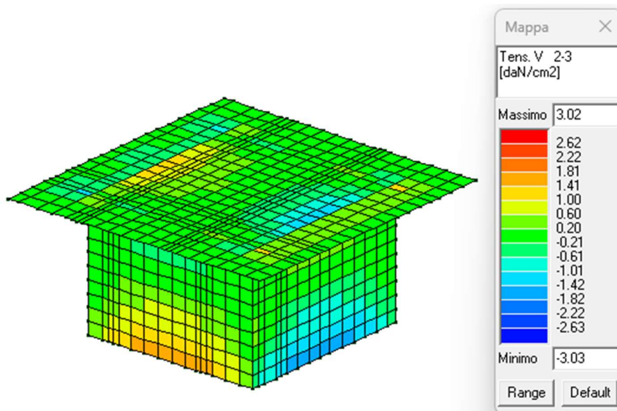
Figura 22: Tensioni di taglio 2-3 in daN/cm 2 .
