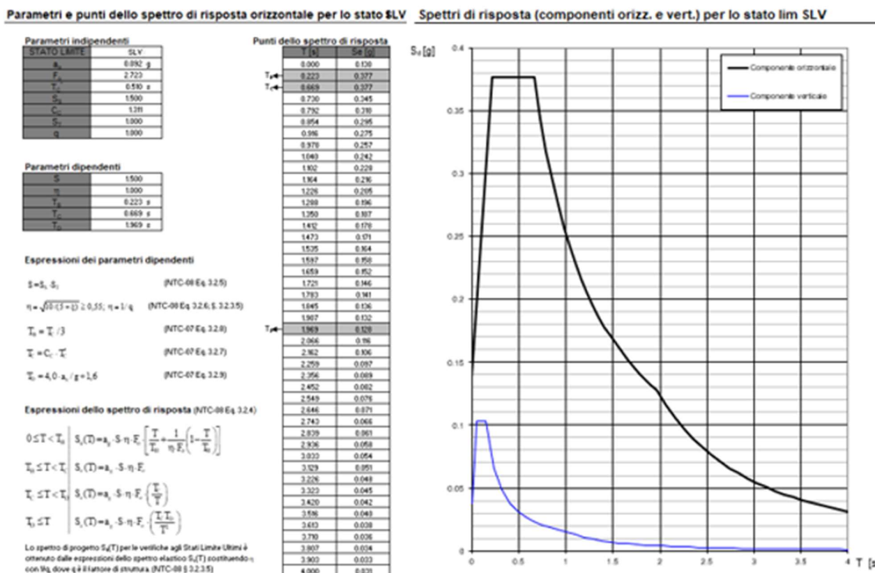
Figura 16: Parametri spettro di risposta SLV.
