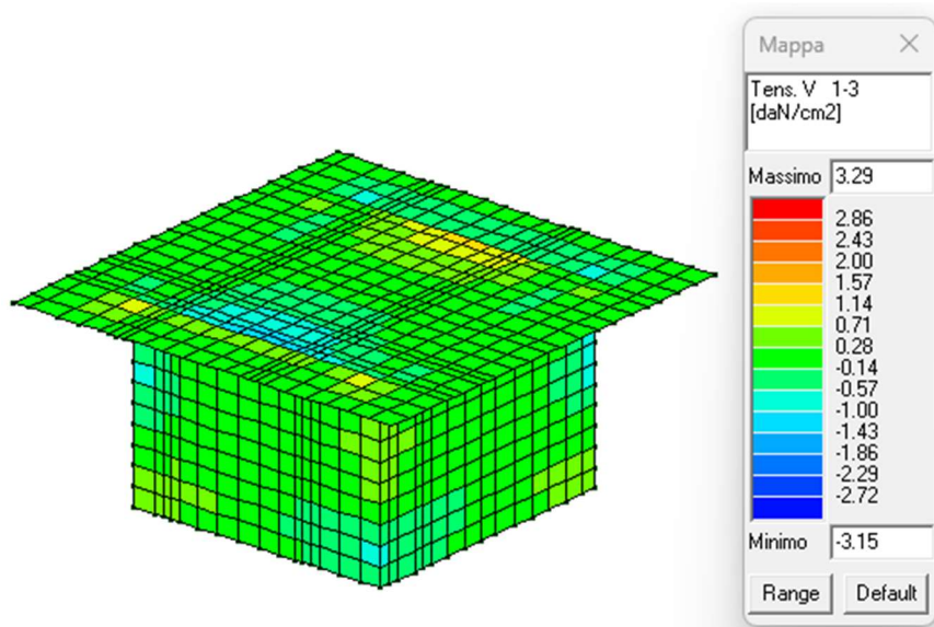
Figura 21: Tensioni di taglio 1-3 in daN/cm 2 .
