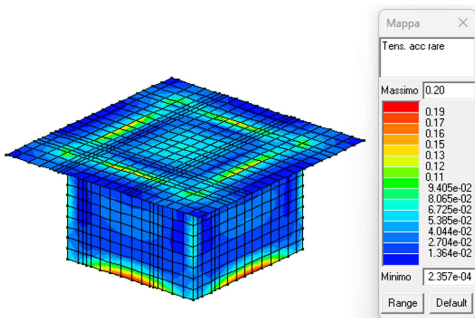
Figura 27: Verifica tensioni rare nell'acciaio.
