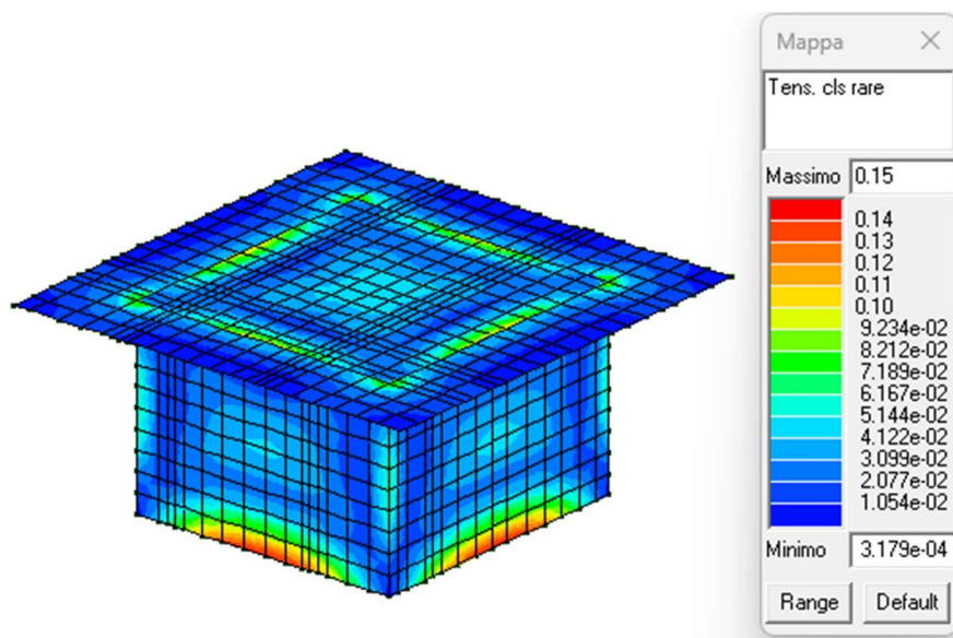
Figura 26: Verifica tensioni rare nel cls.
