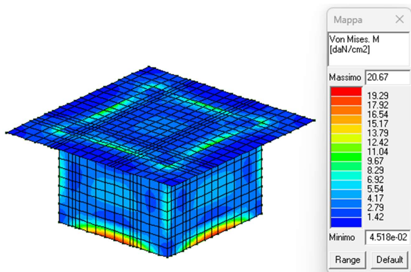
Figura 20: Tensioni di flessione (M) tramite formulazione di Von Mises.
