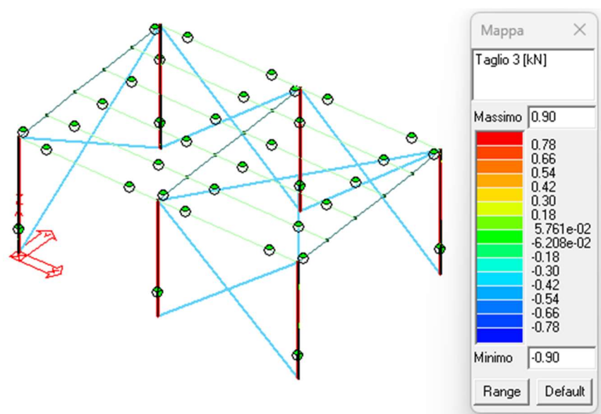
Figura 30: Azioni di taglio V3-3 (N) sulle colonne.
