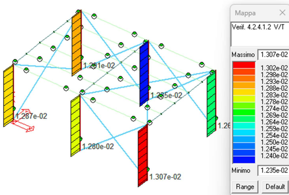
Figura 35: Verifica a taglio torsione colonne.
