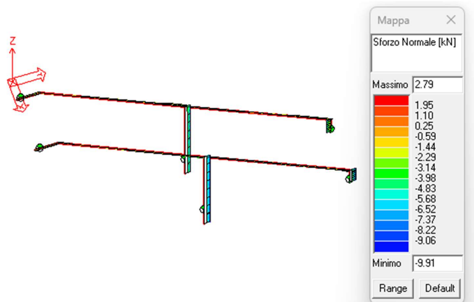
Figura 52: Azioni assiali (N) sulle travi.
