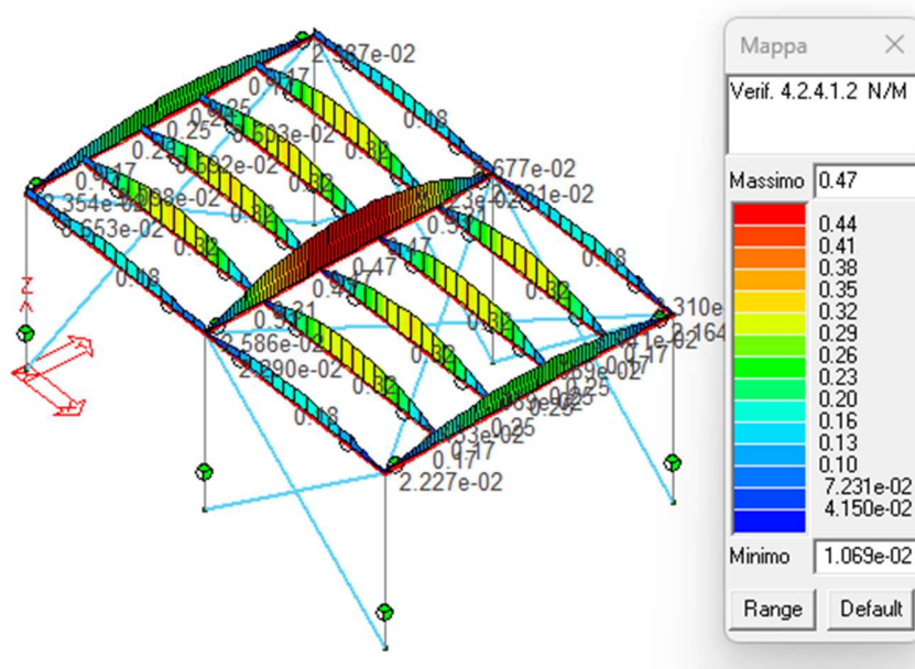
Figura 45: Verifica N/M travi.
