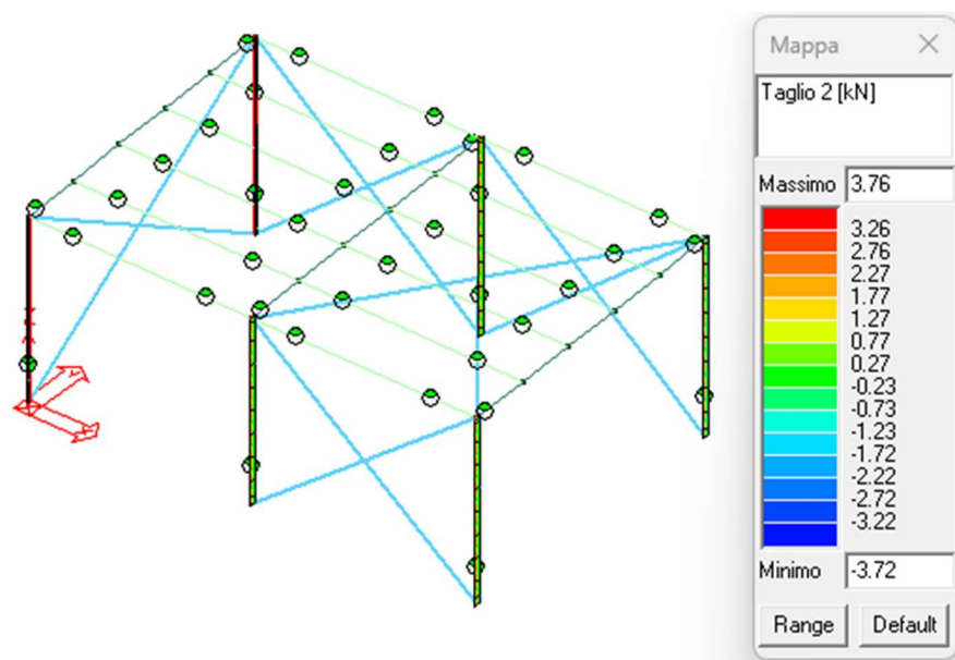
Figura 29: Azioni di taglio V2-2 (N) sulle colonne.
