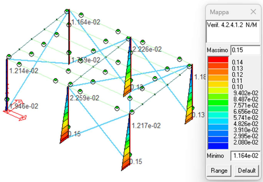
Figura 34: Verifica N/M colonne.
