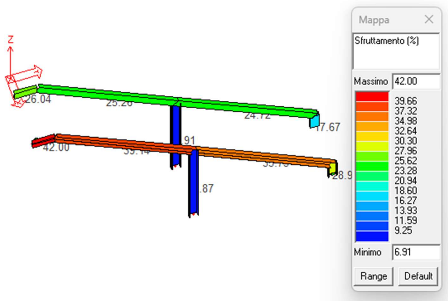
Figura 55: Sfruttamento (%) scala.
