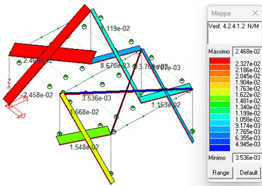
Figura 51: Verifica N/M controventi
