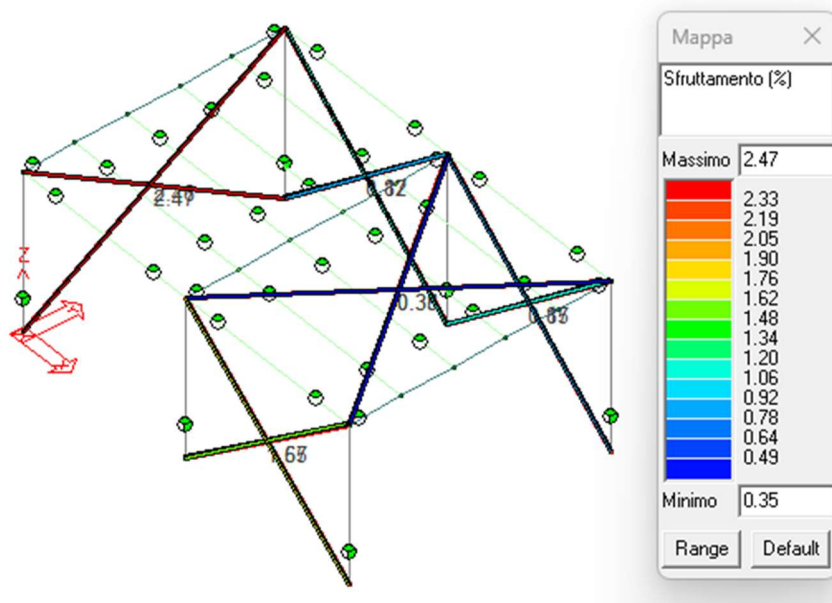
Figura 50: Sfruttamento (%) controventi.
