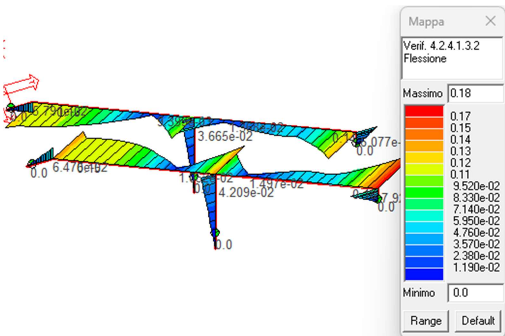
Figura 58: Verifica ad instabilità flessionale scala.
