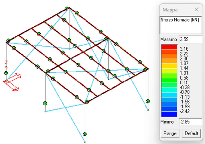
Figura 41: Azioni assiali (N) sulle travi.
