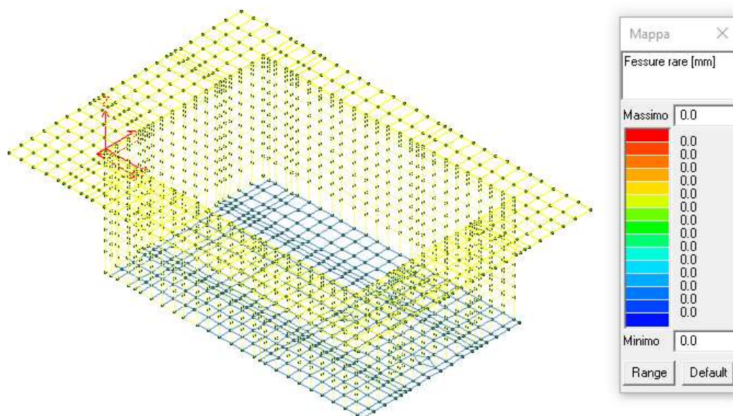
Figura 25: Fessure nel cls.
