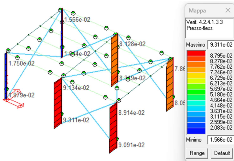
Figura 36: Verifica ad instabilità presso-flessionale colonne.
