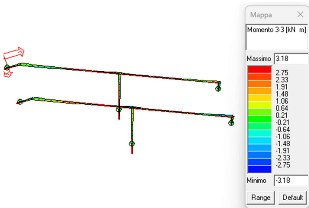
Figura 54: Azioni di taglio M3-3 (N) scala.
