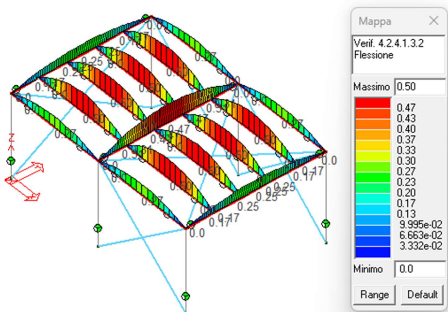
Figura 47: Verifica ad instabilità flessionale travi.
