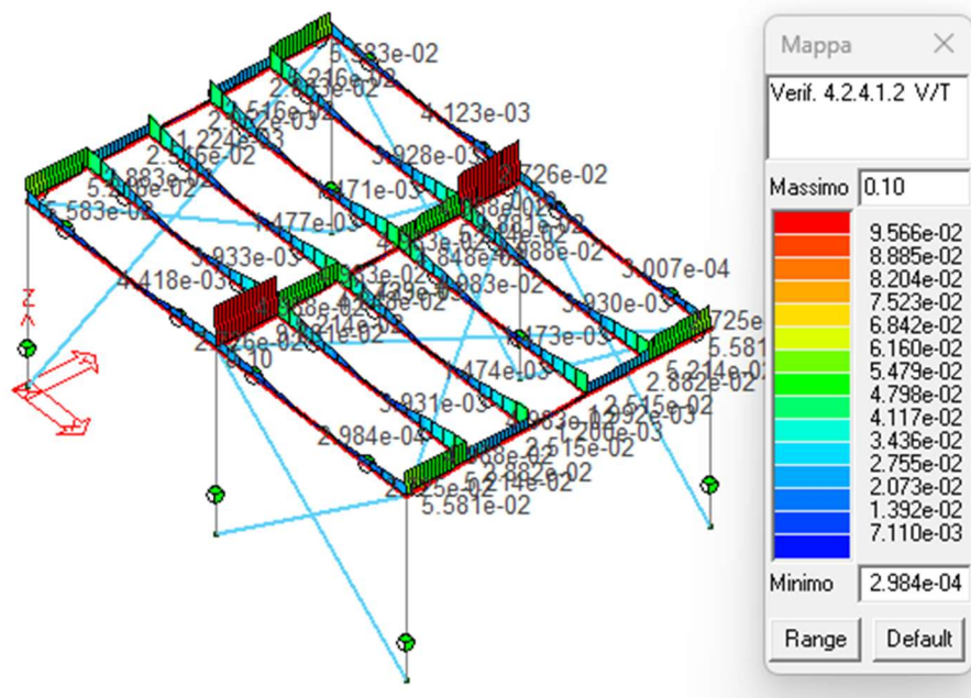
Figura 46: Verifica a taglio torsione travi.
