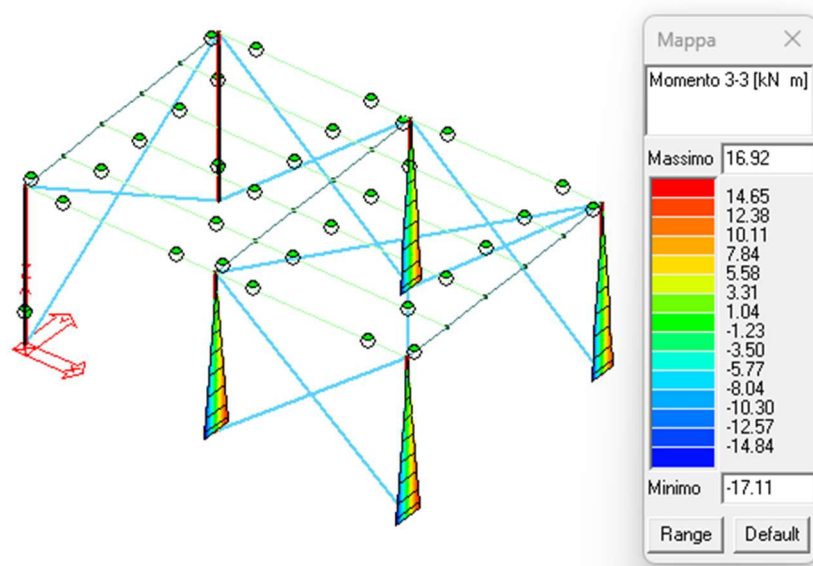
Figura 32: Azioni di taglio M3-3 (N) sulle colonne
