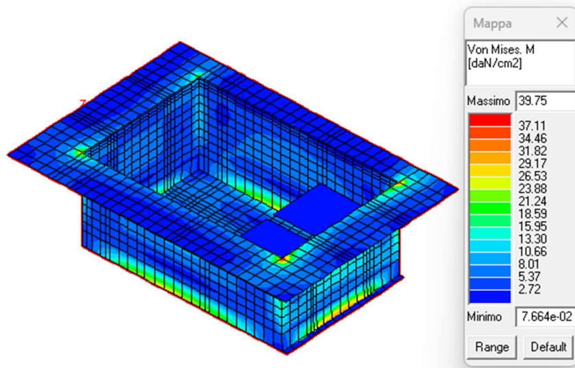
Figura 20: Tensioni di flessione (M) tramite formulazione di Von Mises.
