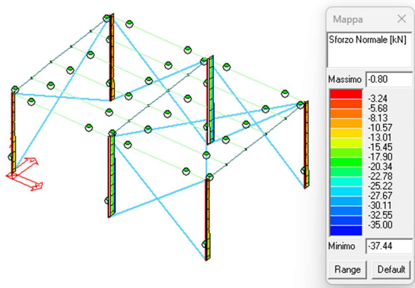
Figura 28: Azioni assiali (N) sulle colonne.
