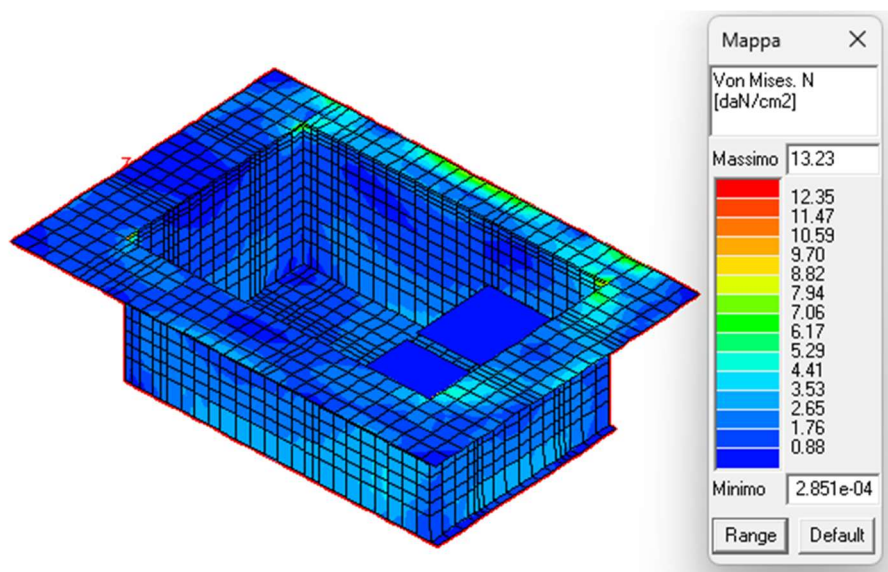
Figura 19: Tensioni di membrana (N) tramite formulazione di Von Mises.
