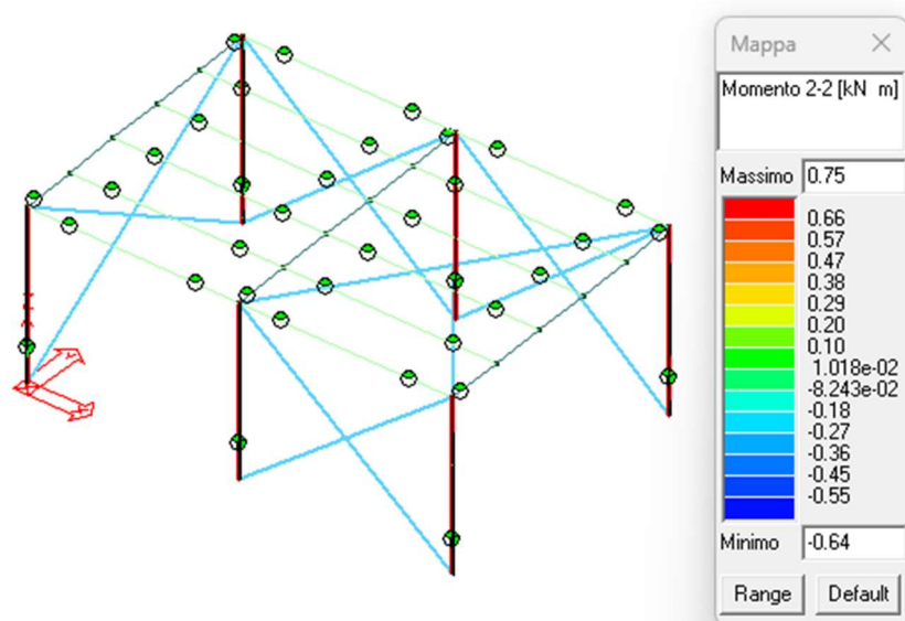
Figura 31: Azioni di taglio M2-2 (N) sulle colonne.
