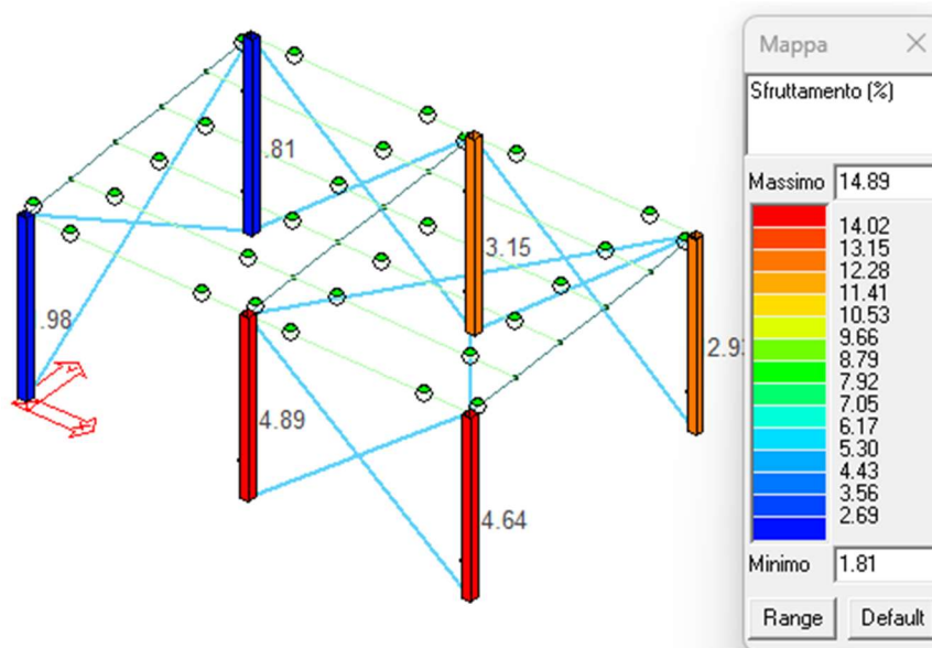
Figura 33: Sfruttamento (%) colonne.
