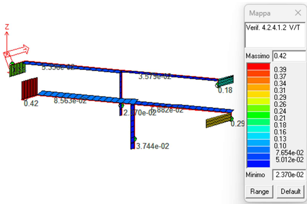
Figura 57: Verifica a taglio torsione scala.
