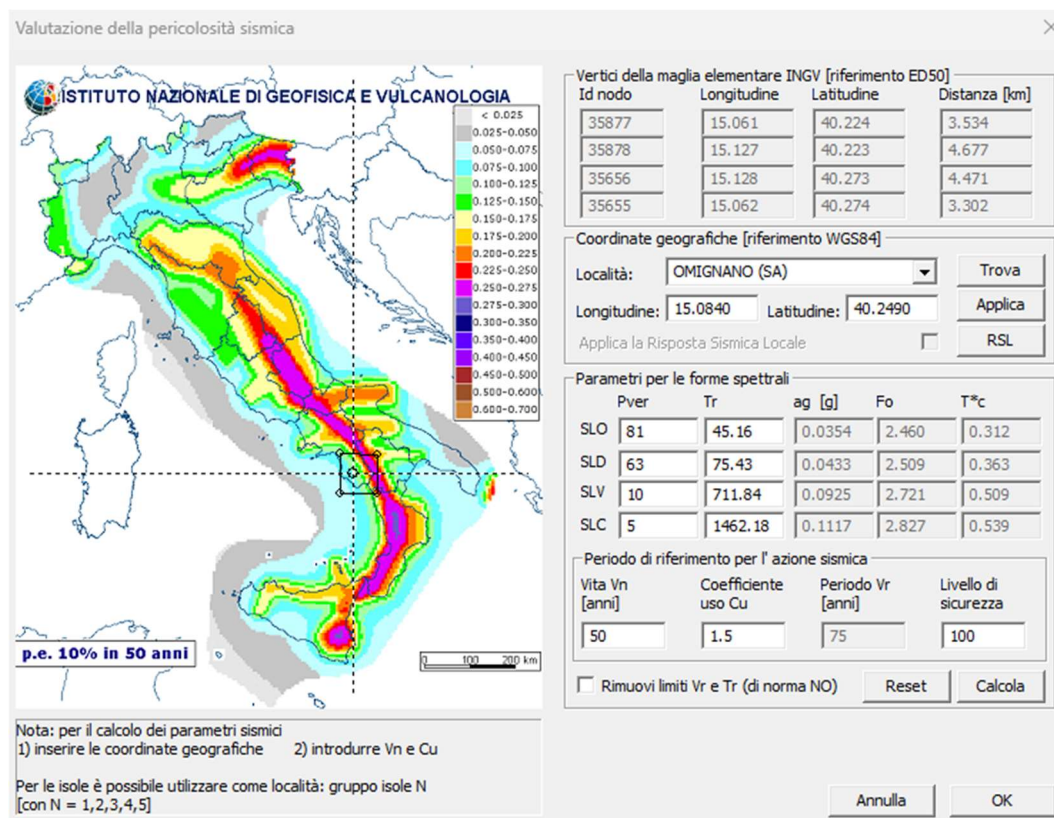
Figura 7: Valutazione della pericolosità sismica.
