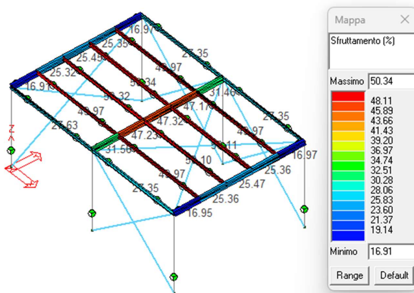
Figura 44: Sfruttamento (%) travi.
