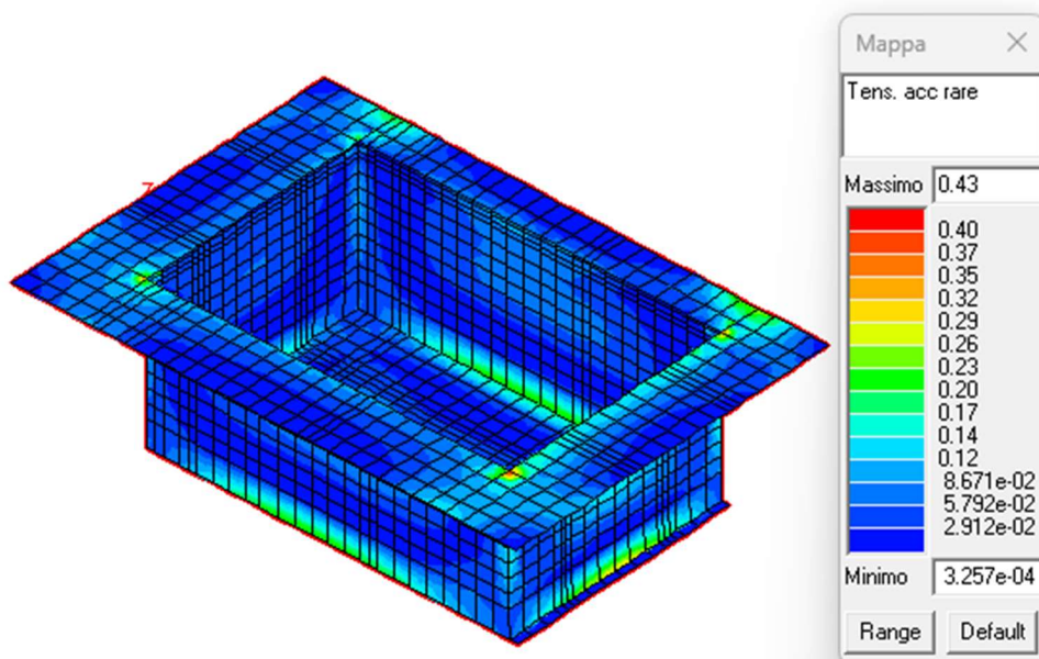
Figura 27: Verifica tensioni rare nell'acciaio.
