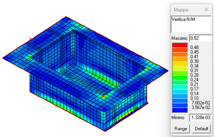
Figura 23: Verifica N/M
