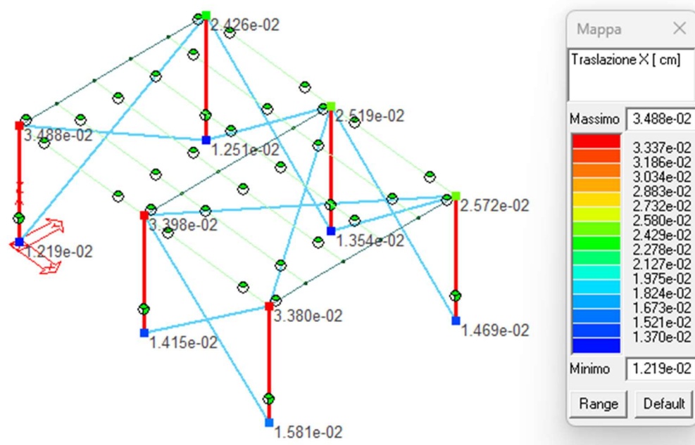
Figura 39: Massimi spostamenti in direzione X - SLE.
