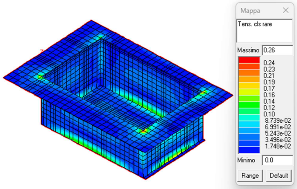
Figura 26: Verifica tensioni rare nel cls.
