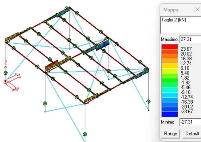
Figura 42: Azioni di taglio V2-2 (N) sulle travi.
