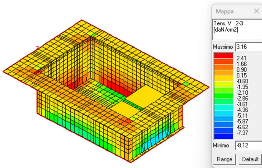
Figura 22: Tensioni di taglio 2-3 in daN/cm 2 .
