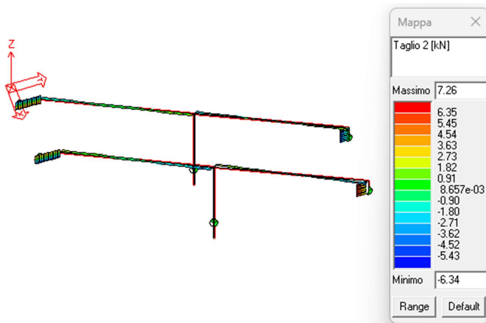
Figura 53: Azioni di taglio V2-2 (N) sulle travi.
