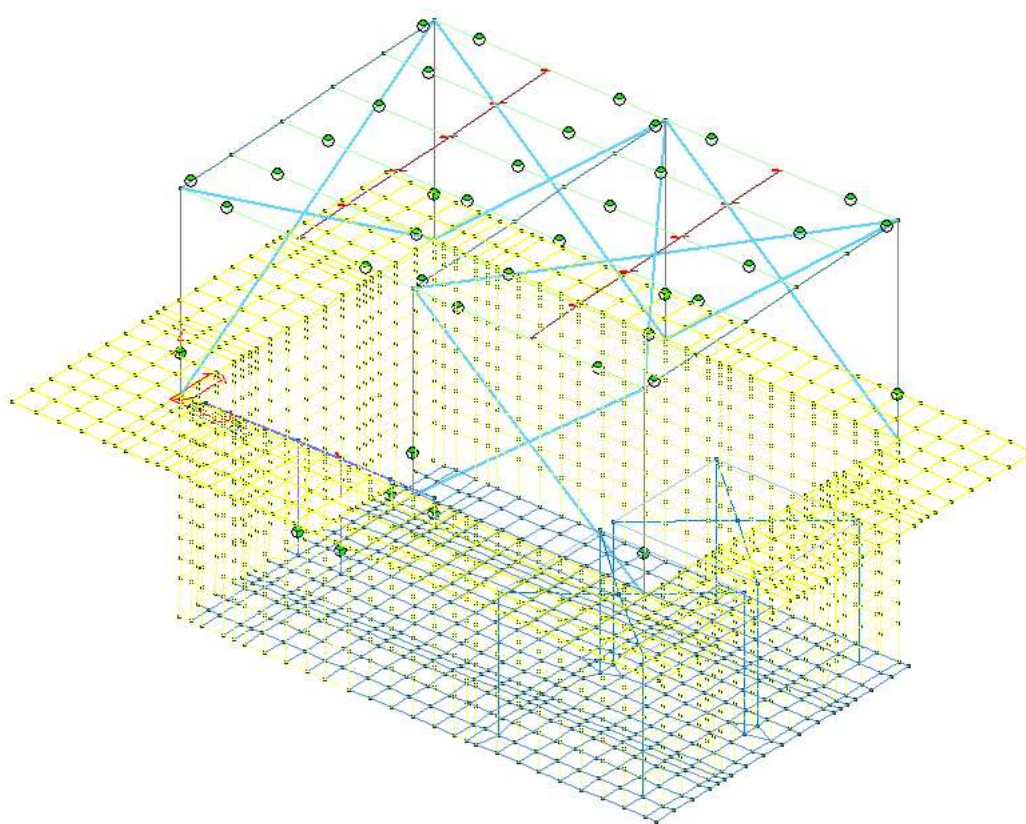
Figura 18: Vista complessiva del modello di calcolo
