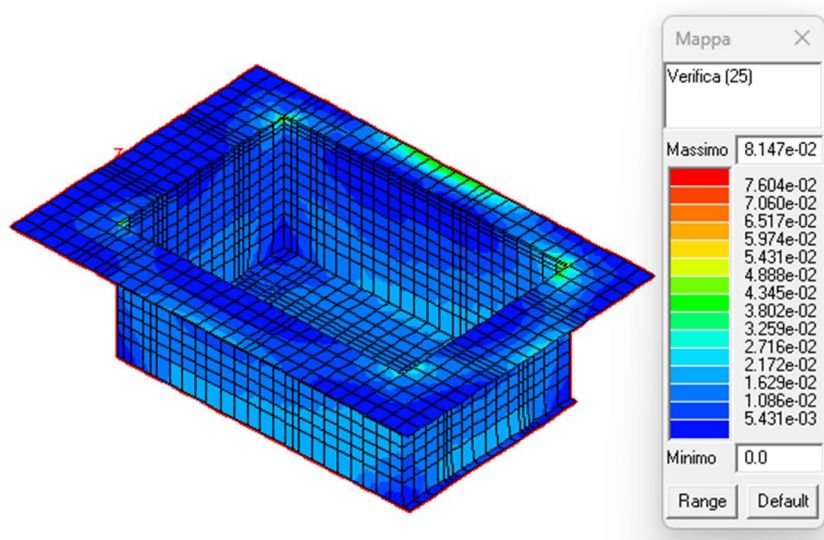
Figura 24: Verifica 25
