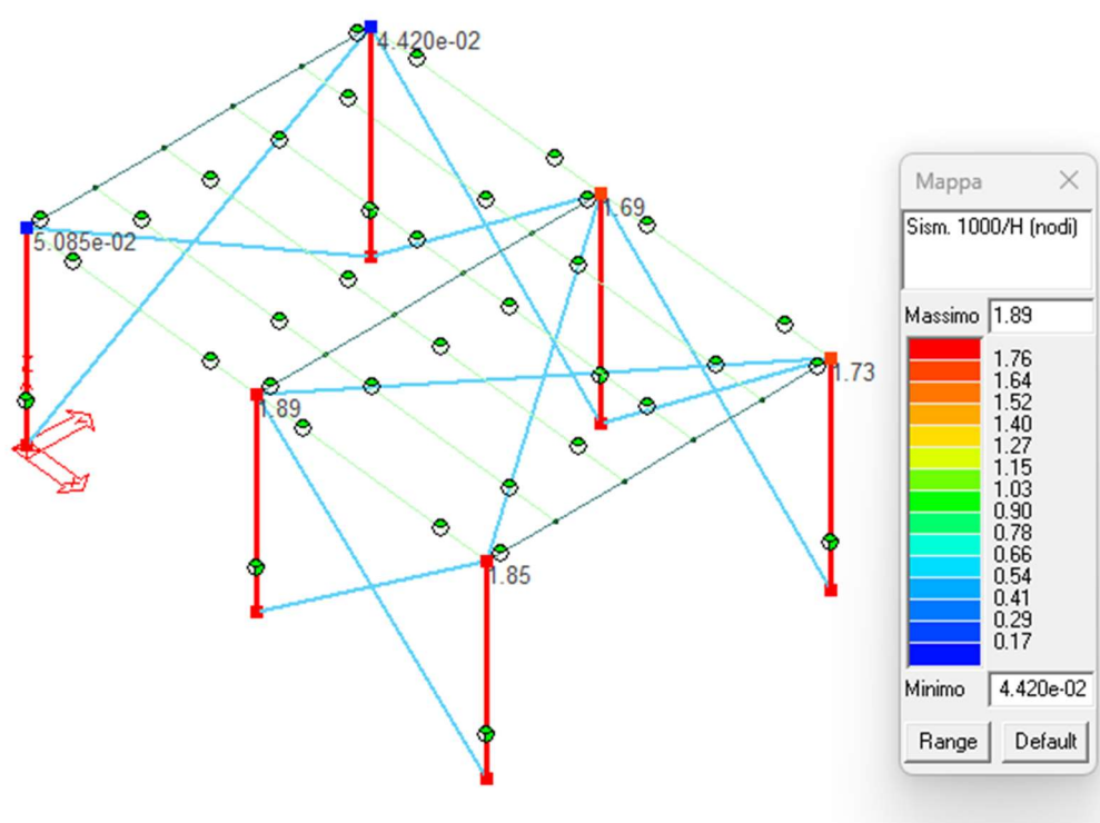
Figura 38: Verifica spostamenti interpiano orizzontale struttura di sostegno.
