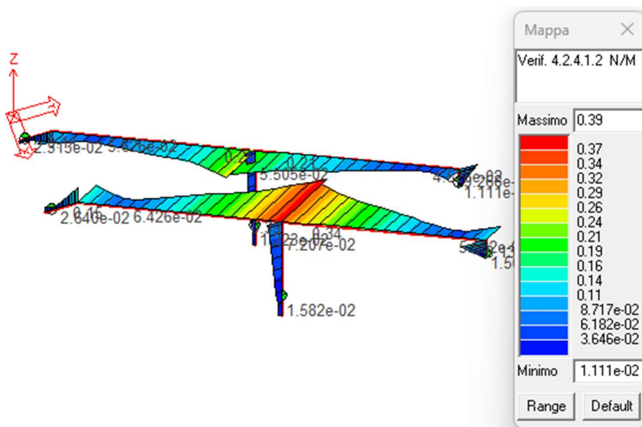
Figura 56: Verifica N/M scala.
