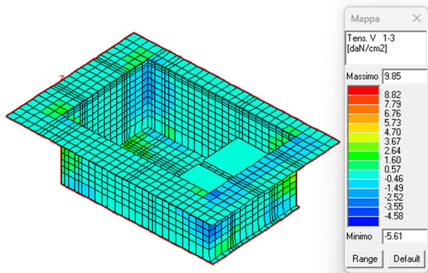
Figura 21: Tensioni di taglio 1-3 in daN/cm 2 .
