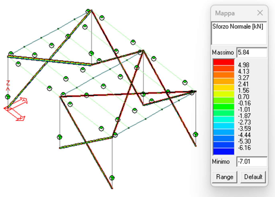
Figura 49: Azioni assiali (N) sui controventi.
