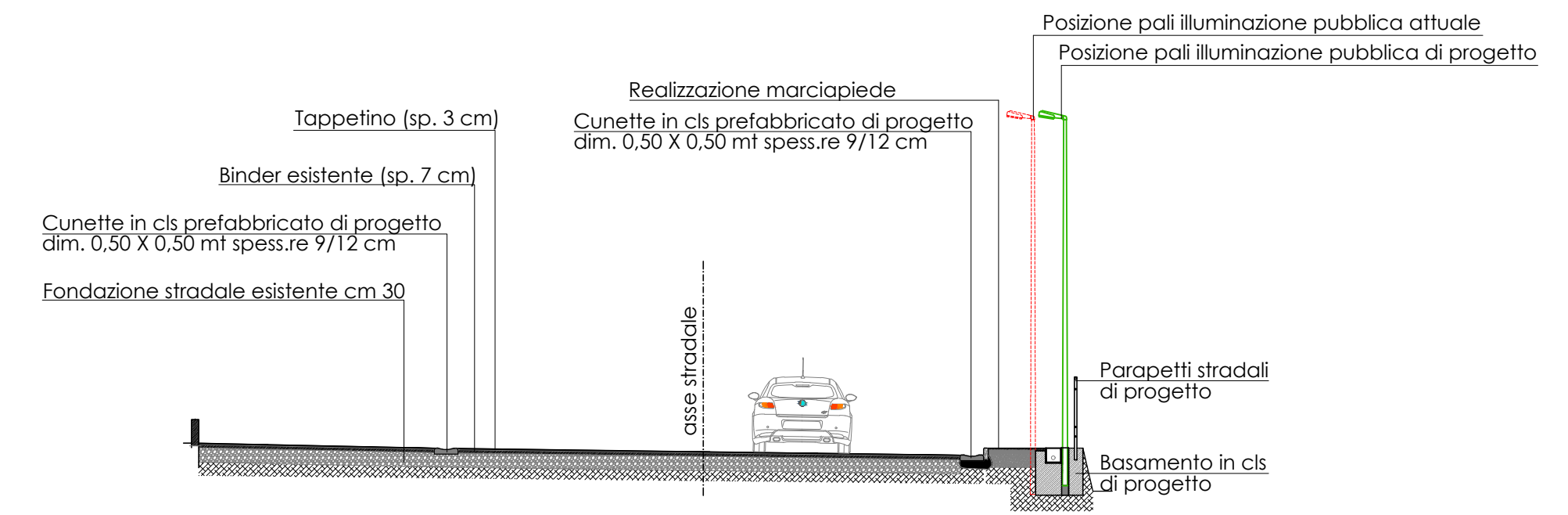
Sezione 1 scala 1:100
