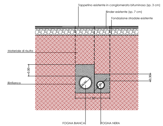
SCHEMA TIPO SEZIONE DI POSA STRADALE STATO DI FATTO
