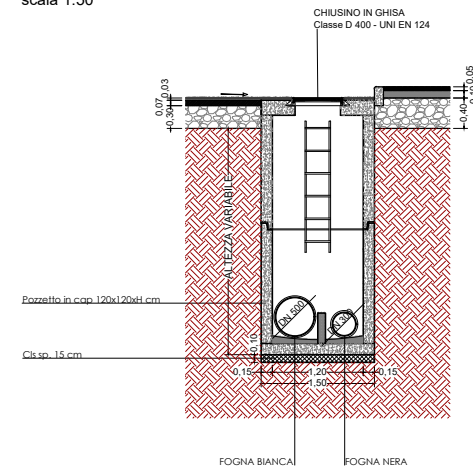
SEZIONE A - A POZZETTO STATO DI FATTO scala 1:50
