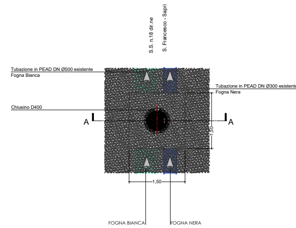
PIANTA POZZETTO STATO DI FATTO scala 1:50
