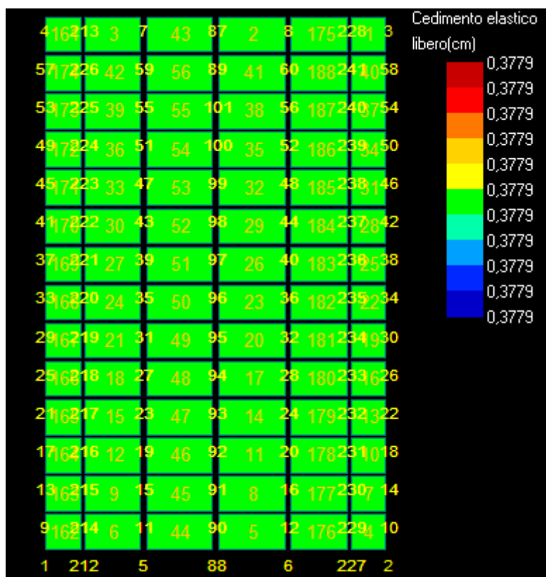
Figura 15: Cedimento - Stratigrafia 1.
