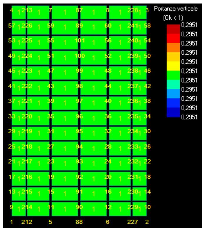
Figura 11: Portata – carico limite - Stratigrafia 1.
