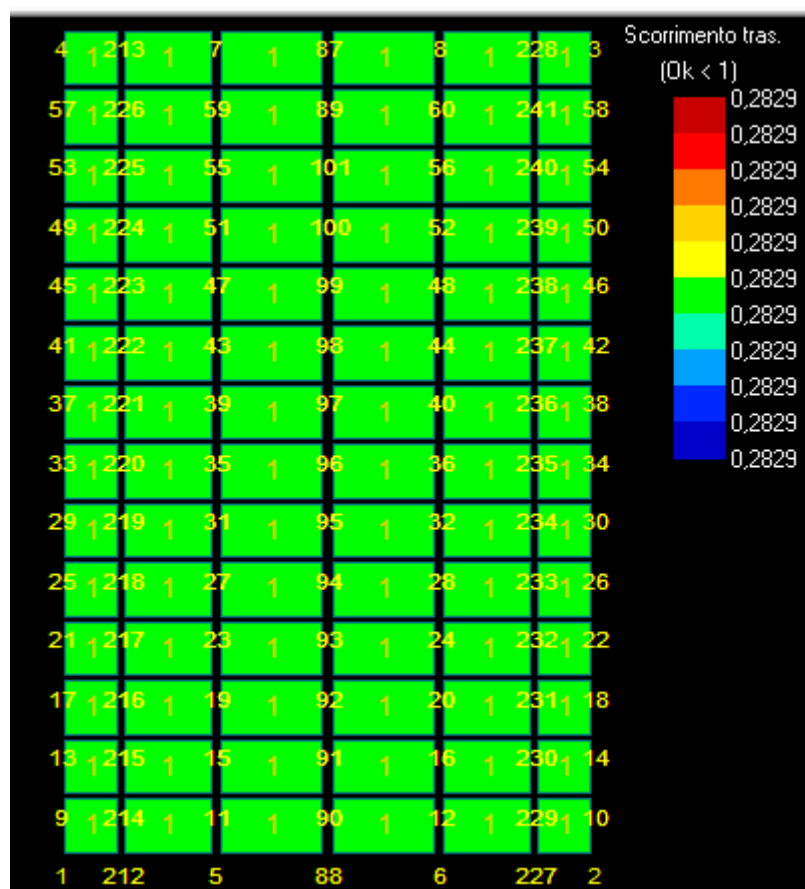
Figura 14: Scorrimento - Stratigrafia 2.
