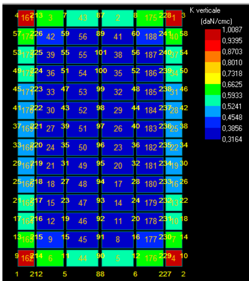
Figura 8: Costante di Winkler – stratigrafia 2.
