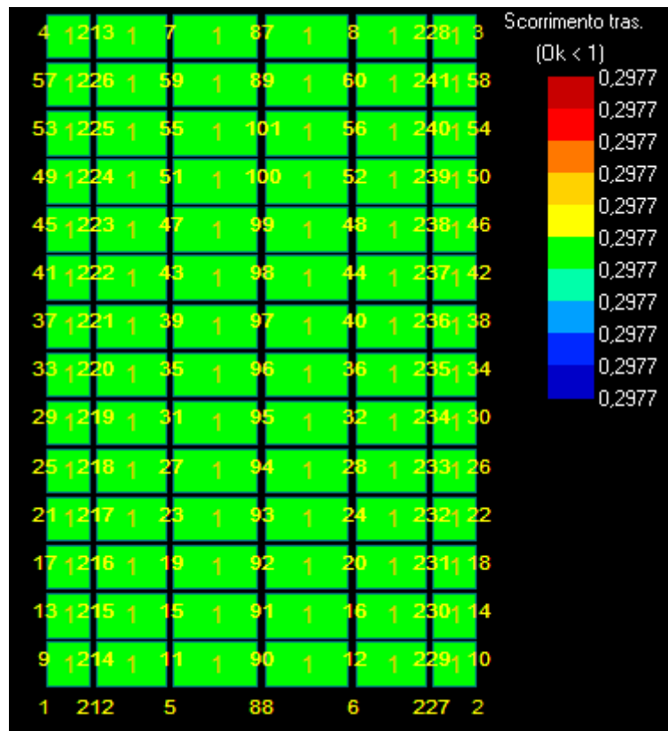
Figura 13: Scorrimento - Stratigrafia 1.
