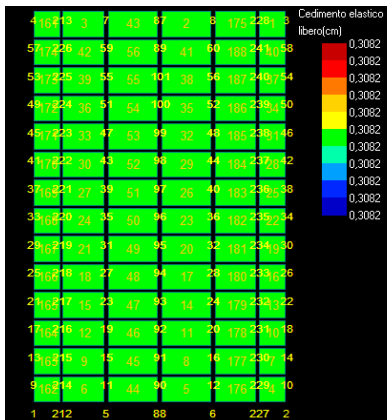
Figura 16: Cedimento - Stratigrafia 2.
