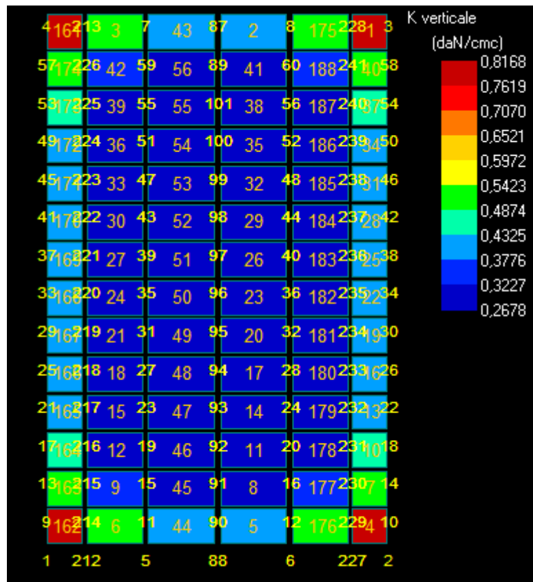
Figura 7: Costante di Winkler – stratigrafia 1.
