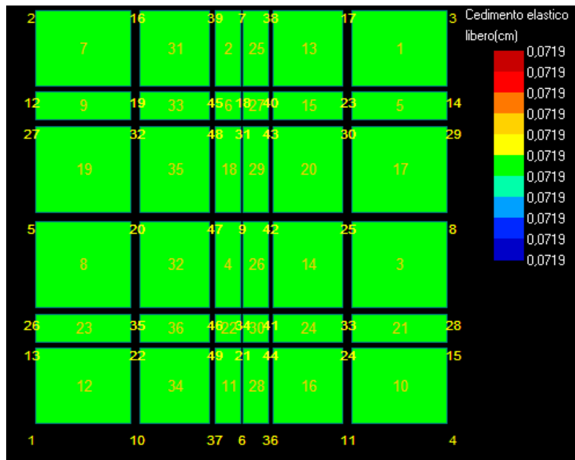
Figura 25: Cedimento - Stratigrafia 3.
