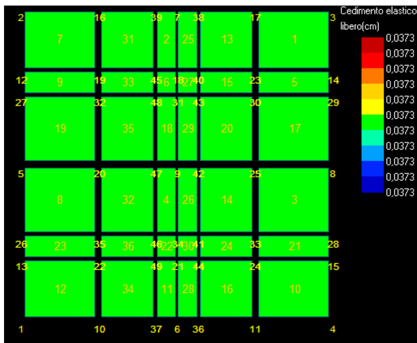
Figura 23: Cedimento - Stratigrafia 1.
