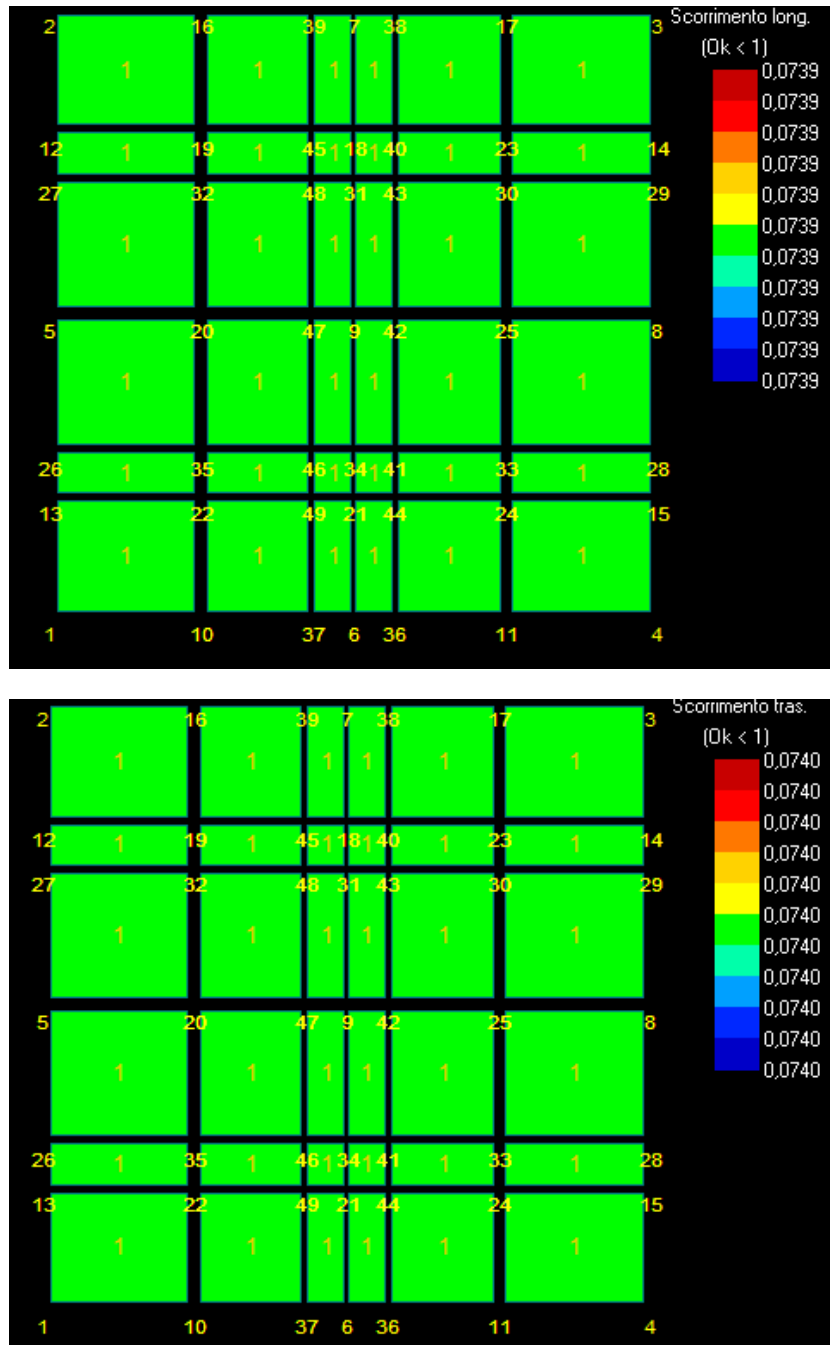
Figura 22: Scorrimento - Stratigrafia 4.
