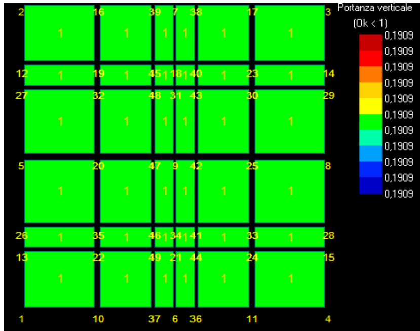
Figura 16: Portata – carico limite - Stratigrafia 2.
