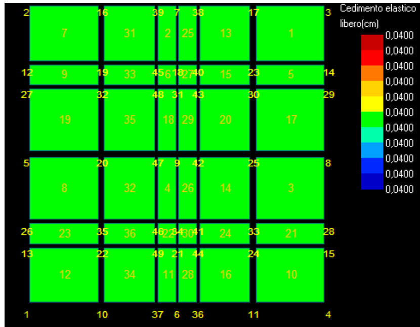
Figura 26: Cedimento - Stratigrafia 4.
