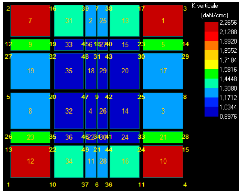
Figura 10: Costante di Winkler – stratigrafia 2.
