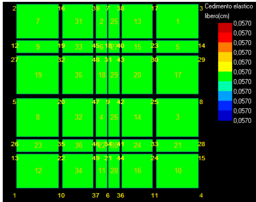
Figura 24: Cedimento - Stratigrafia 2.
