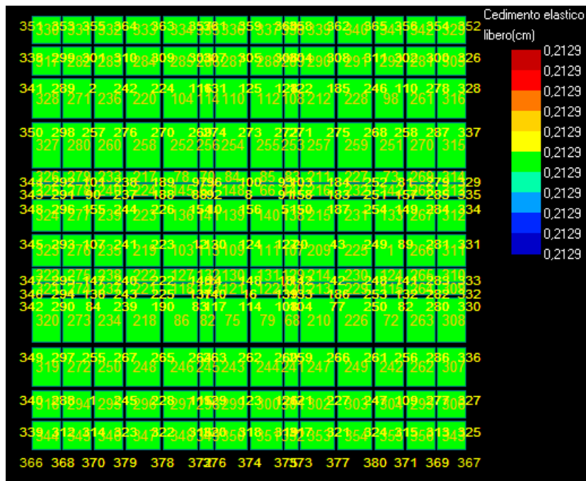
Figura 24: Cedimento - Stratigrafia 2.
