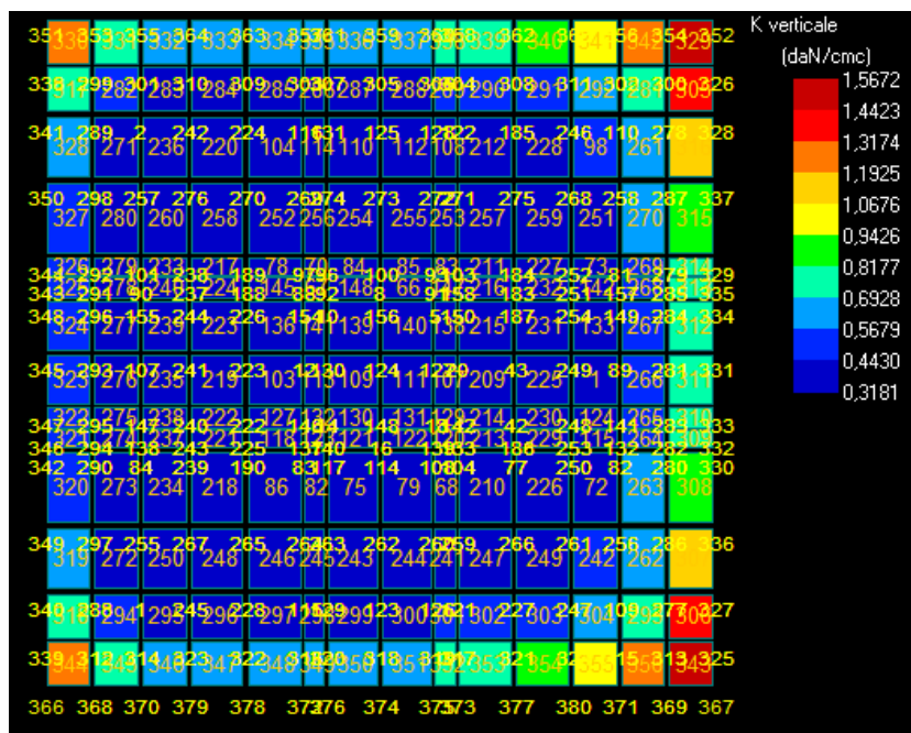
Figura 11: Costante di Winkler – stratigrafia 3.
