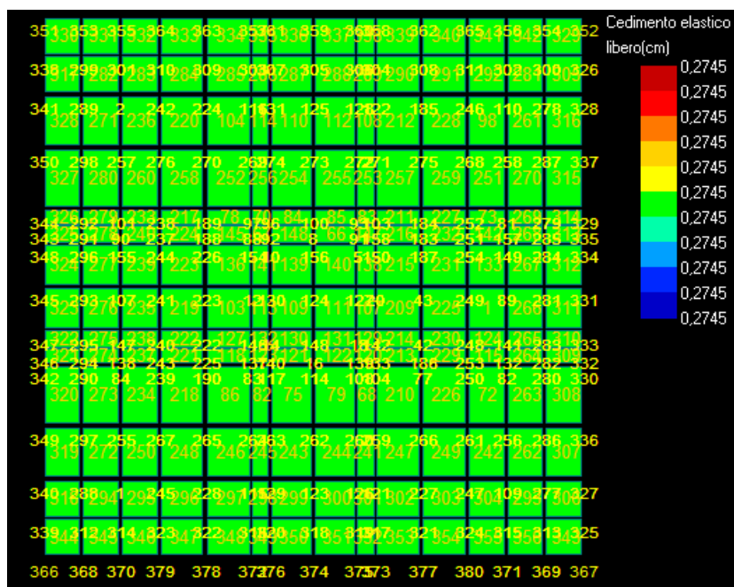
Figura 25: Cedimento - Stratigrafia 3.
