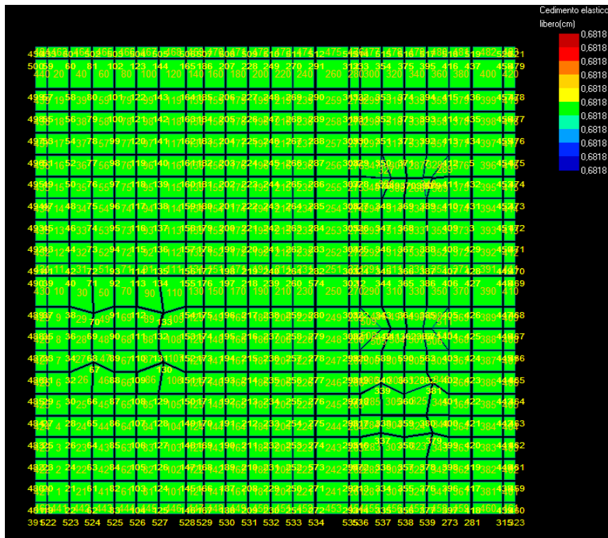
Figura 23: Cedimento - Stratigrafia 1.
