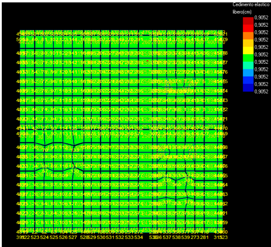
Figura 25: Cedimento - Stratigrafia 3.
