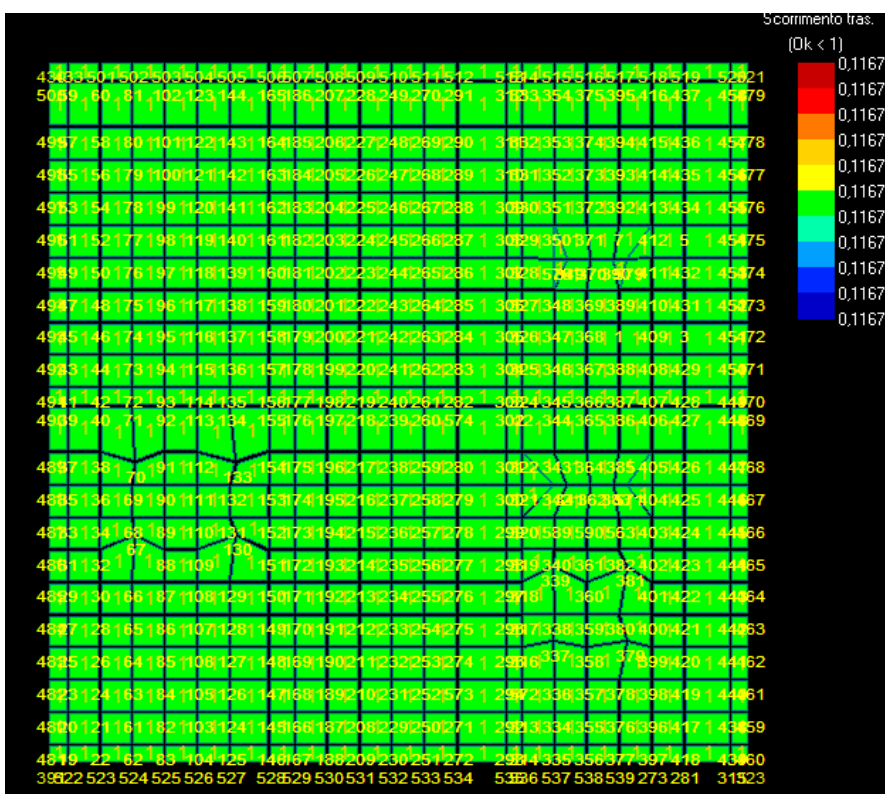
Figura 22: Scorrimento - Stratigrafia 4.
