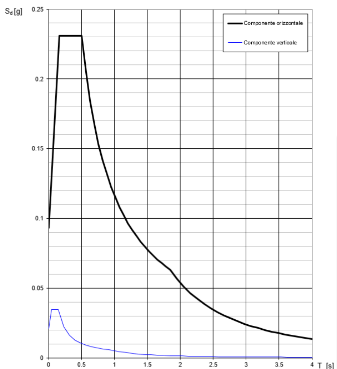
Figura 15: Parametri spettro di risposta SLD.
