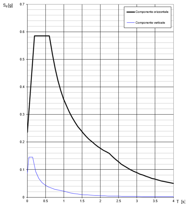
Figura 14: Parametri spettro di risposta SLV.
