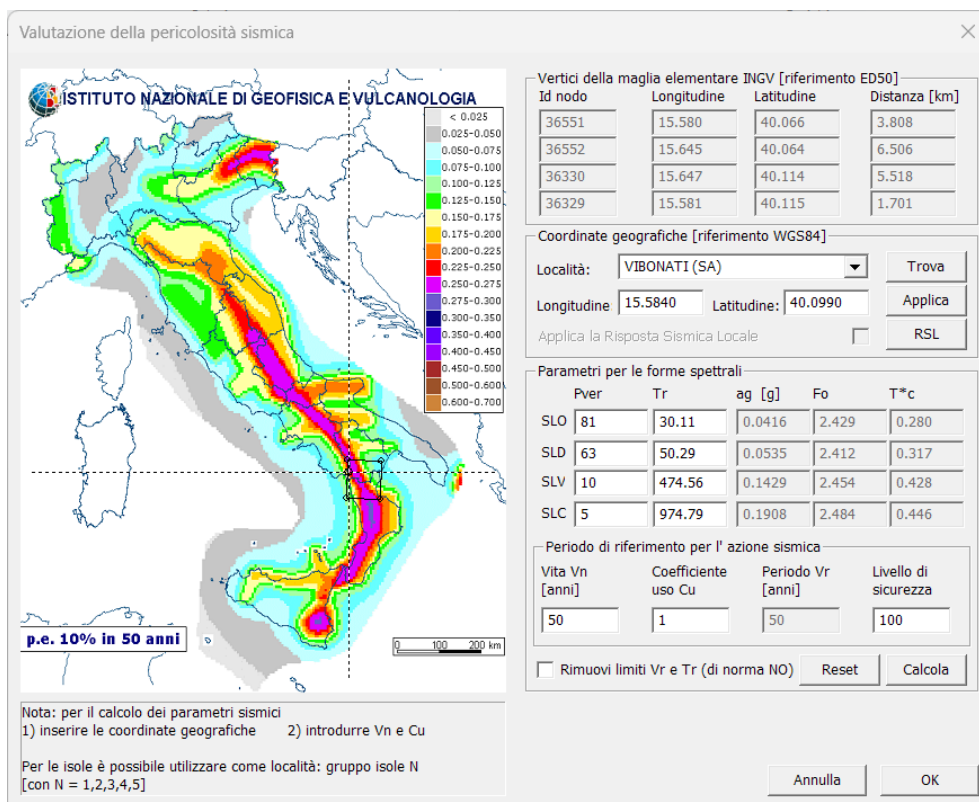
Figura 5: Valutazione della pericolosità sismica.
