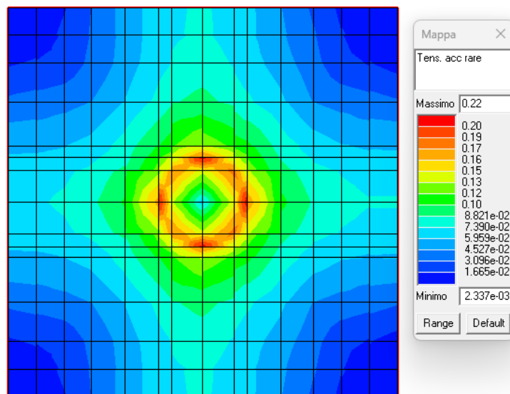
Figura 25: Verifica tensioni rare nell'acciaio.
