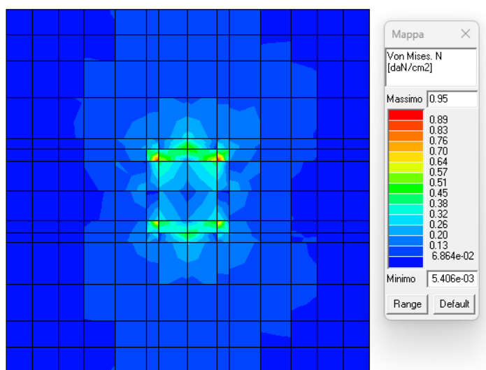
Figura 17: Tensioni di membrana (N) tramite formulazione di Von Mises.
