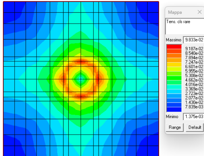
Figura 24: Verifica tensioni rare nel cls.
