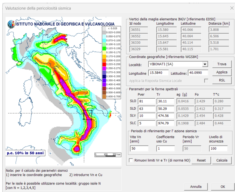
Figura 6: Valutazione della pericolosità sismica.
