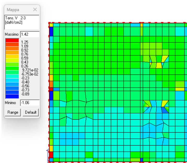
Figura 21: Tensioni di taglio 2-3 in daN/cm 2 .
