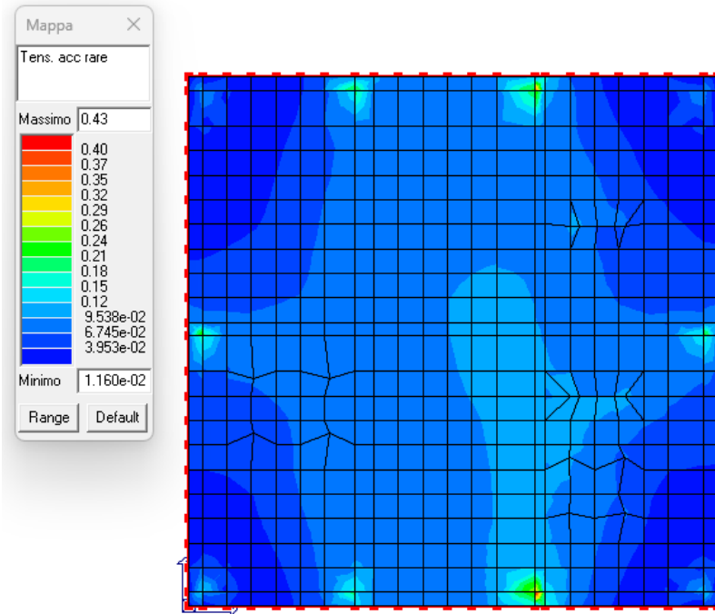
Figura 26: Verifica tensioni rare nell'acciaio.
