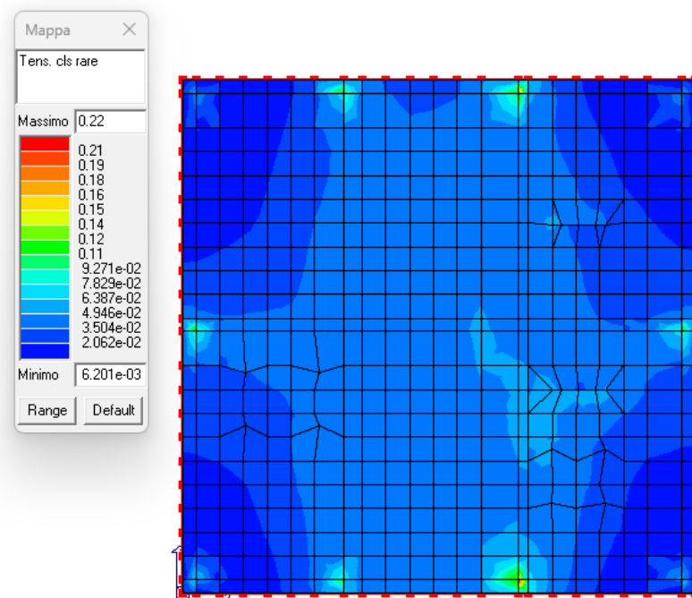
Figura 25: Verifica tensioni rare nel cls.
