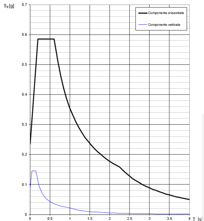
Figura 15: Parametri spettro di risposta SLV.
