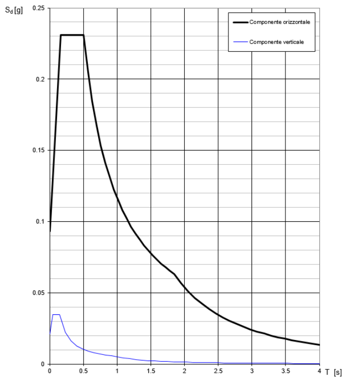
Figura 16: Parametri spettro di risposta SLD.
