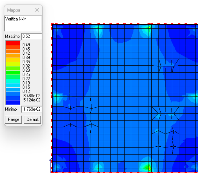
Figura 22: Verifica N/M
