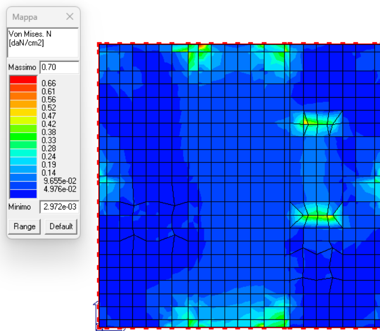
Figura 18: Tensioni di membrana (N) tramite formulazione di Von Mises.
