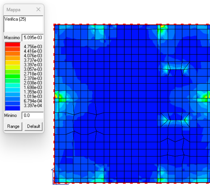
Figura 23: Verifica 25
