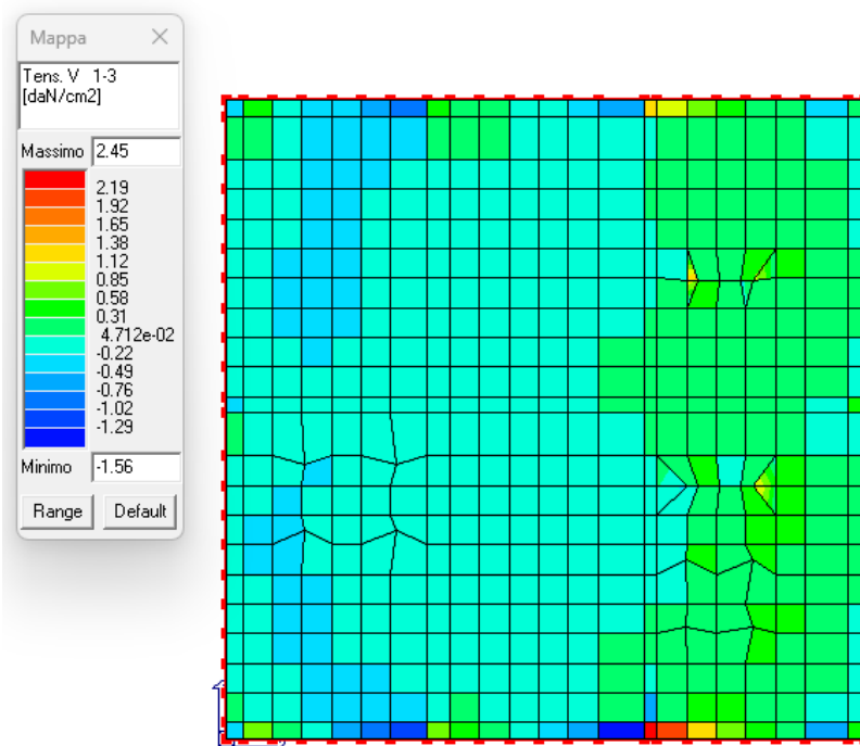
Figura 20: Tensioni di taglio 1-3 in daN/cm 2 .
