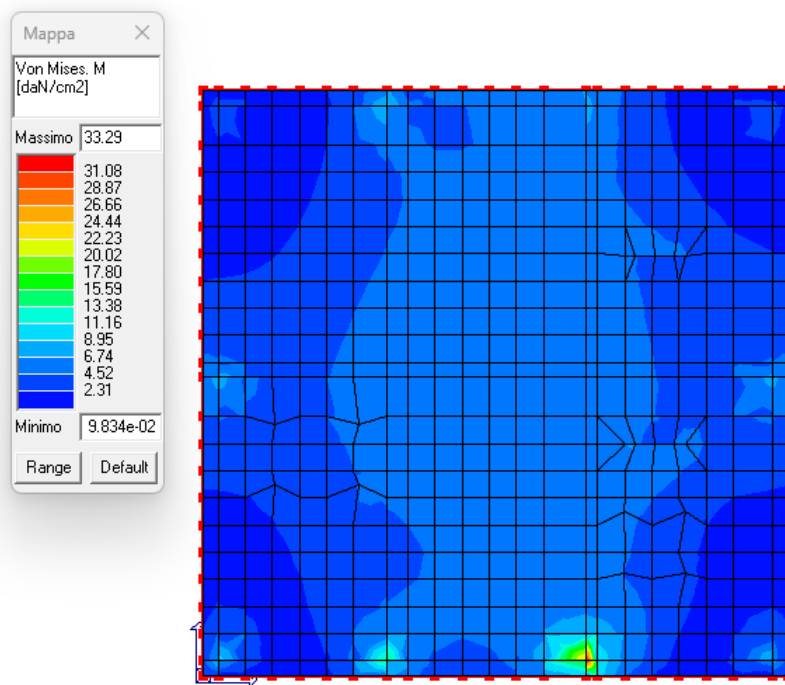
Figura 19: Tensioni di flessione (M) tramite formulazione di Von Mises.
