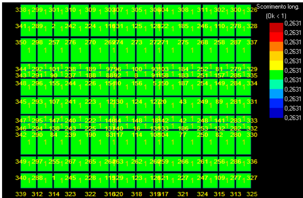
Figura 13: Scorrimento - Stratigrafia 1.
