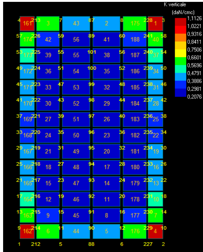
Figura 7: Costante di Winkler – stratigrafia 1.
